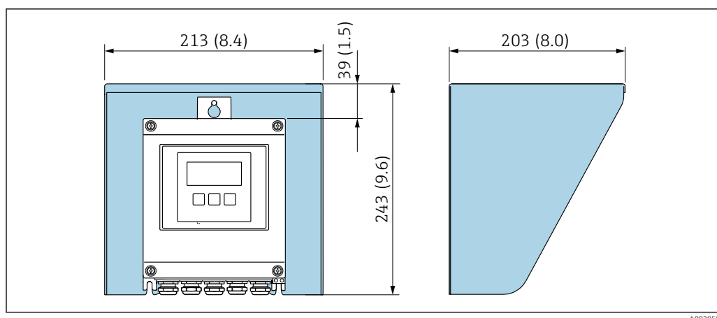
19 Tettuccio di protezione dalle intemperie per Proline 500 – digital; unità ingegneristica mm (in)
