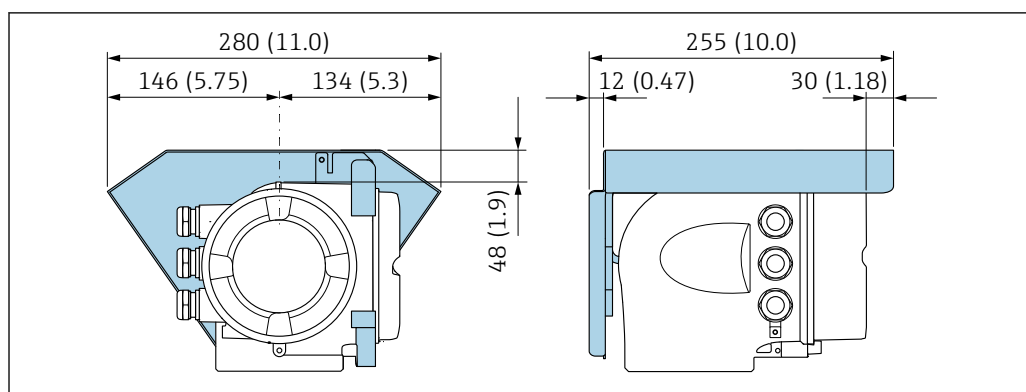
20 Tettuccio di protezione dalle intemperie per Proline 500 – unità ingegneristica mm (in)
