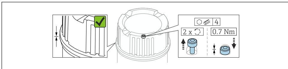
18 Fedél rögzítőcsavarral
