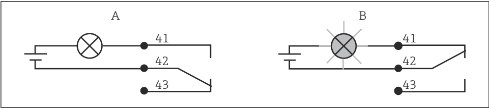
12 Aanbevolen fail-safe schakeling voor het alarmcontact
