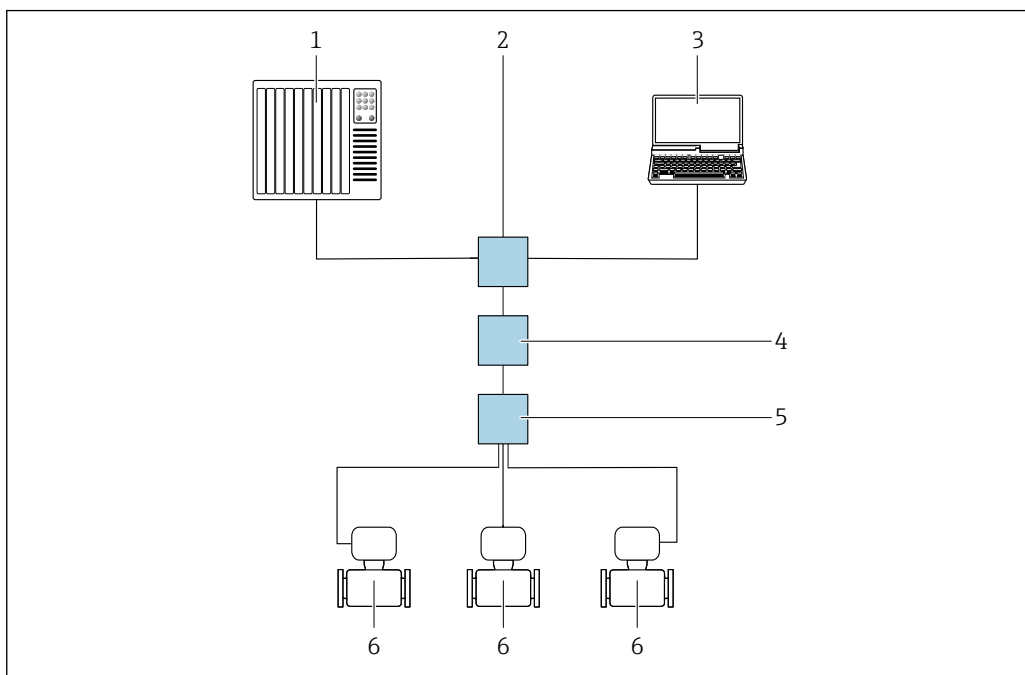
图 33 通过 APL 网络进行远程操作
