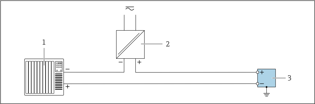
25 接线实例：脉冲输出/频率输出/开关量输出（无源）
