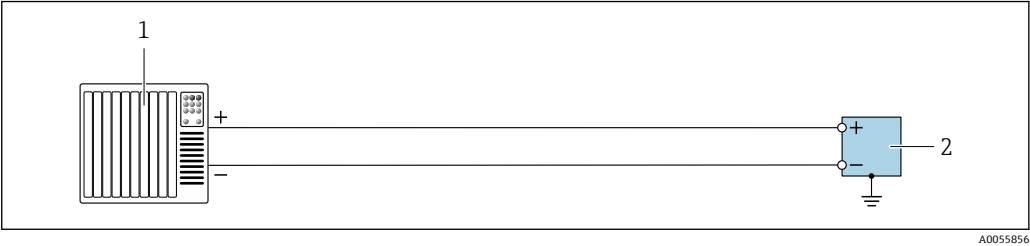
24 接线实例：脉冲输出/频率输出/开关量输出（有源）
