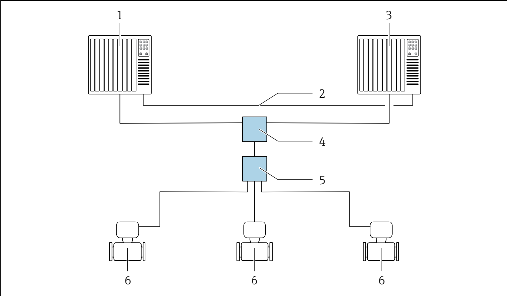
图 36 S2 系统冗余布局实例：星形拓扑结构
