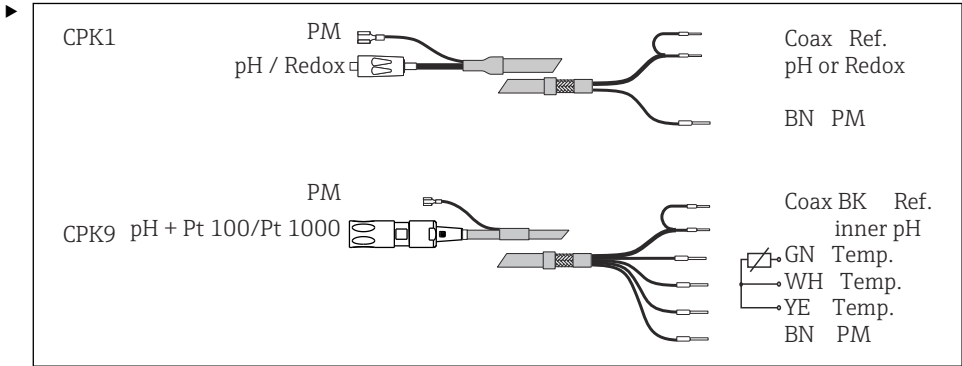
11 Koble til en pH/ORP-sensor med CPK1- eller CPK9-kabler
