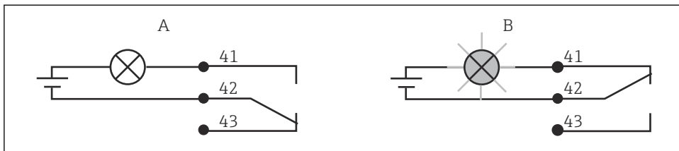
14 Anbefalt feilsikker omkobling for alarmkontakten
