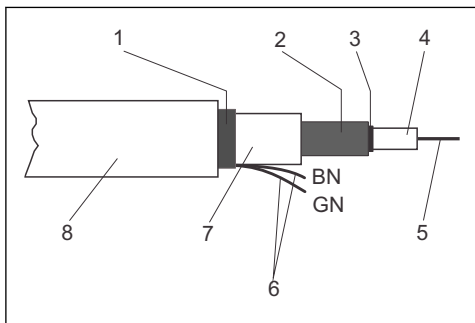
12 Struktur på kabel CMK
