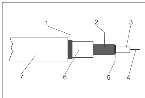
13 Struktur på kabel CYK71
