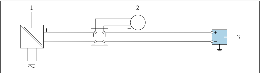
图 10 接线实例：4 ... 20 mA 电流输入
