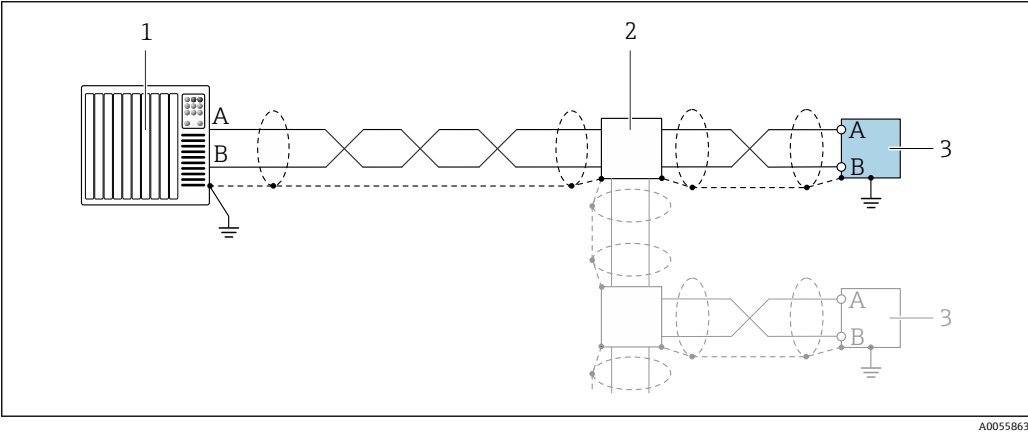
15 接线实例：Modbus RS485
