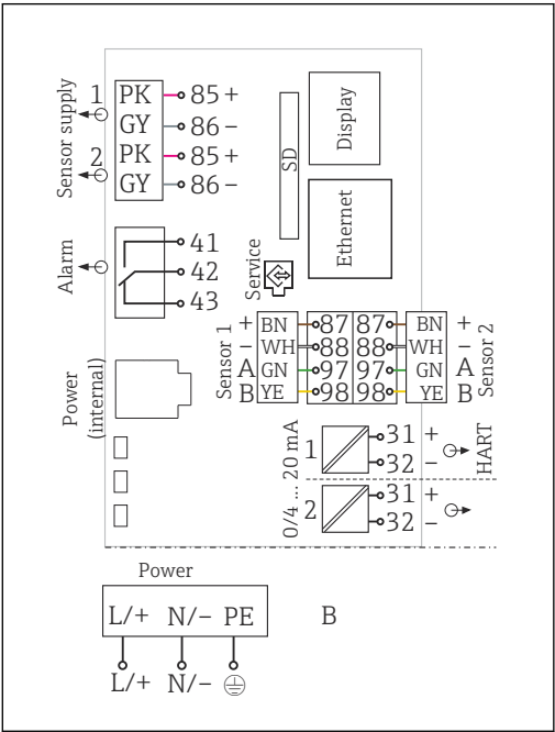
图 15 BASE2-E 模块和外接供电单元 (B) 的完整接线图
