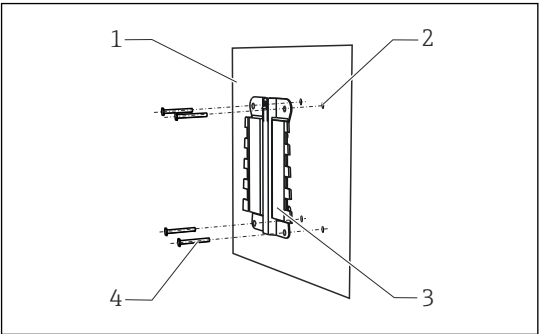
图 30 墙装示意图
