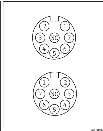
图 23 M12 连接头；上图：插座；下图：插头（均为俯视图）
