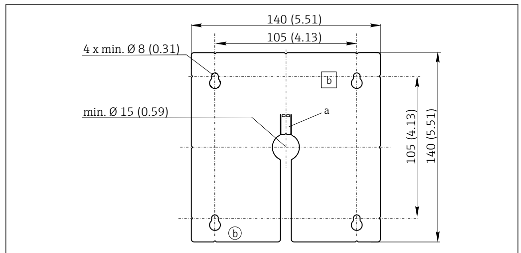
33 外接显示单元的安裝板的外形尺寸示意图; 单位: mm (in)
