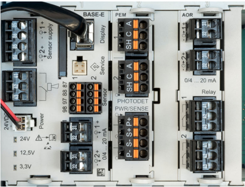
7 CM44P: 示意图
