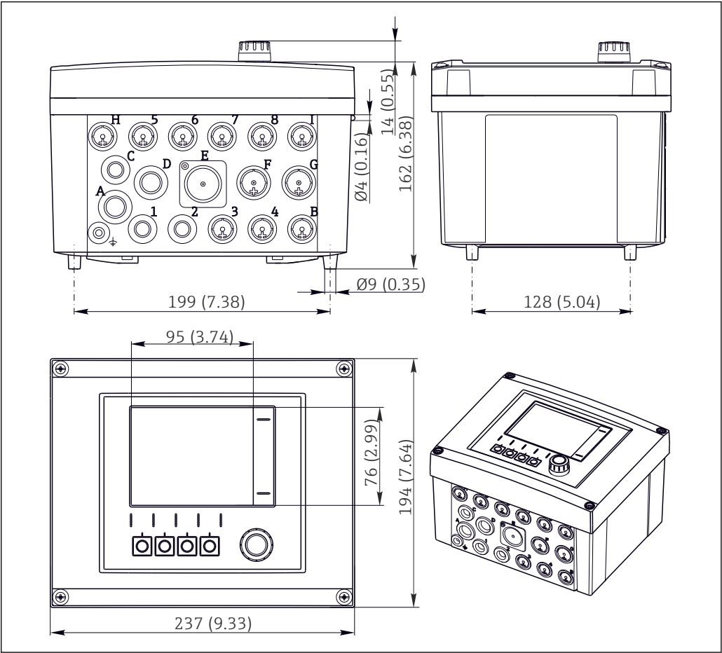
34 现场型外壳的外形尺寸，单位：mm (in)
