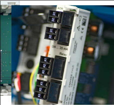
8 扩展模块示意图
