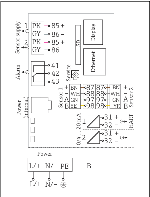
图 13 BASE2-E 模块和扩展供电单元 (B) 的完整接线图
