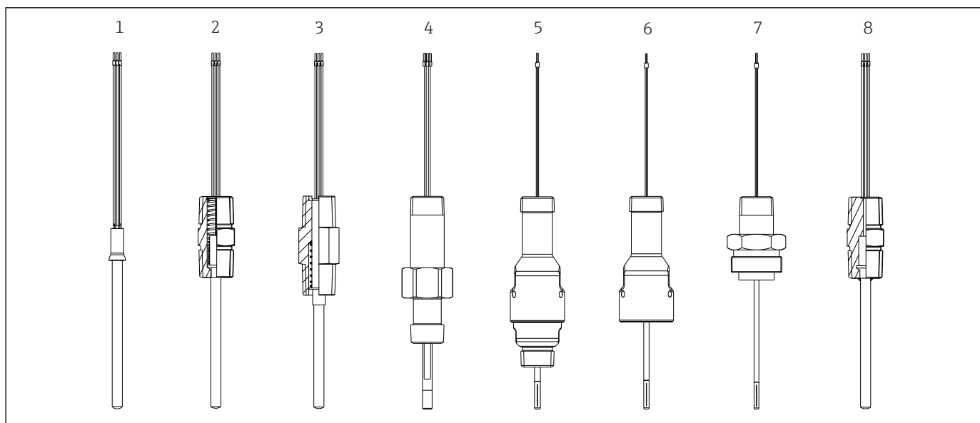
1 Aperçu de la construction de l'insert de mesure iTHERM TS212 pour toutes les options de tube prolongateur
