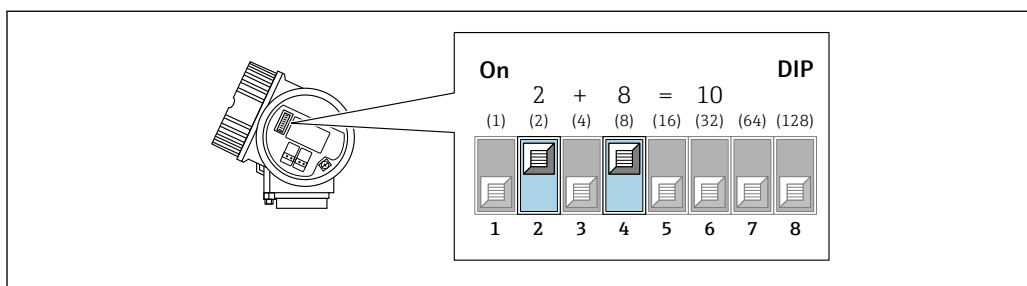
10 Microinterruttore indirizzi nel vano connessioni; esempio di come configurare l'indirizzo del dispositivo 10.
