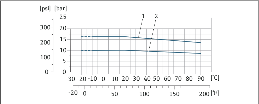
图 25 过程连接材质：不锈钢 (-20 °C (-4 °F)) ； 碳钢 (-10 °C (14 °F))
