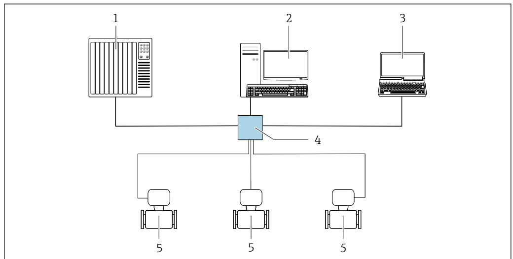
图 43 通过 Modbus TCP + Ethernet 进行远程操作 - 100 Mbit/s: 星形拓扑结构
