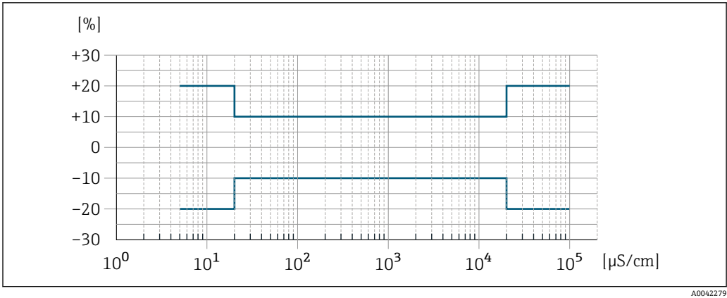
15 测量误差 (标准)
