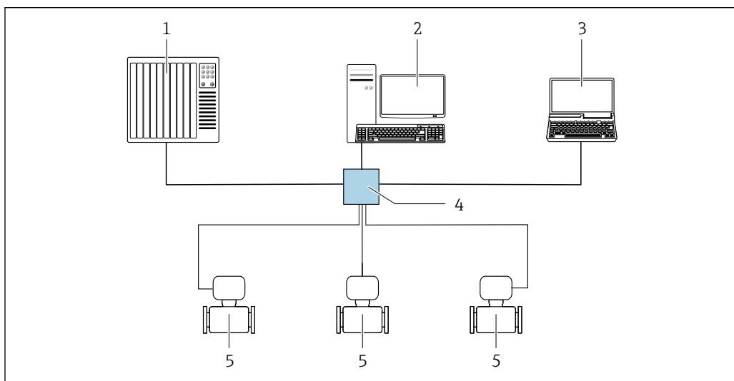
图 44 通过 EtherNet/IP 网络进行远程操作：星形拓扑结构
