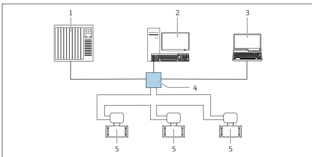
图 45 通过 EtherNet/IP 网络进行远程操作：环形拓扑结构
