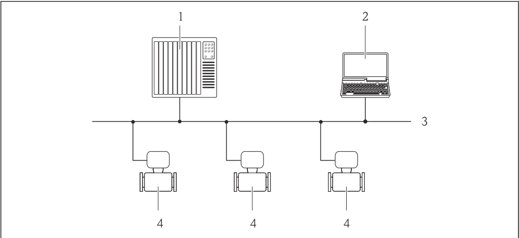
39 通过 PROFIBUS DP 网络进行远程操作
