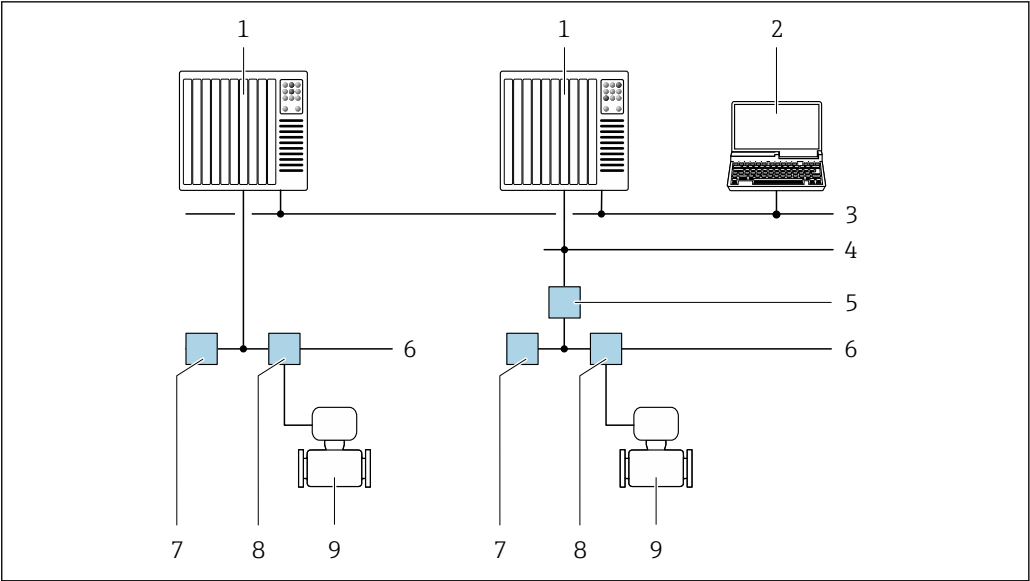
38 通过 FOUNDATION Fieldbus 网络进行远程操作
