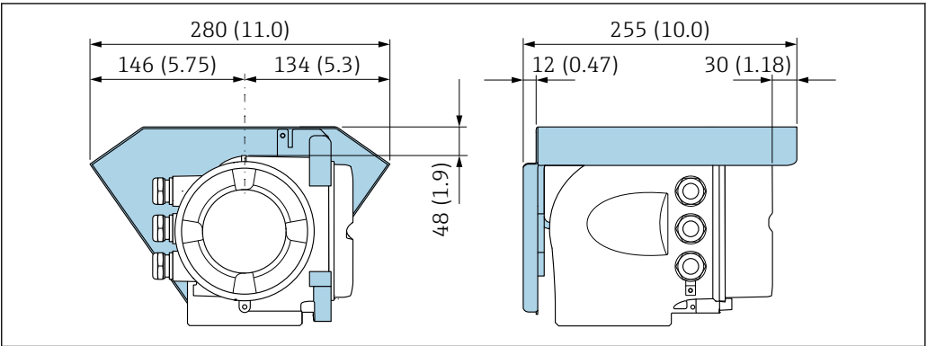
图 17 单位: mm (in)
