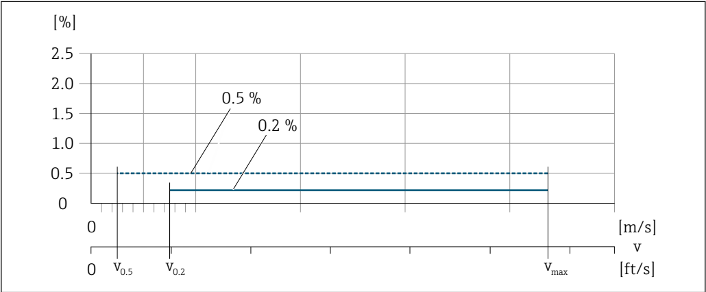
图 14 设计测量精度 (% o.r.)
