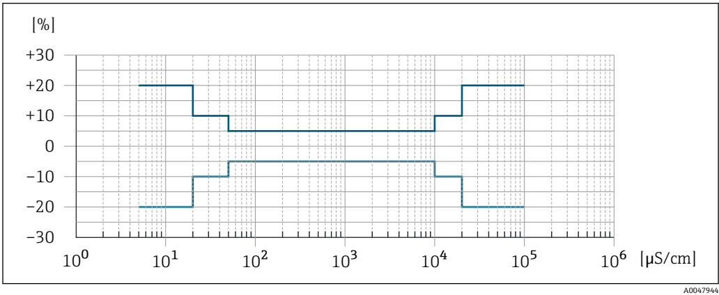
16 测量误差 (可选: 订购选项“电导率测量标定”, 选型代号 CW)
