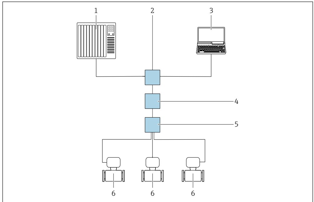
图 42 通过 Modbus TCP + Ethernet-APL 通信进行远程操作（有源信号）
