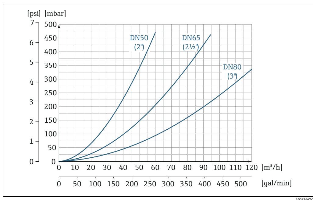
图 26 压损: 适用口径 DN 50...80 (2...3"); 订购选项“设计”, 选型代号 C “固定法兰, 缩径测量管, 无前后直管段长度要求”
