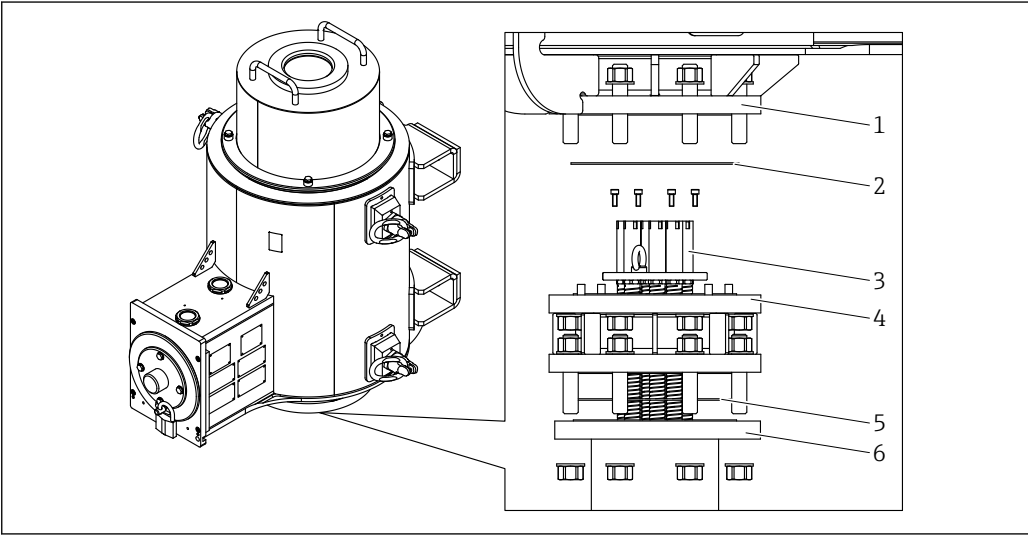
图 14 波纹管安装转接头
