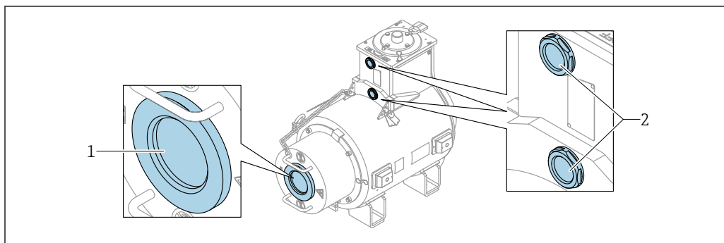
图 34 观察窗位置
