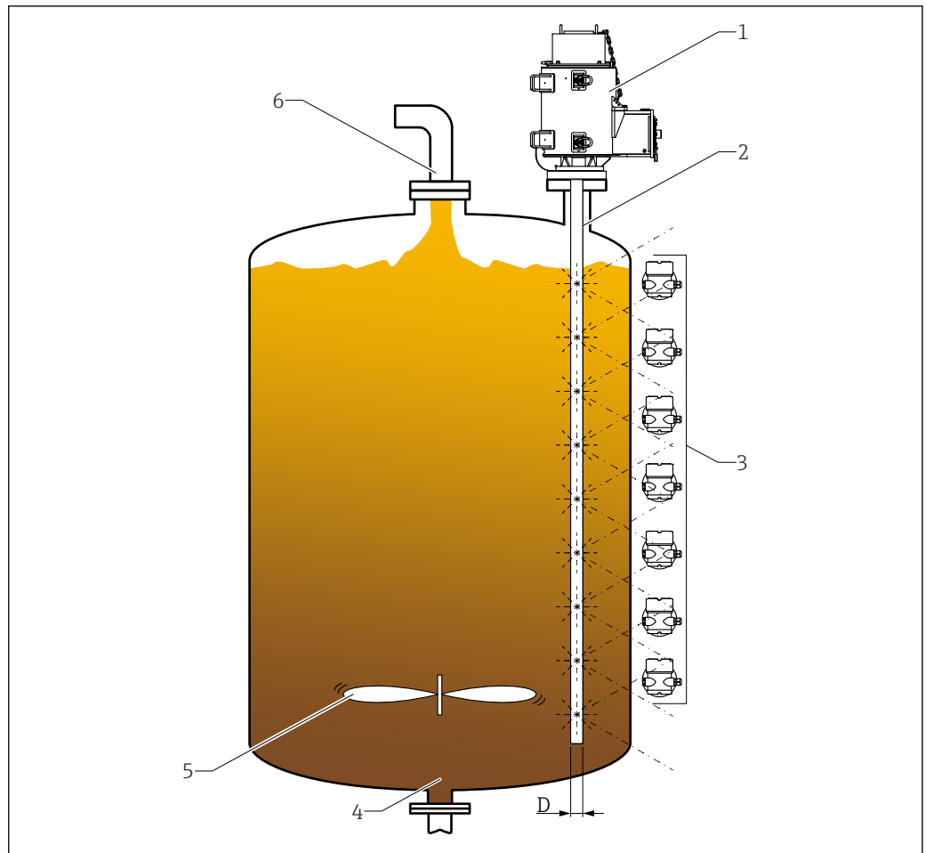
图 29 密度测量（多点）
