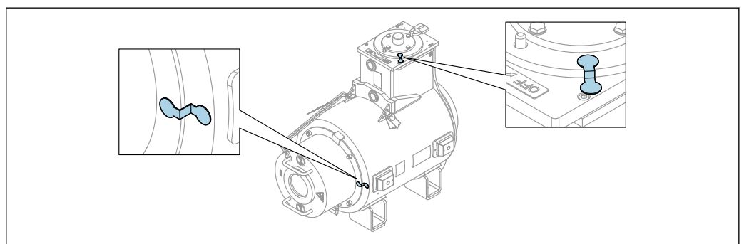
43 源盒上的安全密封件
