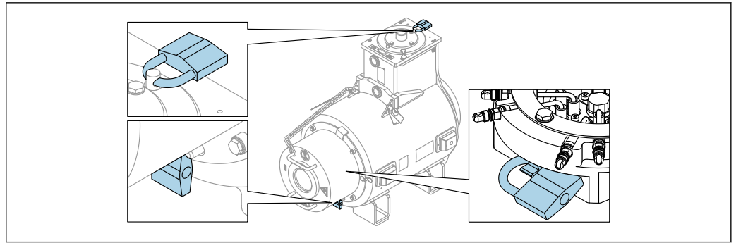
41 锁具
