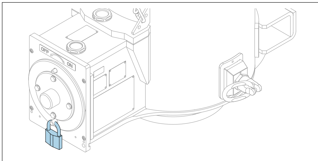
图 11 防扭转装置锁具
