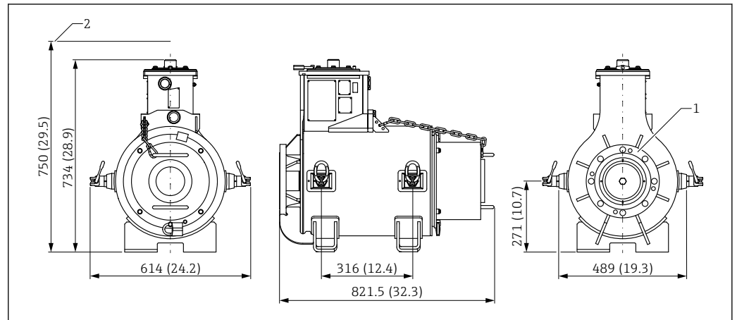
图 23 外形尺寸。测量单位 mm (in)
