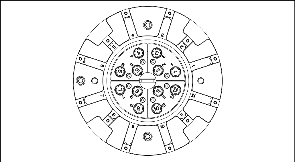
图 31 源匣装载示意图 (12 位)
