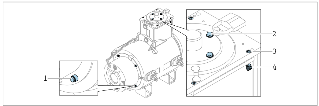
图 35 外壳上的螺纹连接
