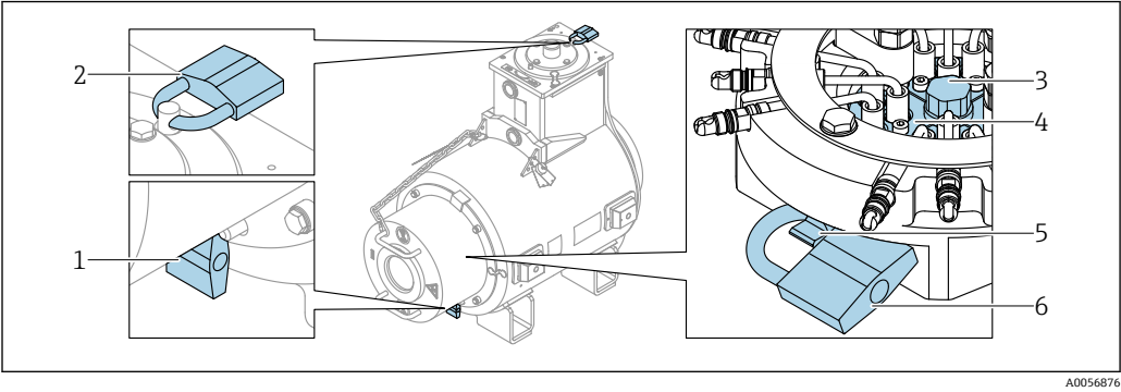
图 37 防盗保护部件
