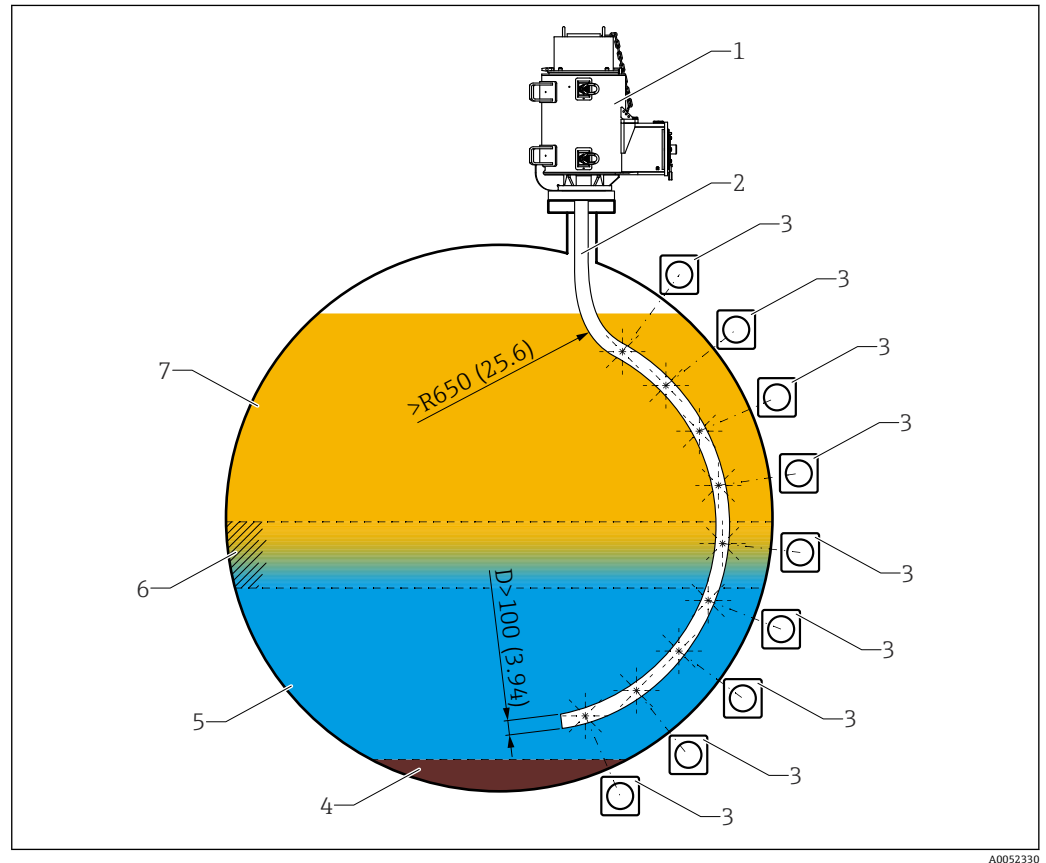
图 27 界面测量
