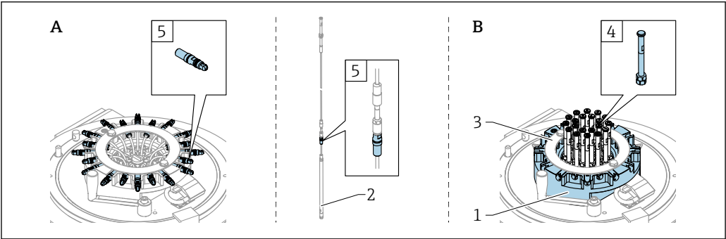
图 38 源匣和放射源座
