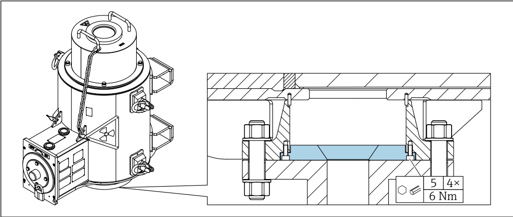
图 13 保护管安装转接头
