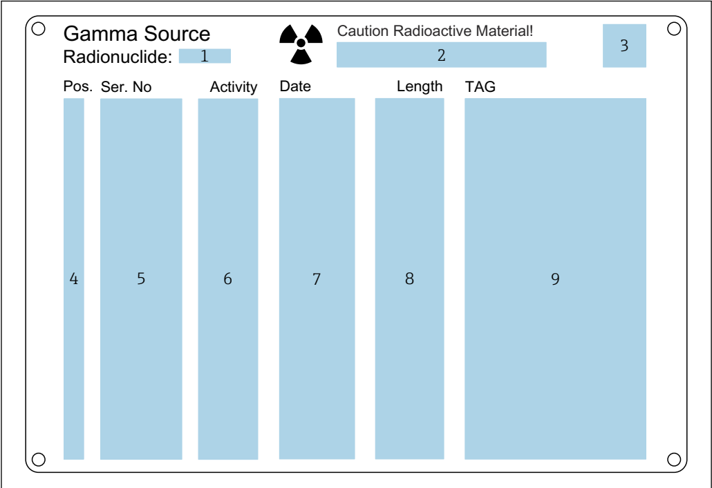
18 放射源铭牌上的标示内容
