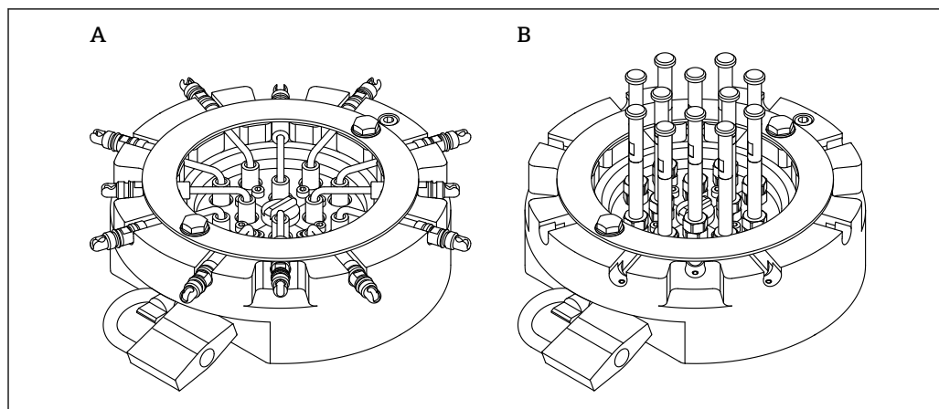
图 5 固定环，带 12 枚可拆卸放射源
