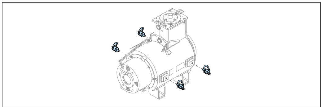
图 44 源盒上的吊点
