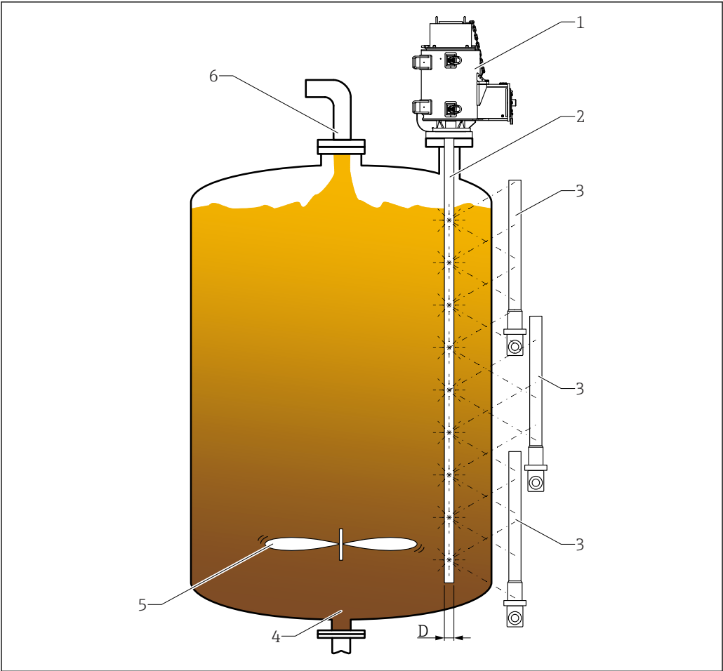
图 28 液位测量
