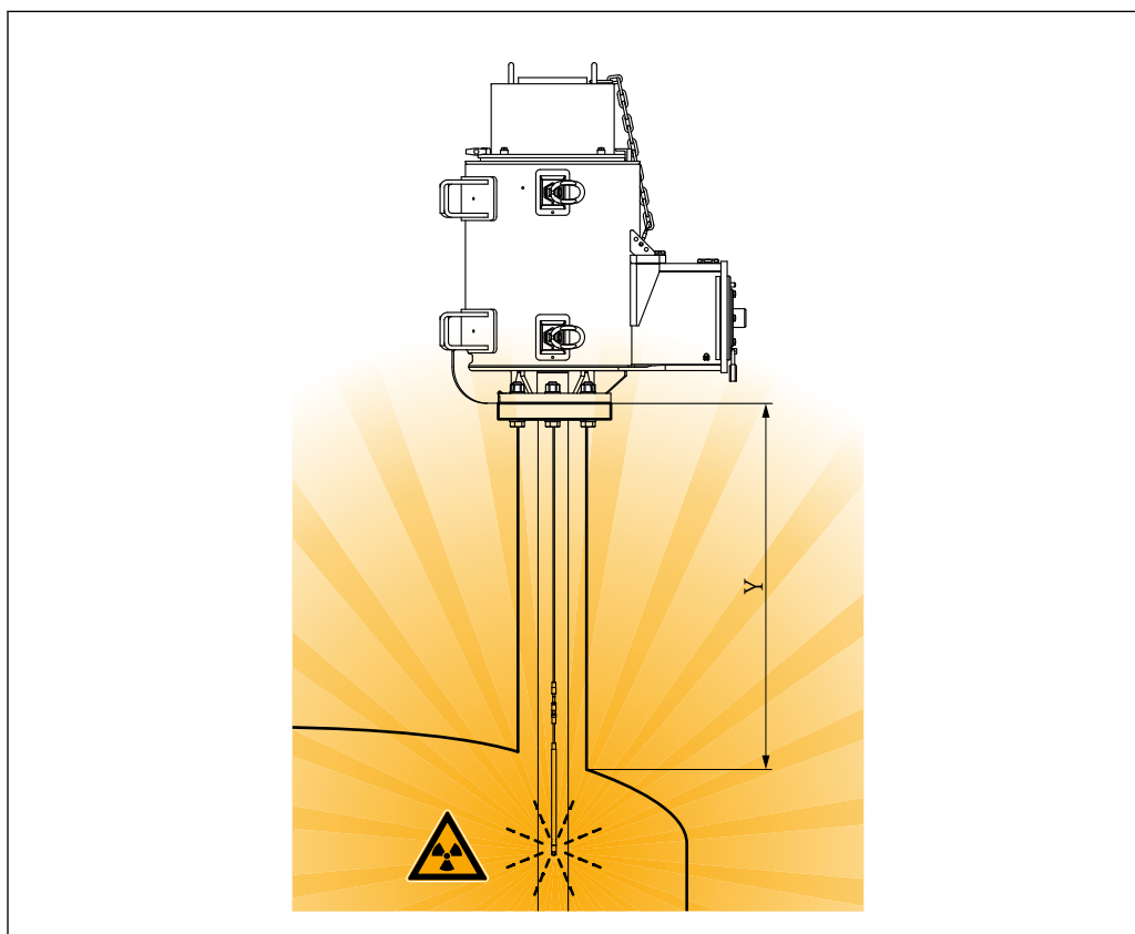
26 安装尺寸
