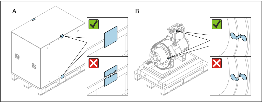
图 15 保护密封件位置
