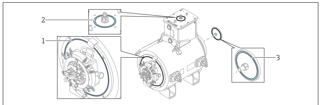
图 36 密封圈
