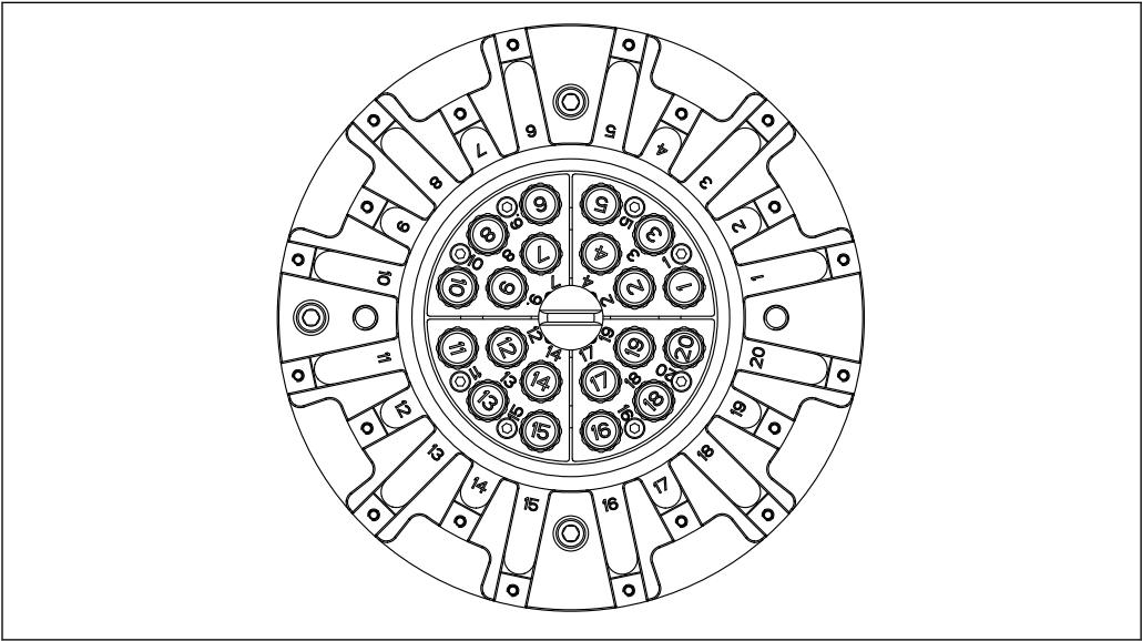
图 30 源匣装载示意图（20 位）
