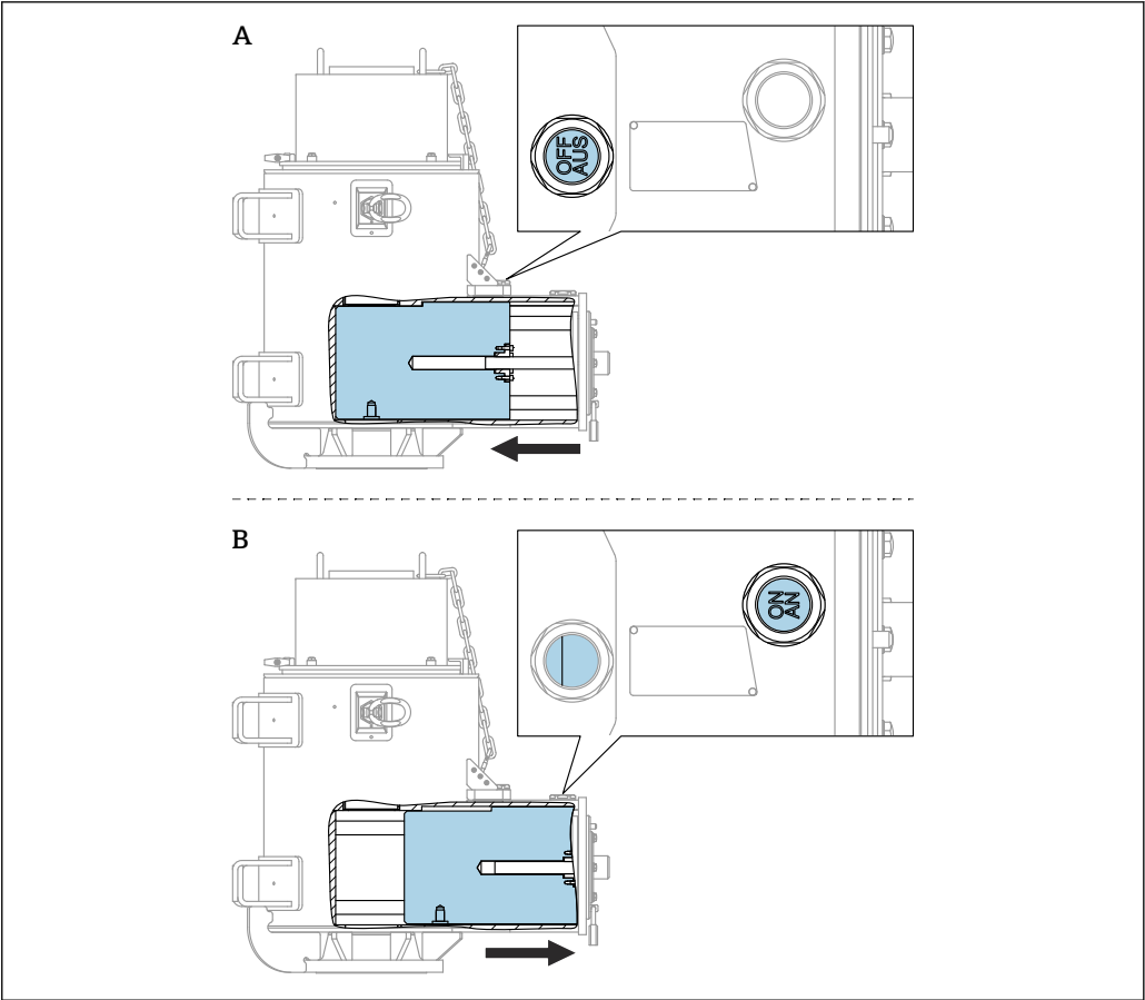
图 3 源闸位置
