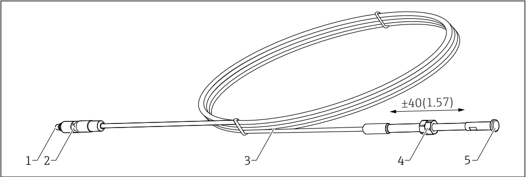
图 9 延长缆
