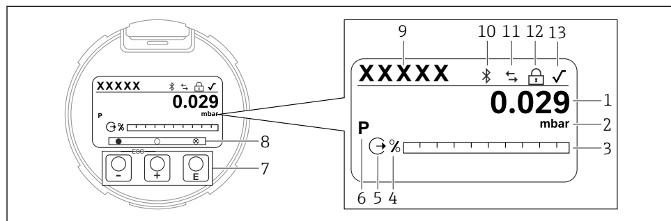
図 4 光学式操作キー付きグラフィックディスプレイ
