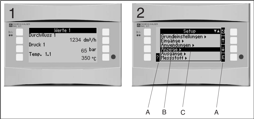
Abb. 16: Anzeigedarstellung des Energierechners
