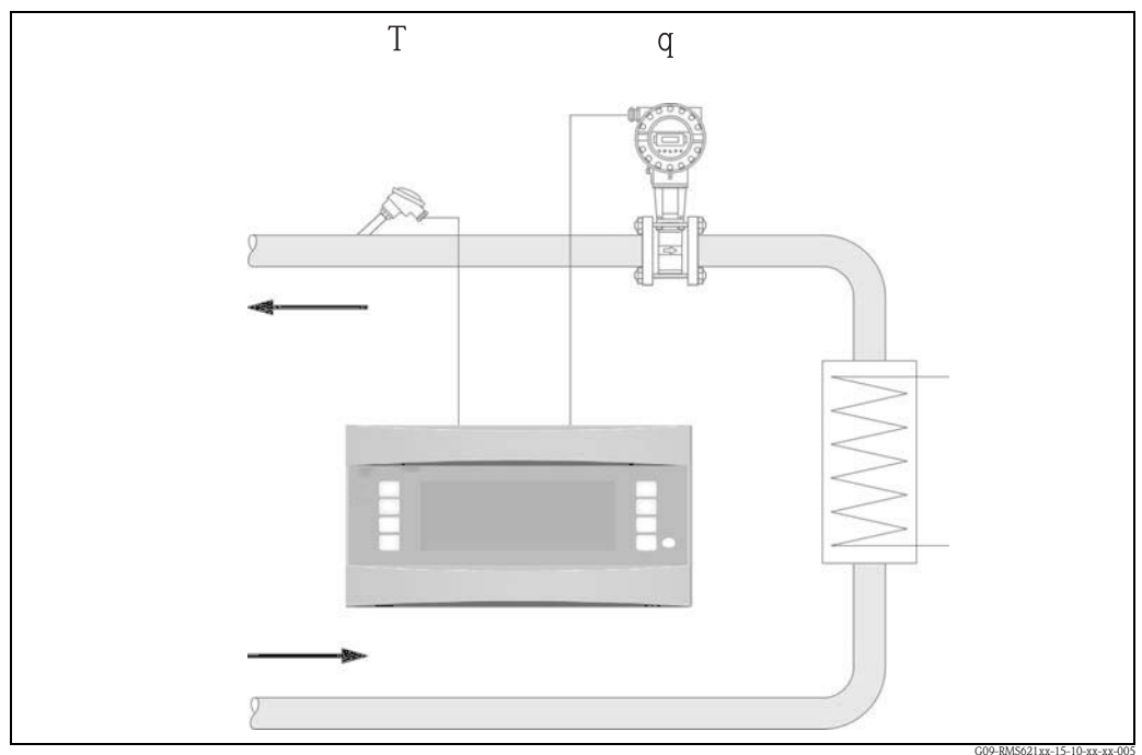
Abb. 28: Applikation Wasser/Wärmemenge
