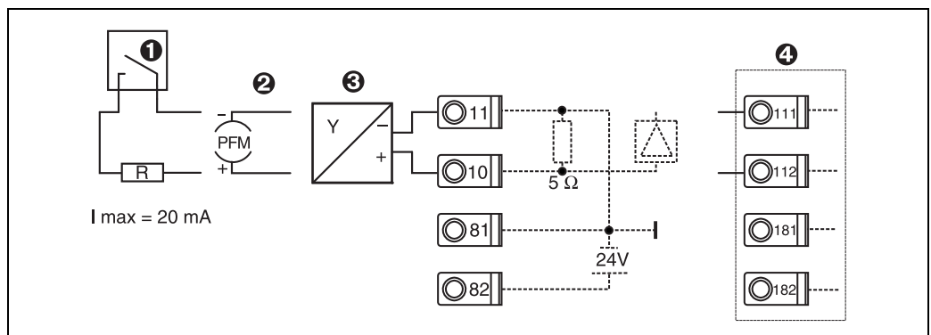
Abb. 7: Anschluss eines aktiven Sensors, z.B. am Eingang 1 (Slot A I).
