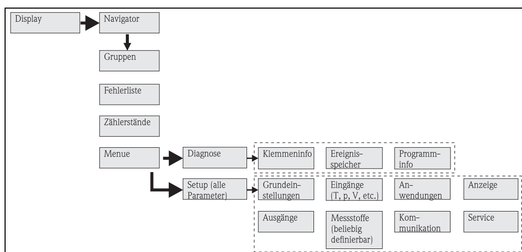
Abb. 21: Funktionsmatrix (Auszug) für die Vor-Ort-Parametrierung des Energiemanagers. Eine ausführliche Funktionsmatrix ist im Anhang zu finden.
