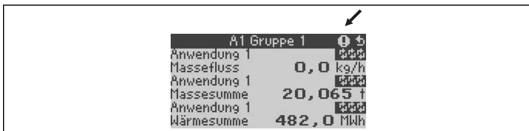
Abb. 19: Fehlermeldung Dampfkondensation (Beispiel)
