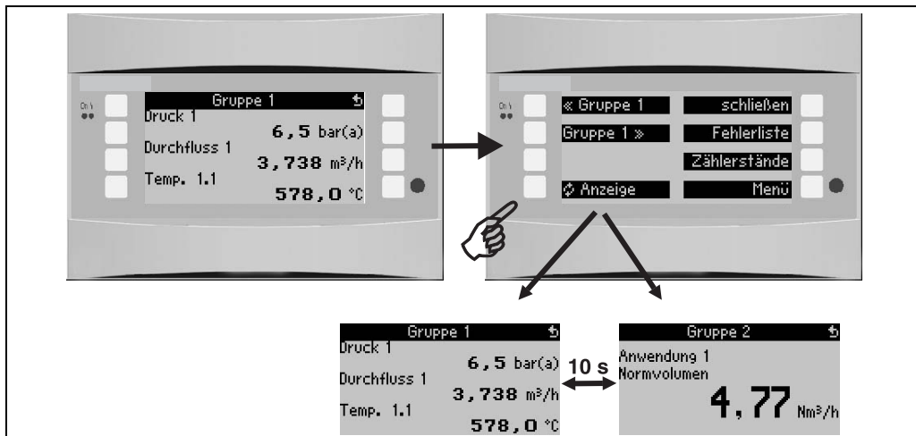
Abb. 23: Automatischer Wechsel verschiedener Anzeigegruppen
