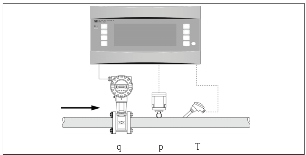
Abb. 34: Applikation Gas Normvolumen/Masse/Heizwert
