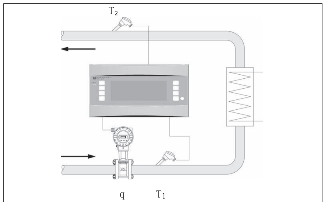
Abb. 32: Applikation Flüssigkeit/Wärmedifferenz
