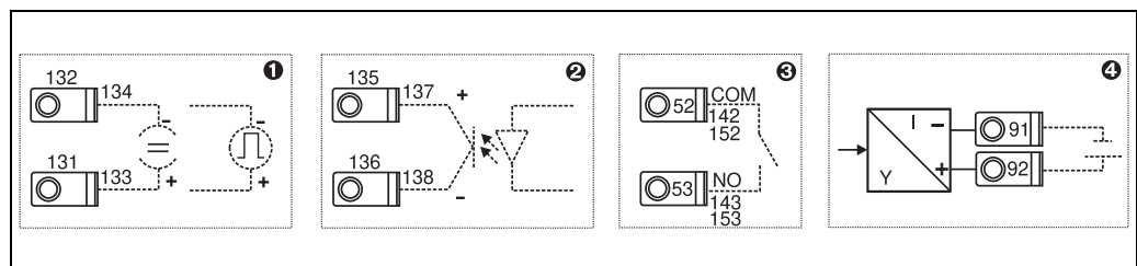
Abb. 10: Anschluss Ausgänge
