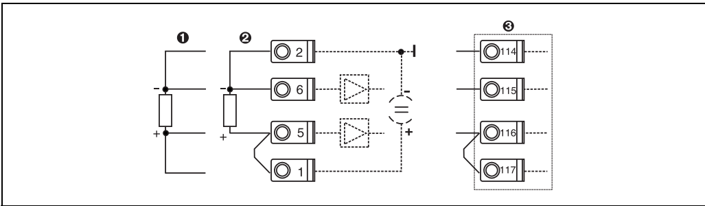
Abb. 9: Anschluss Temperatursensor, z.B. am Eingang 1 (Slot E I)
