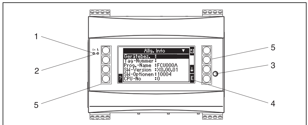
Abb. 15: Anzeige- und Bedienelemente
