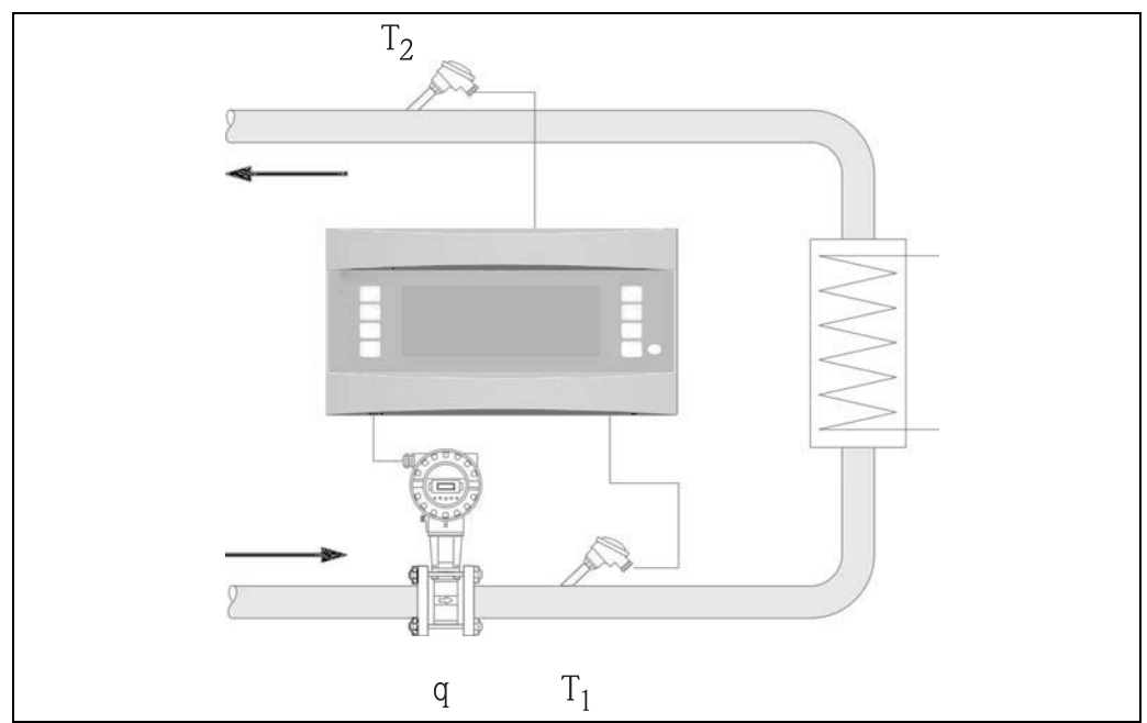
Abb. 29: Applikation Wasser/Wärmedifferenz
