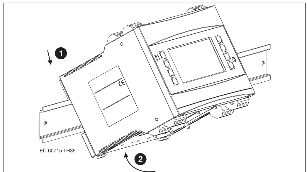
Abb. 3: Gerätemontage auf Hutschiene
