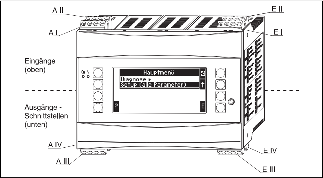
Abb. 5: Slot-Belegung (Grundgerät)
