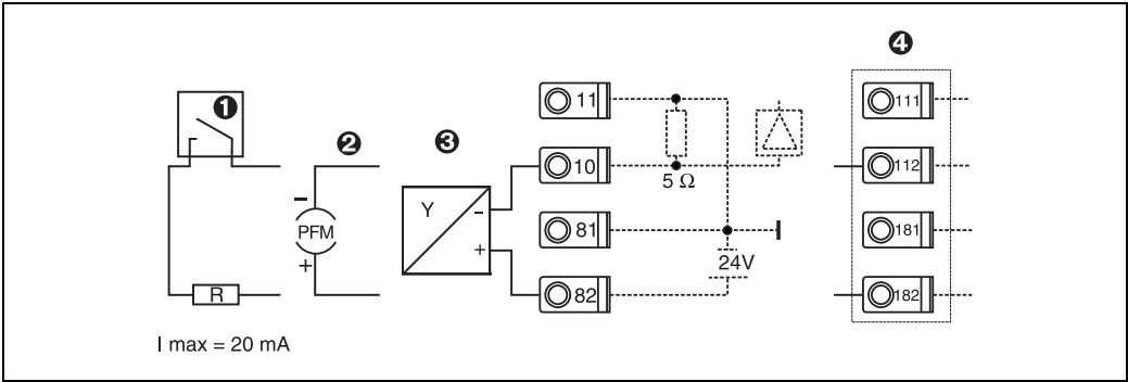
Abb. 8: Anschluss eines passiven Sensors, z.B. am Eingang 1 (Slot A I).
