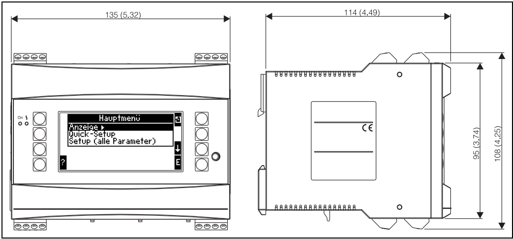
Abb. 25: Gehäuse für Hutschiene nach IEC 60715; Abmessungen in mm (inch)
