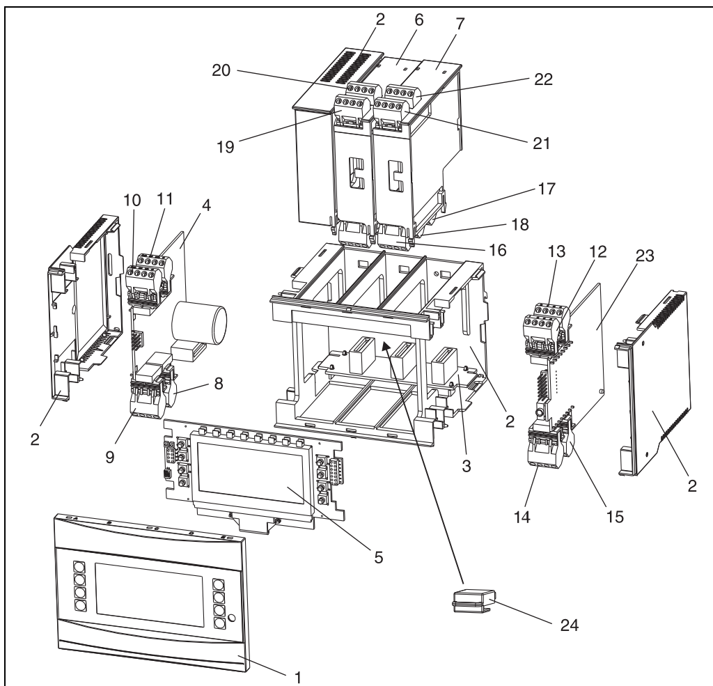
Abb. 24: Ersatzteile des Energiemanagers
