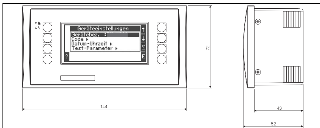
Abb. 26: Bedien-Anzeige-Einheit für Schaltschrankbau (optional oder als Zubehör erhältlich); Abmessungen in mm
