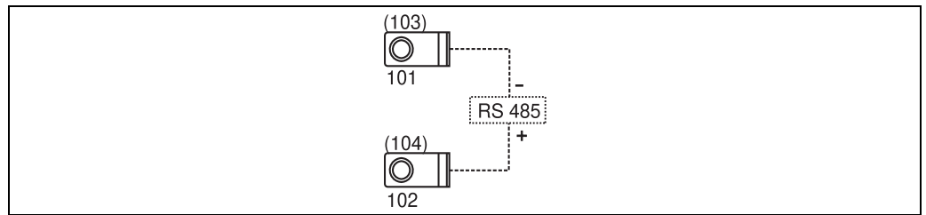
Abb. 11: Anschluss Schnittstellen
