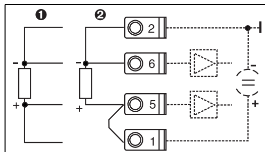
Abb. 1: Anschluss Temperatursensor, z.B. am Eingang 1 (Slot E1)
