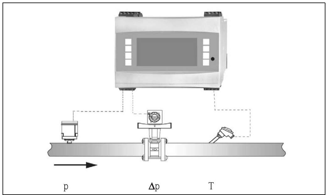
Abb. 30: Applikation Dampfmasse/Wärmemenge
