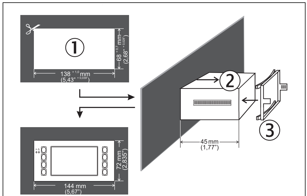
Abb. 13: Schalttafeleinbau
