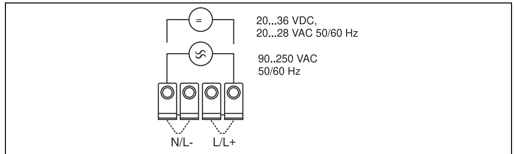
Abb. 6: Anschluss Hilfsenergie
