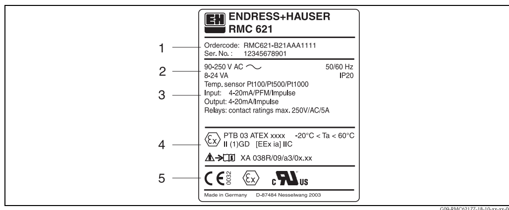
Abb. 2: Typenschild des Energiemanagers (beispielhaft)
