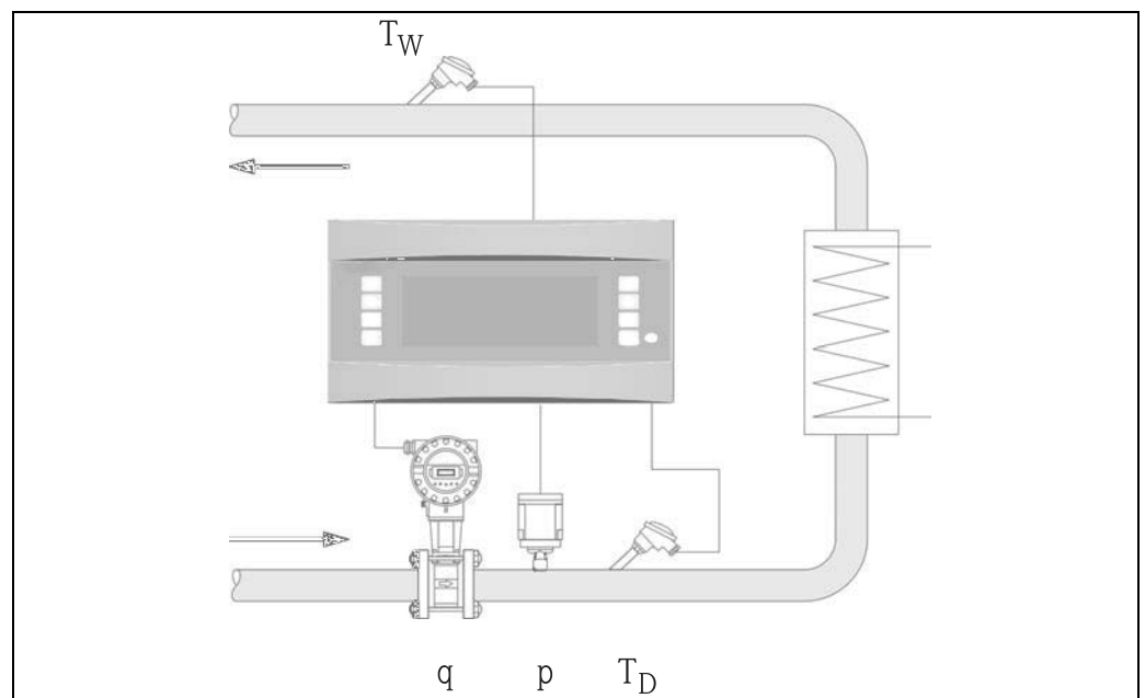
Abb. 31: Applikation Dampf/Wärmedifferenz
