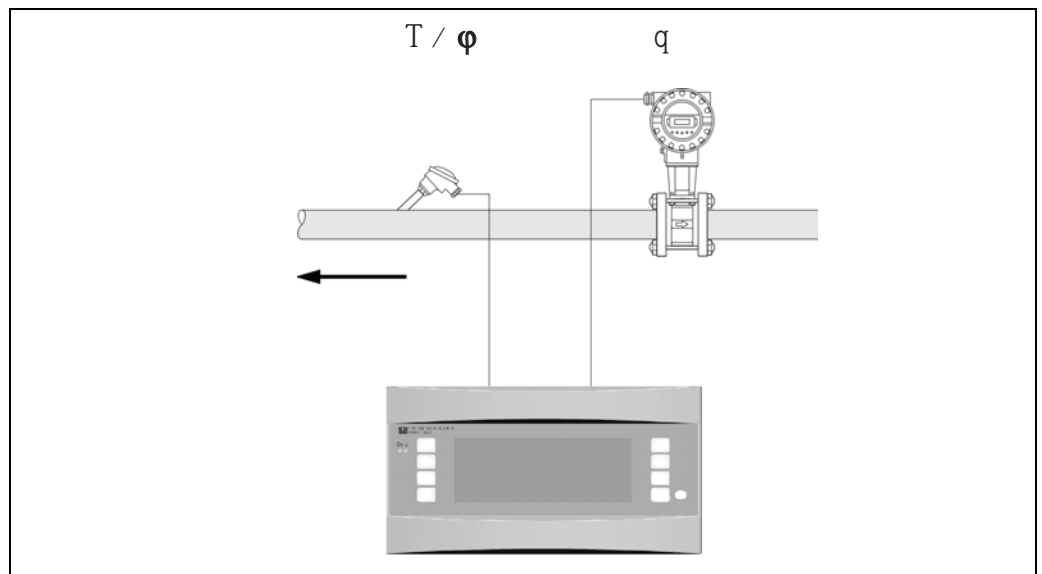
Abb. 33: Applikation Flüssigkeit Normvolumen/Heizwert
