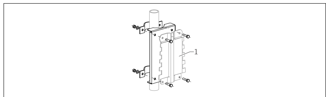
图 66 安装板，适用聚碳酸酯现场型外壳
