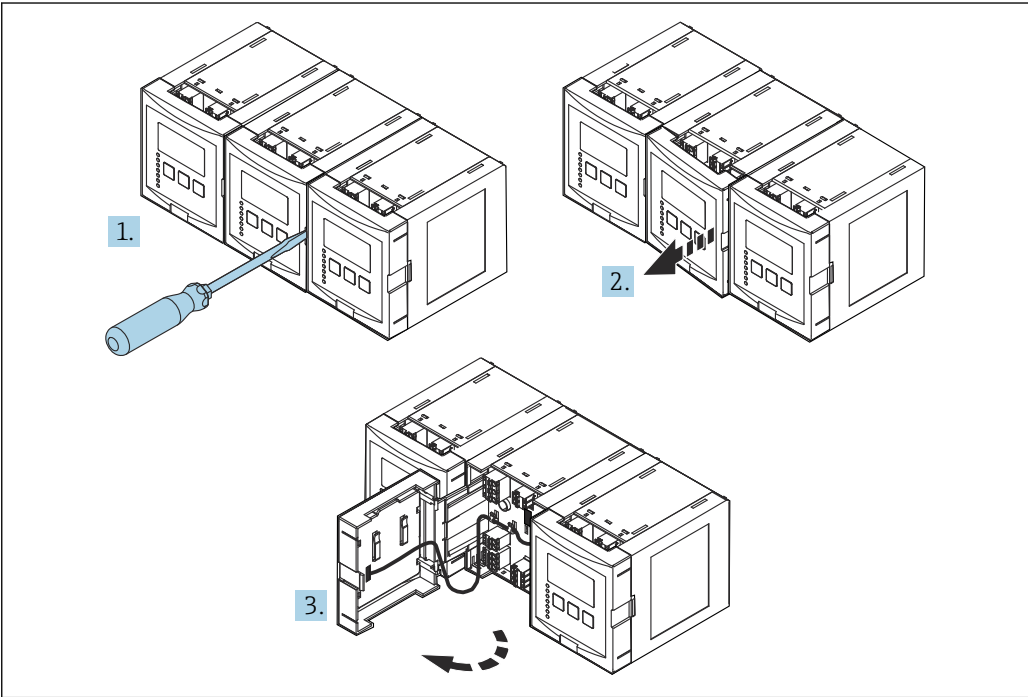
20 接线腔检修口：并排安装多个 DIN 导轨外壳单元
