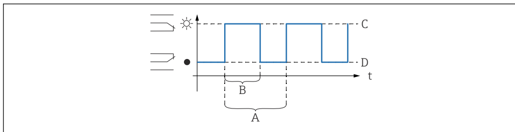
图 58 设置时间脉冲继电器
