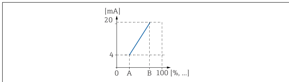
图 62 电流量程比工作原理
