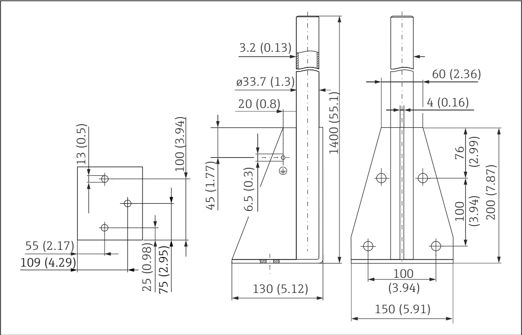
图 68 外形尺寸。测量单位 mm (in)
