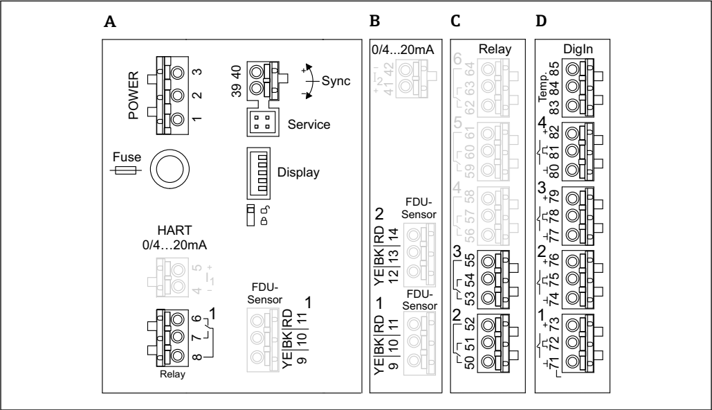
图 21 接线区；显示为灰色的接线端子并非在每个设备型号上提供
