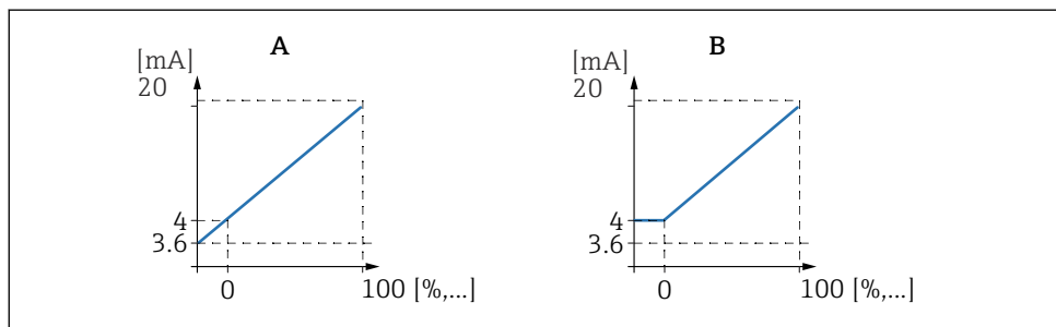
图 61 4mA 阈值 (仅当电流范围= 4 ... 20 mA)
