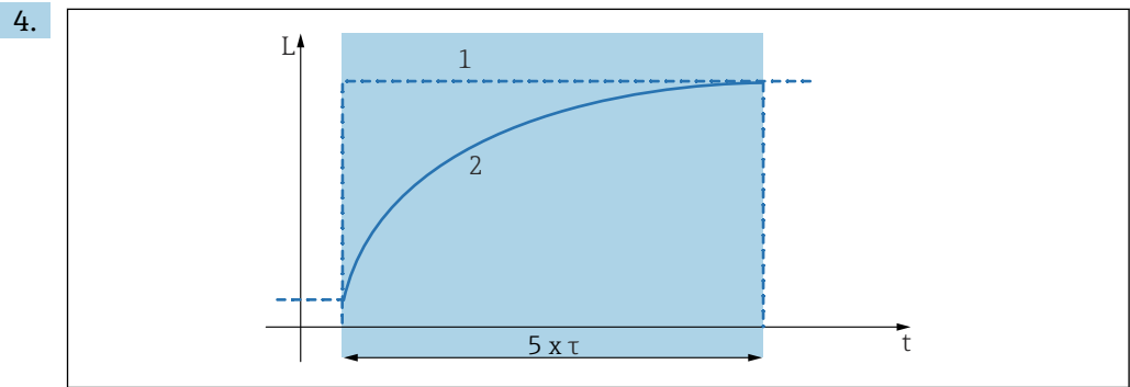
60 输出阻尼时间 1 测量值 2 输出电流
