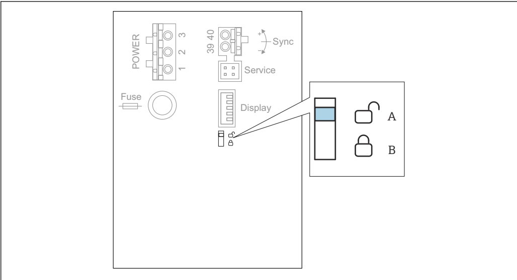
图 63 硬件锁定
