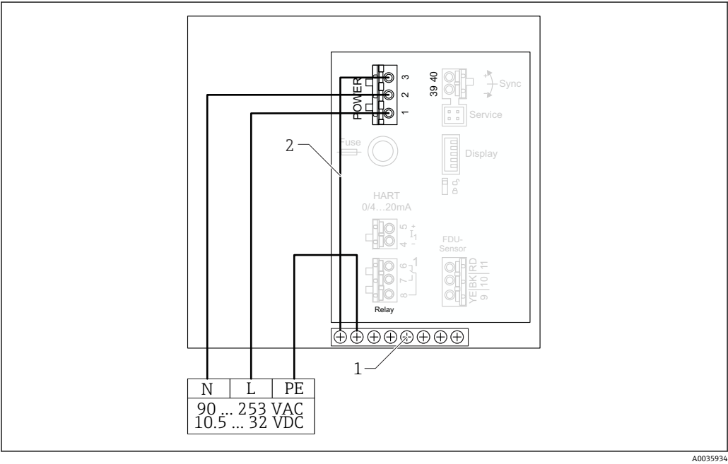
图 22 聚碳酸酯现场型外壳内的电源连接
