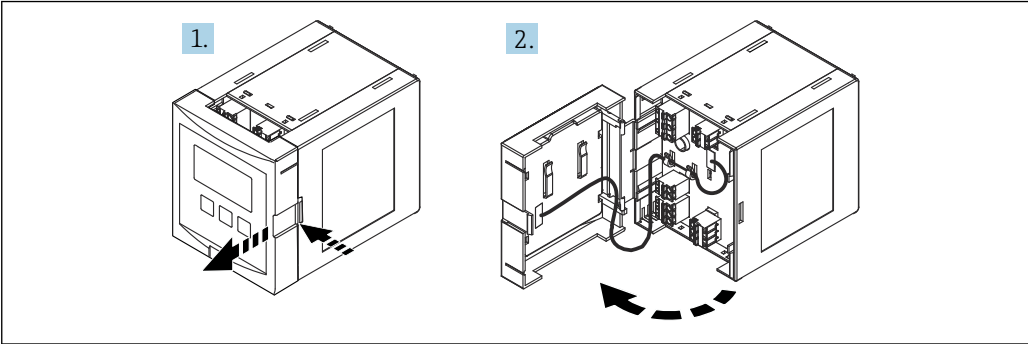
19 接线腔检修口：单个 DIN 导轨外壳单元
