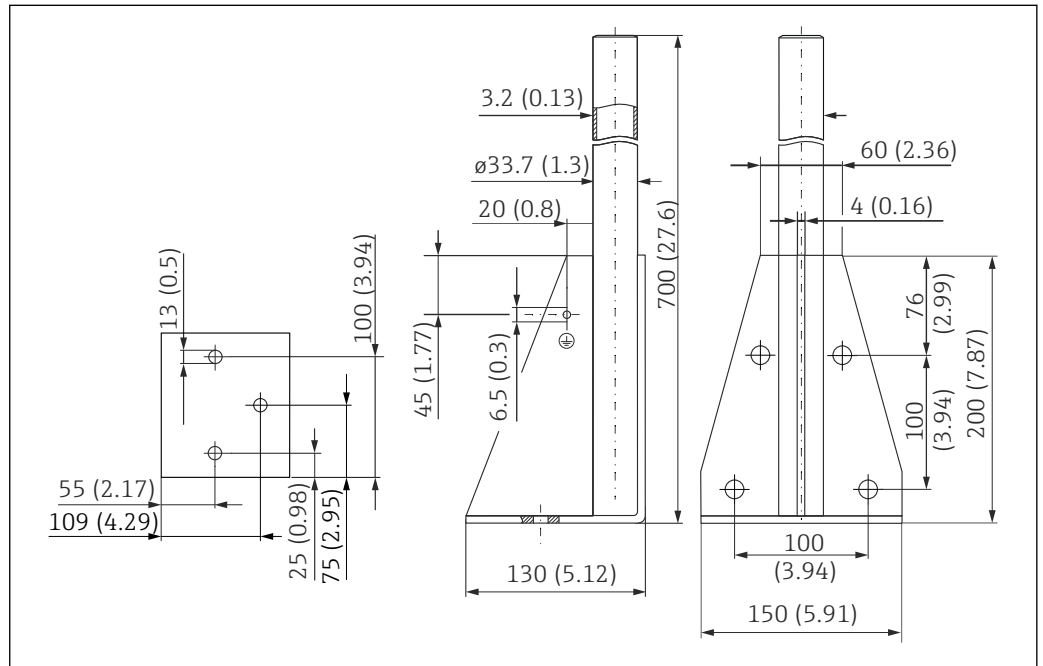
图 67 外形尺寸。测量单位 mm (in)
