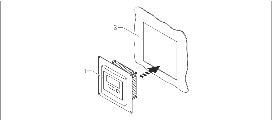
图 69 使用安装适配板
