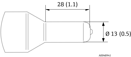
图 4. 1"直径 Rxn-41 探头末端；单位：mm (in)
