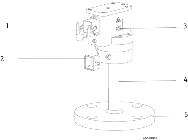
图 1. Rxn-41 探头
