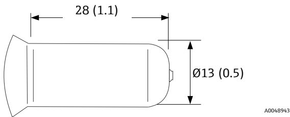
图 6. 2"直径 Rxn-41 探头末端; 单位: mm (in)
