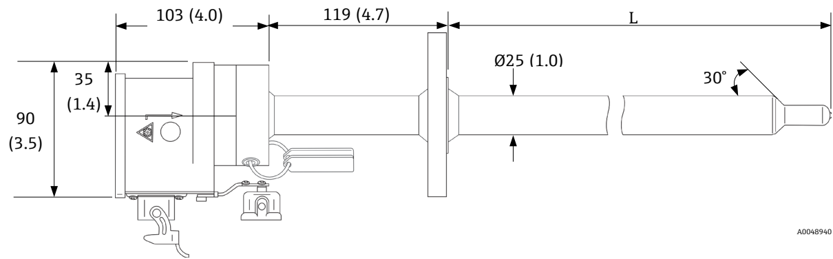
图 3. 1"直径 Rxn-41 探头；单位：mm (in) L = 浸入深度，取决于规格参数
