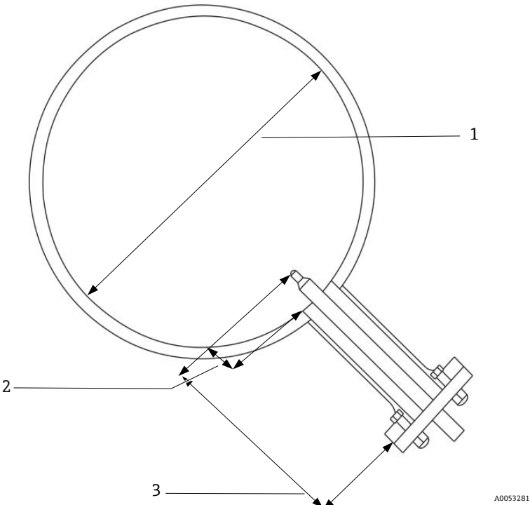
图 2: LNG 燃料加注船的 Rxn-41 探头安装参数
