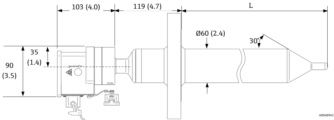
图 5. 2"直径 Rxn-41 探头; 单位: mm (in) L = 浸入深度, 取决于规格参数
