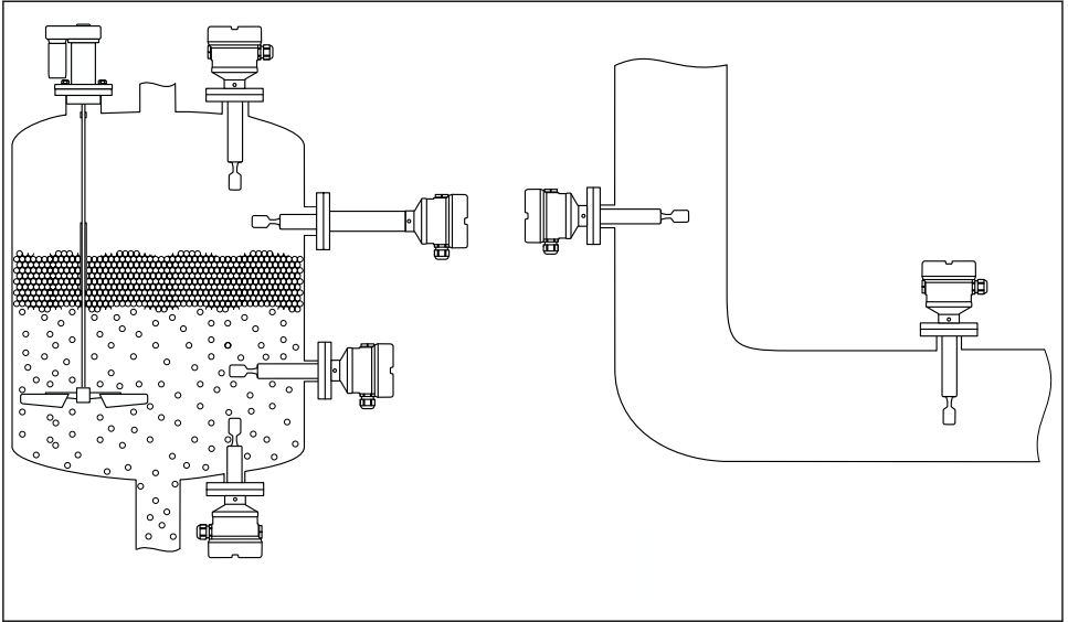
2 Esempi di installazione in recipiente, serbatoio o tubo
