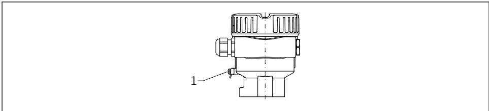
1 Morsetto di terra per il collegamento della linea di equalizzazione del potenziale (esempio)
