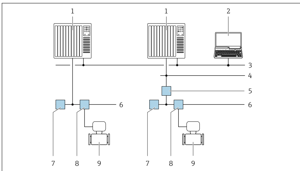
図 24 FOUNDATION Fieldbus ネットワークを介したリモート操作のオプション
