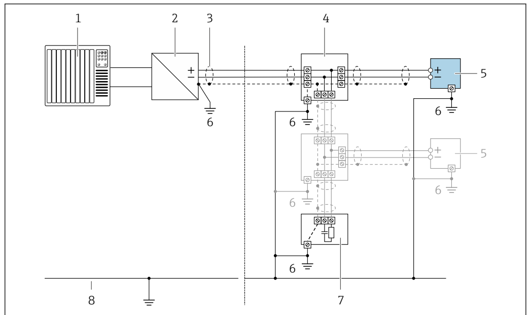
18 FOUNDATION Fieldbus の接続例
