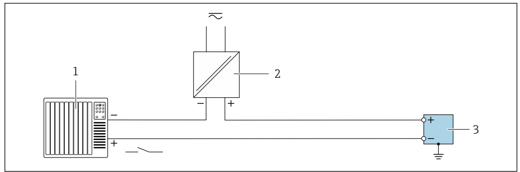
■ 17 ステータス入力の接続例
