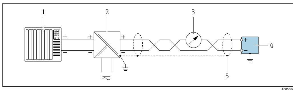
10 4～20 mA 電流出力（パッシブ）、HART 搭載の接続例
