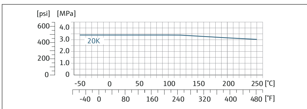
図 27 フランジ材質 1.4301 (SUS F304 相当) ; 接液部 アロイ C22
