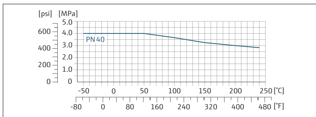
図 25 フランジ材質 1.4301 (SUS F304 相当) ; 接液部 アロイ C22
