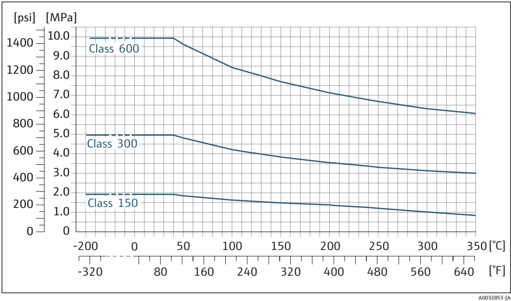
図 21 フランジ材質 1.4404 (SUS F316 相当または SUS F316L 相当)
