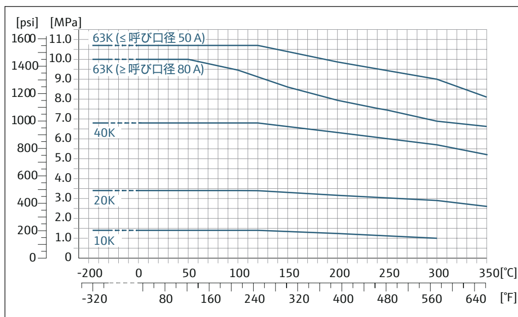
図 23 フランジ材質 1.4404 (SUS F316 相当または SUS F316L 相当)、アロイ C22
