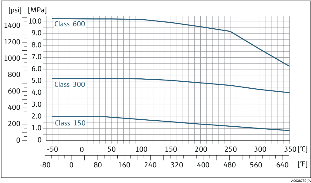
図 22 フランジ材質 アロイ C22
