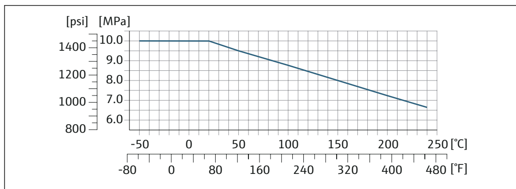
図 32 接続部の材質 1.4404 (SUS 316 相当または SUS 316L 相当)
