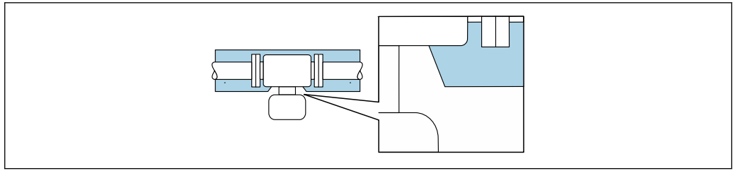
図 33 伸長ネックを覆わない断熱材：
