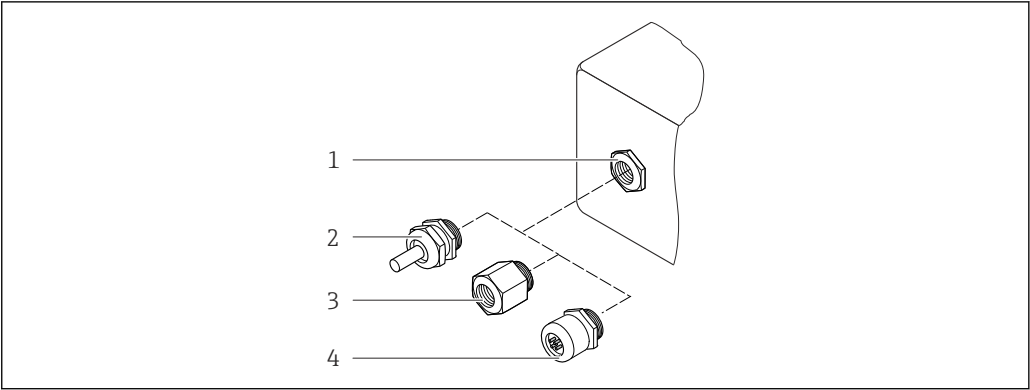
48 可能な電線口/ケーブルグランド
