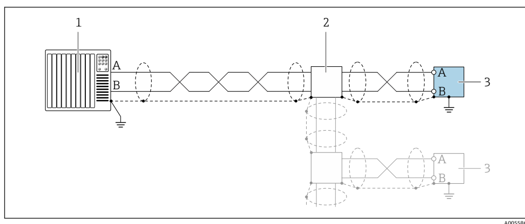
11 Modbus RS485 の接続例
