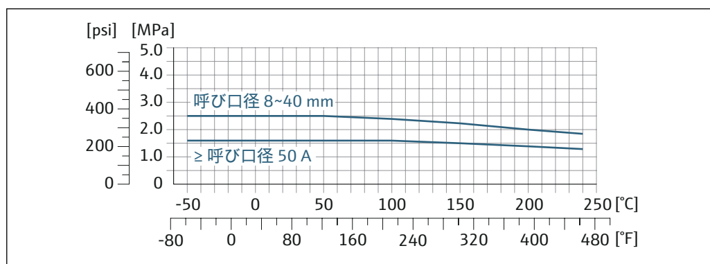
図 24 接続部の材質 1.4404 (SUS 316 相当または SUS 316L 相当)
