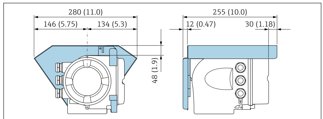
図 43 Proline 500 用の日除けカバー、単位 mm (in)
