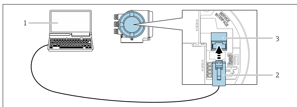
図 63 サービスインタフェース (CDI-RJ45) 経由の接続
