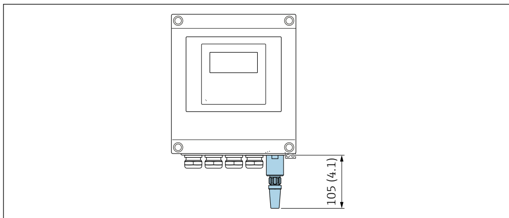
図 44 単位 mm (in)
