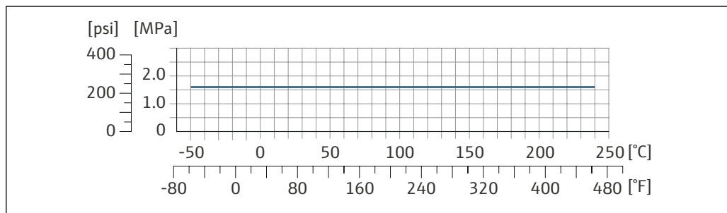
図 31 接続部の材質 1.4404 (SUS 316 相当または SUS 316L 相当)
