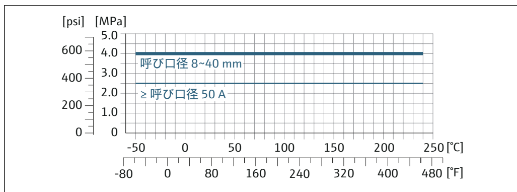
図 29 接続部の材質 1.4404 (SUS 316 相当または SUS 316L 相当)
