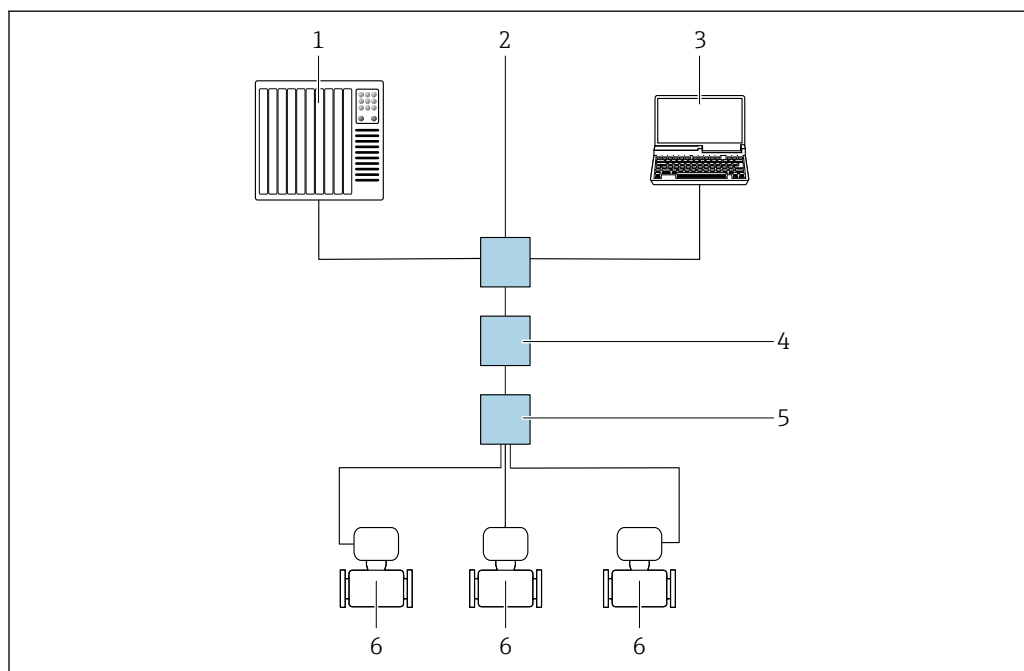
図 60 Modbus TCP over Ethernet-APL プロトコル経由のリモート作用オプション（アクティブ）
