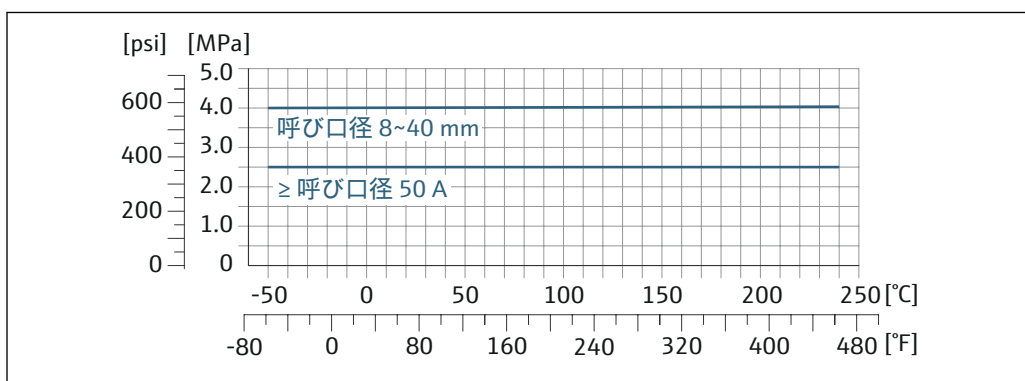
図 28 接続部の材質 1.4404 (SUS 316 相当または SUS 316L 相当)
