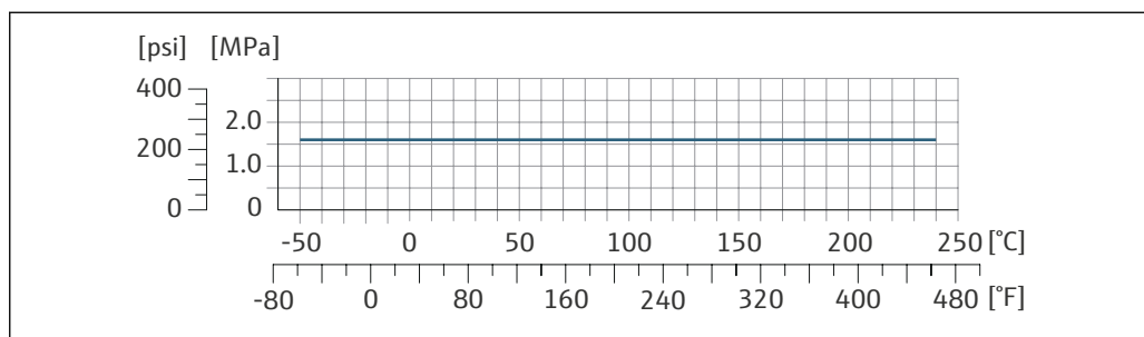
図 30 接続部の材質 1.4404 (SUS 316 相当または SUS 316L 相当)
