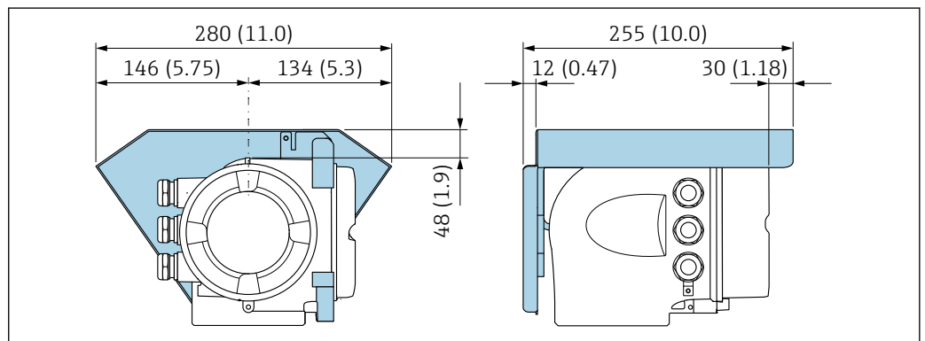
37 Proline 500 用の日除けカバー、単位 mm (in)
