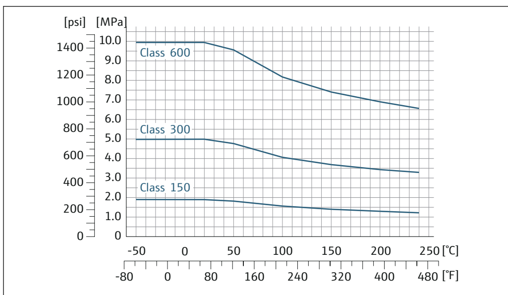
図 26 フランジ材質 1.4301 (SUS F304 相当) ; 接液部 アロイ C22
