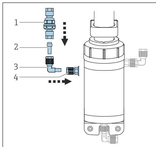
17 Montera rengöringsanslutningen 1 Backventil 2 Nippel 3 Vinkelanslutning 4 Slanganslutning
