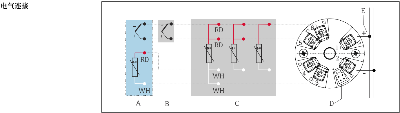
3 模块化温度变送器的接线端子分配 A 传感器输入（热电偶（TC）信号），外部冷端（CJ）Pt1000 B 传感器输入（热电偶（TC）信号），内部冷端（CJ） C 传感器输入（热电阻（RTD）信号）：四线制、三线制、两线制连接 D CDI 接口 E 电源
