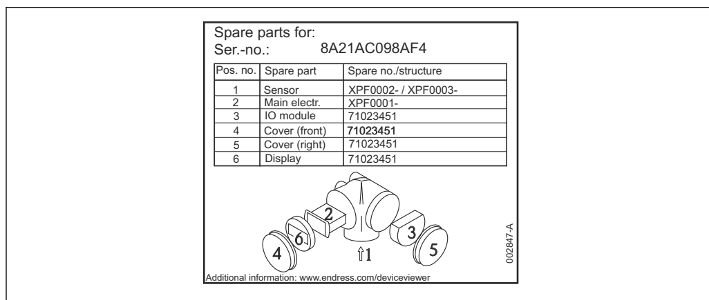
26 Beispiel für Ersatzteiltypenschild im Anschlussraumdeckel
