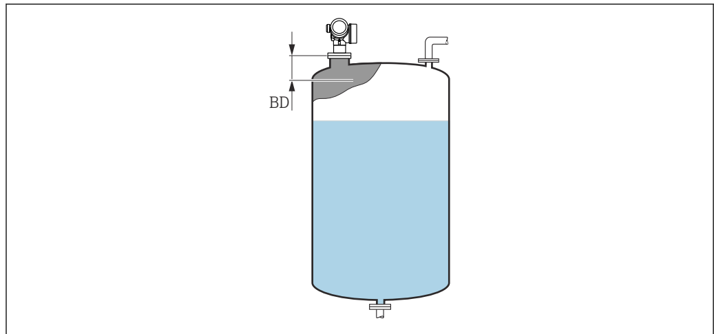
36 Blockdistanz (BD) bei Messung in Flüssigkeiten
