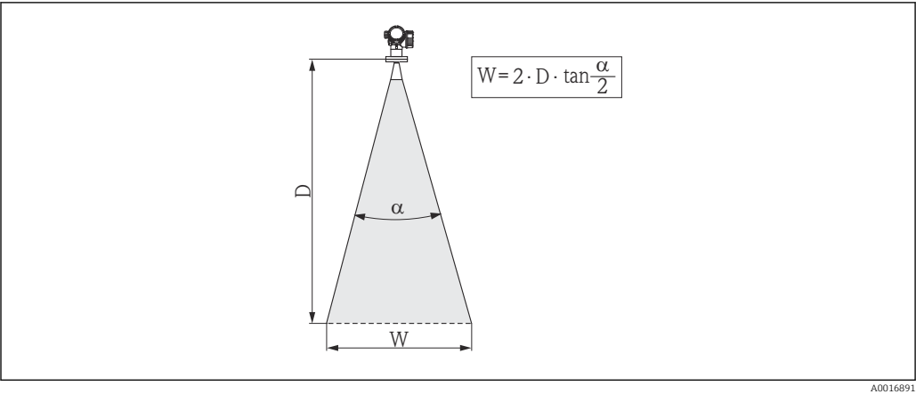
5 Zusammenhang zwischen Abstrahlwinkel \alpha , Distanz D und Kegelweite W
