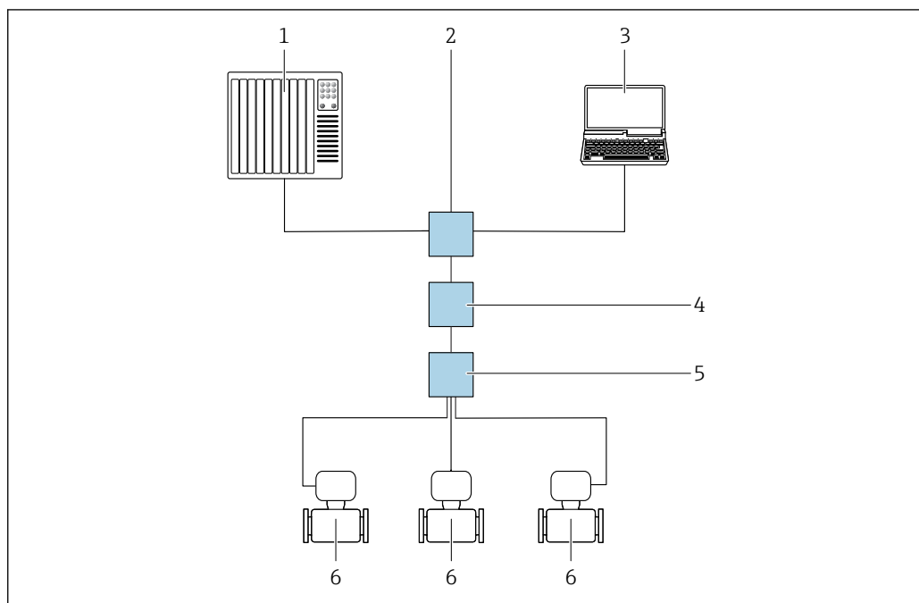
25 Opzioni per il funzionamento a distanza mediante rete APL
