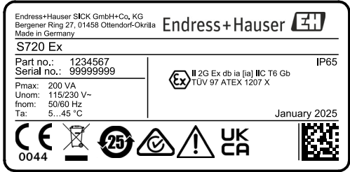
图 4: 铭牌 S720 Ex
