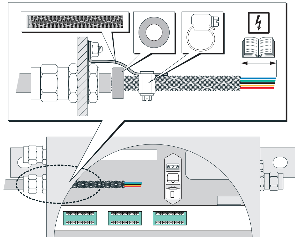
图 11：连接 S720 Ex/S721 Ex 的信号电缆
