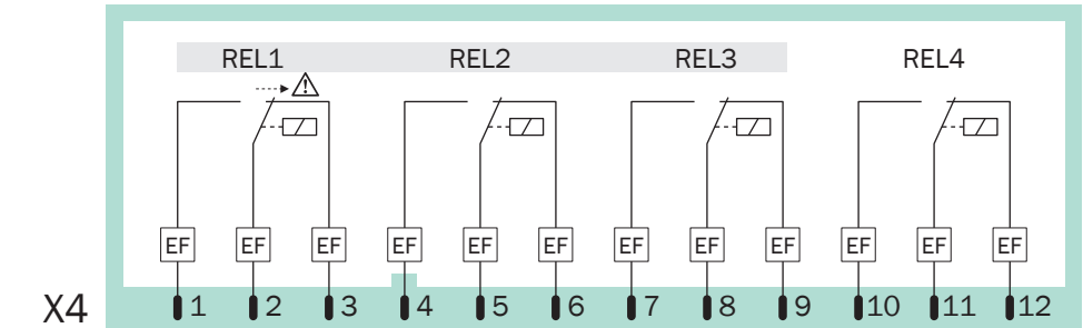
图 18: 插接件 X4（继电器开关量输出）
