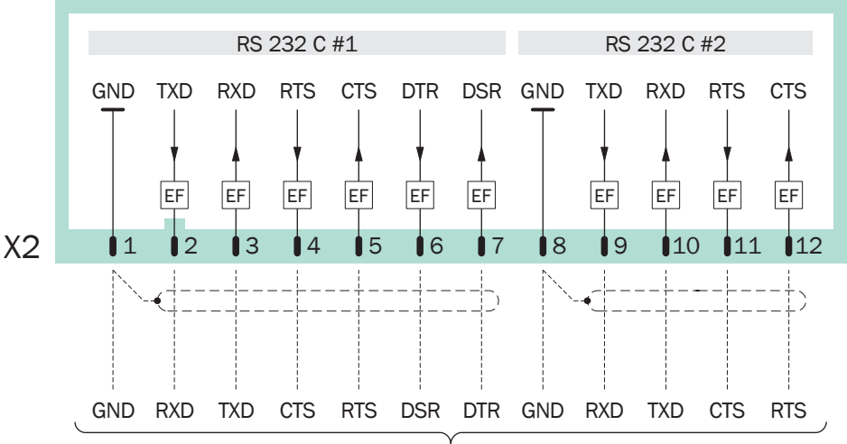
图 23: 插接件 X2 (接口)
