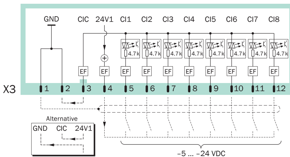
图 21: 插接件 X3 (控制输入)
