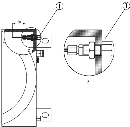
图 9: 安装细图
