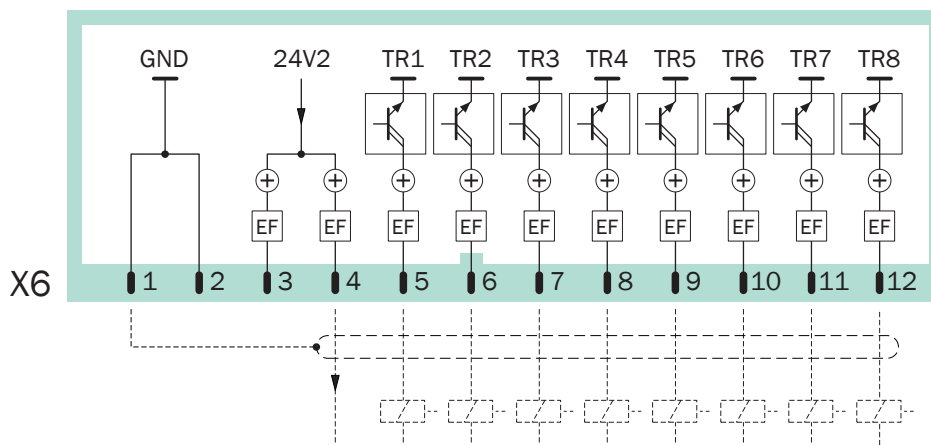
图 20: 插接件 X6 (晶体管开关量输出)
