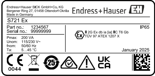
图 5: 铭牌 S721 Ex
