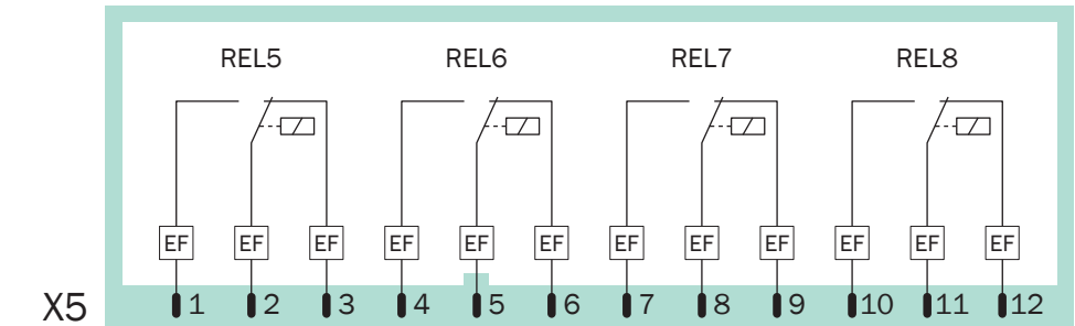
图 19: 插接件 X5（继电器开关量输出）
