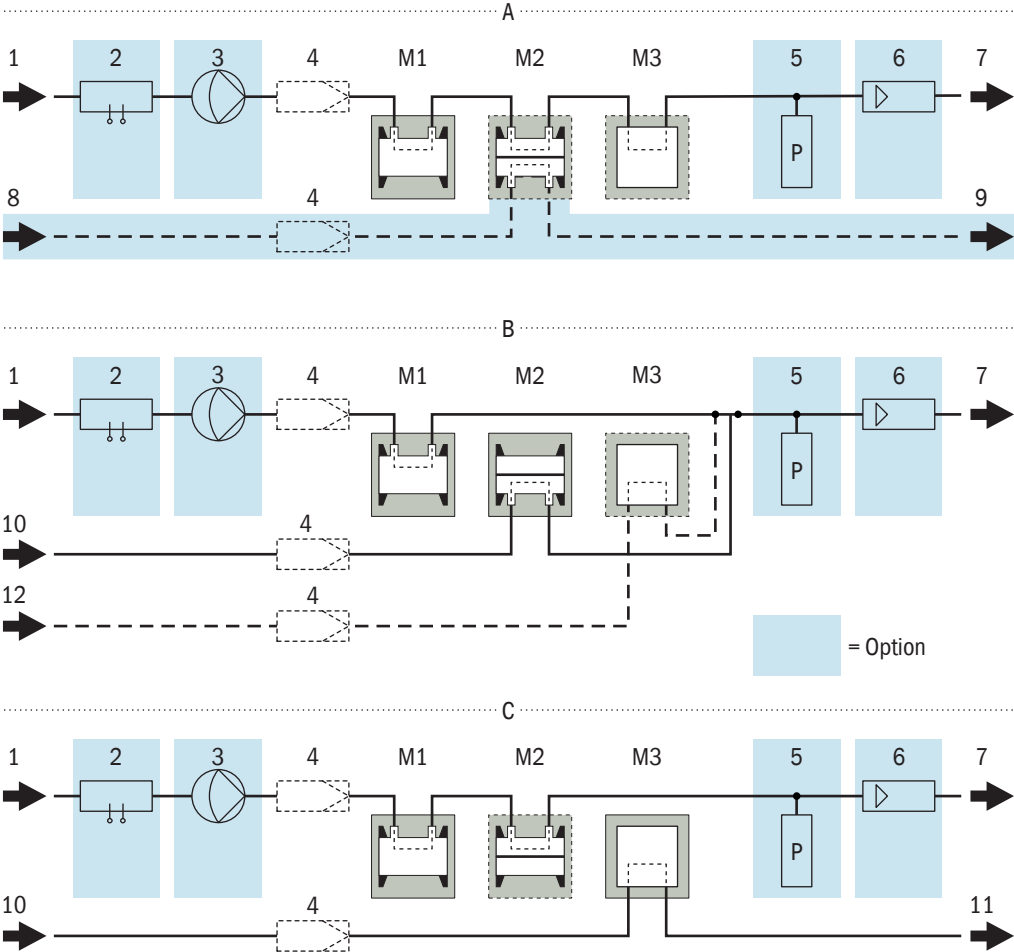
图 38: 内部气流（标准流程图）
