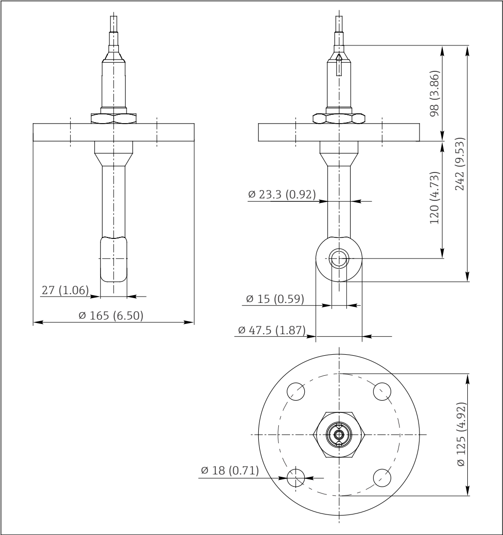
18 Versión, brida EN1092-1 DN 50 PN 16, placa de sellado del sensor de PFA soldado en 316L. Unidad de medida mm (in)
