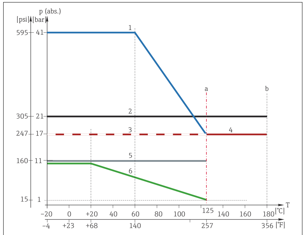
14 Curvas de temperatura/presión
