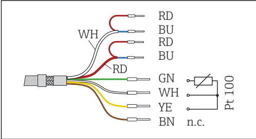
4 CLK6 para alargar el CLS50
