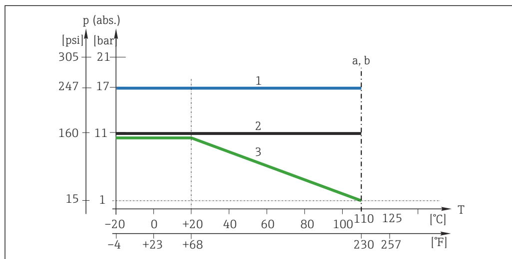
13 Curvas de temperatura/presión
