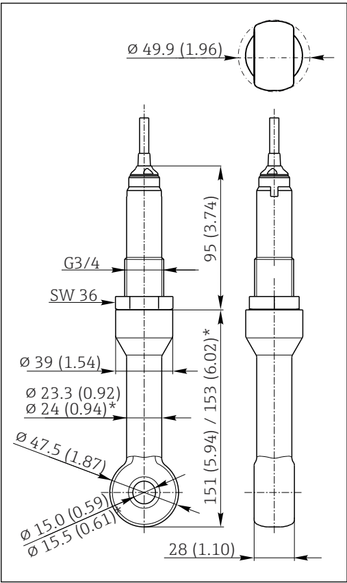
16 Versión con rosca G3/4. Unidad de medida mm (in)
