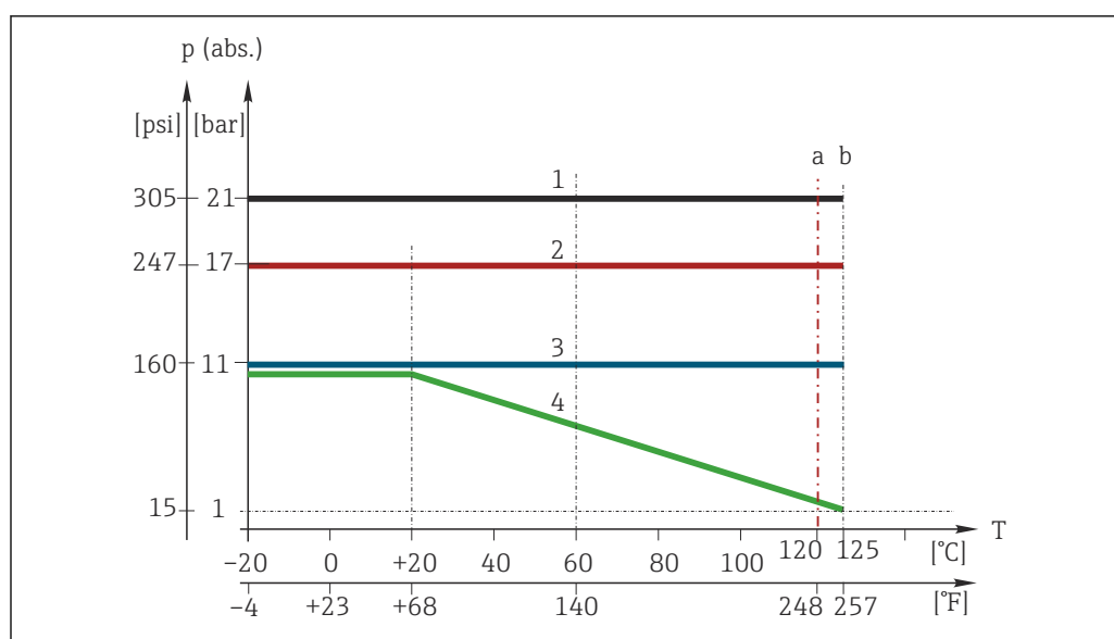
12 Curvas de temperatura/presión
