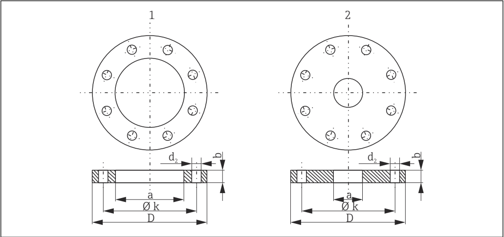
19 Dimensiones de la brida
