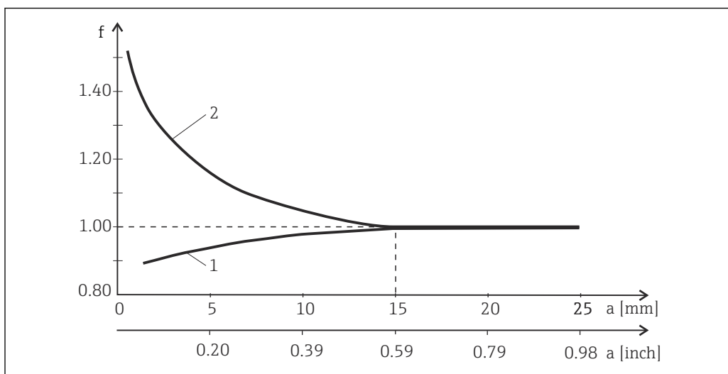
6 Relación entre el factor de instalación f y la distancia a la pared
