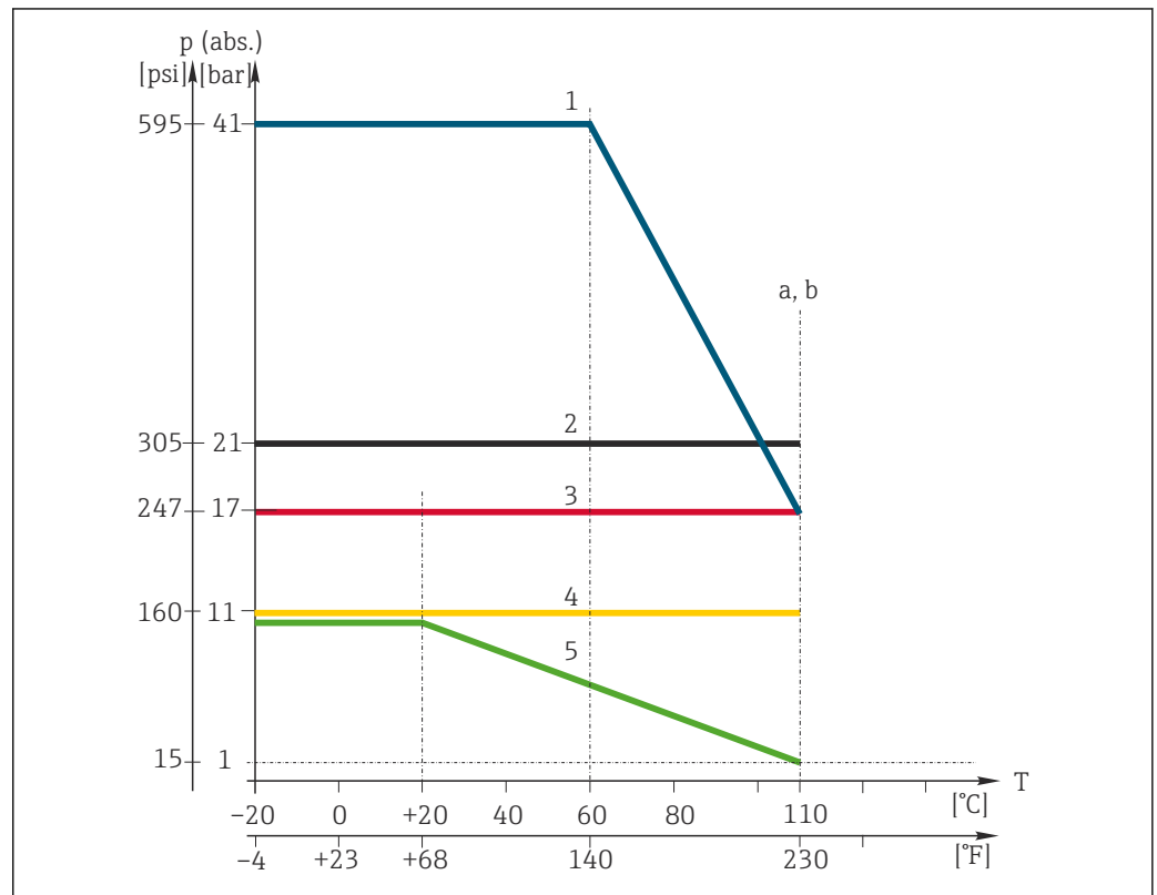
11 Curvas de temperatura/presión
