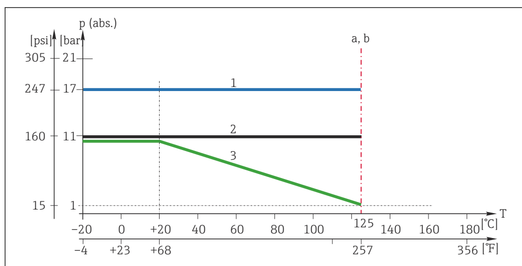
15 Curvas de temperatura/presión
