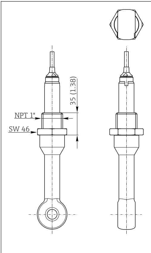
17 Versión, rosca NPT 1". Unidad de medida mm (in)
