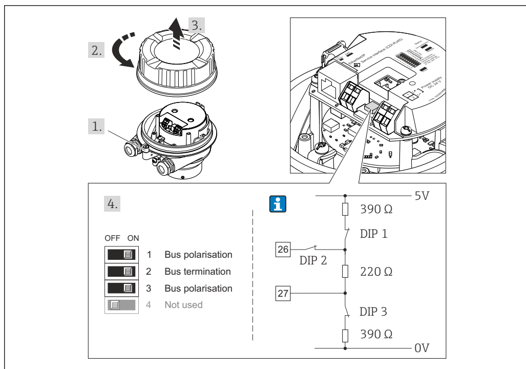
図 11 I/O 電子モジュールの DIP スイッチを使用した終端処理（通信速度 < 1.5 MBaud の場合）
