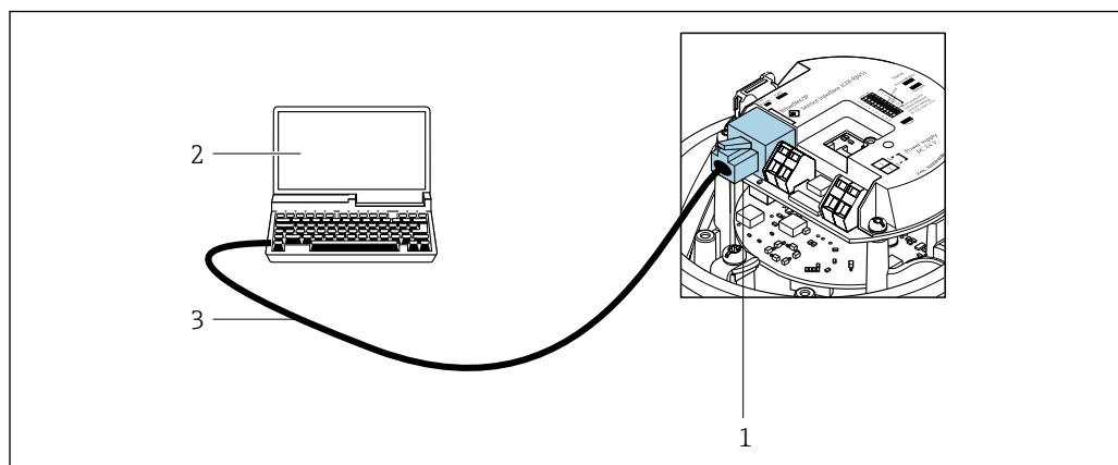
図 14 「出力」のオーダーコードの接続、オプション L : PROFIBUS DP
