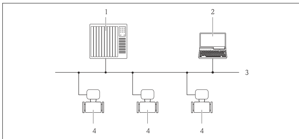
図 13 PROFIBUS DP ネットワークを介したリモート操作のオプション
