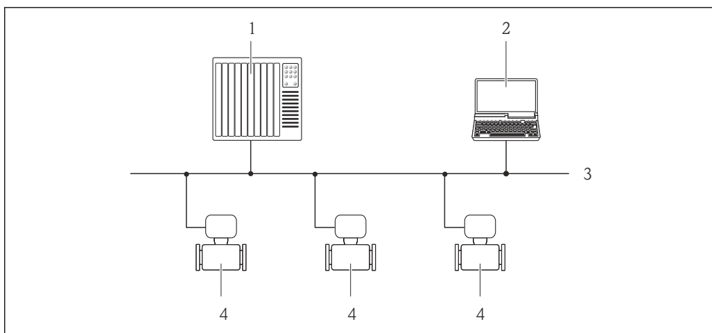
図 18 PROFIBUS DP ネットワークを介したリモート操作のオプション
