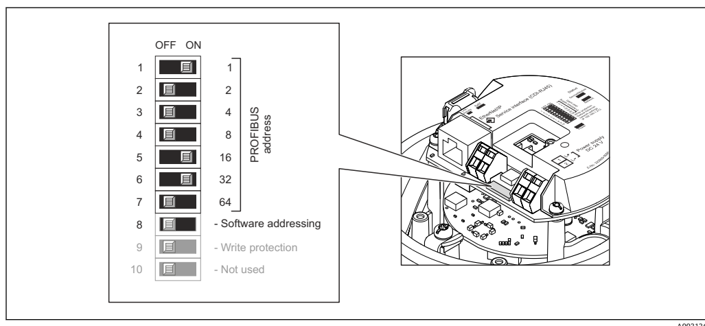
図 10 I/O 電子モジュール上の DIP スイッチを使用したアドレス指定
