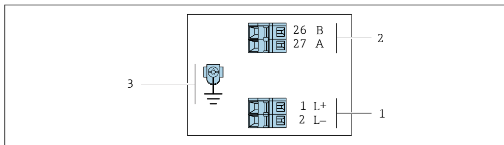
図 6 PROFIBUS DP 端子の割当て
