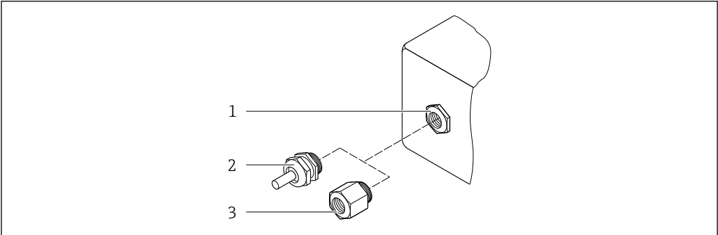
図 17 可能な電線口/ケーブルグランド
