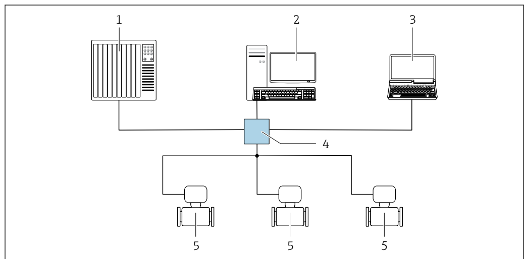
图 34 通过 EtherNet/IP 网络进行远程操作：星形拓扑结构
