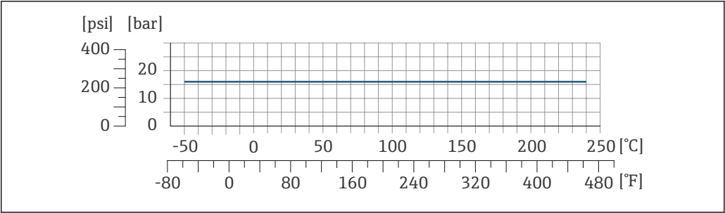
图 26 连接部件材质: 1.4404 (316/316L)
