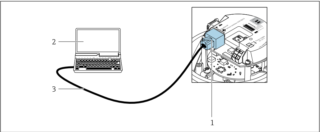
图 39 订购选项“输出”，选型代号 R: PROFINET
