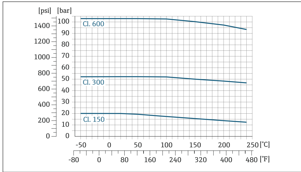
图 17 法兰材质: Alloy C22 合金
