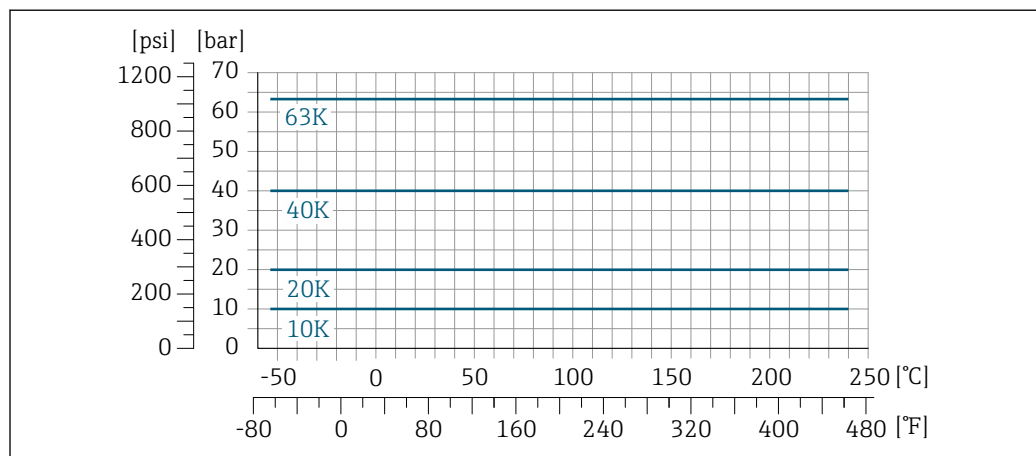
图 18 法兰材质: 1.4404 (F316/F316L)、Alloy C22 合金
