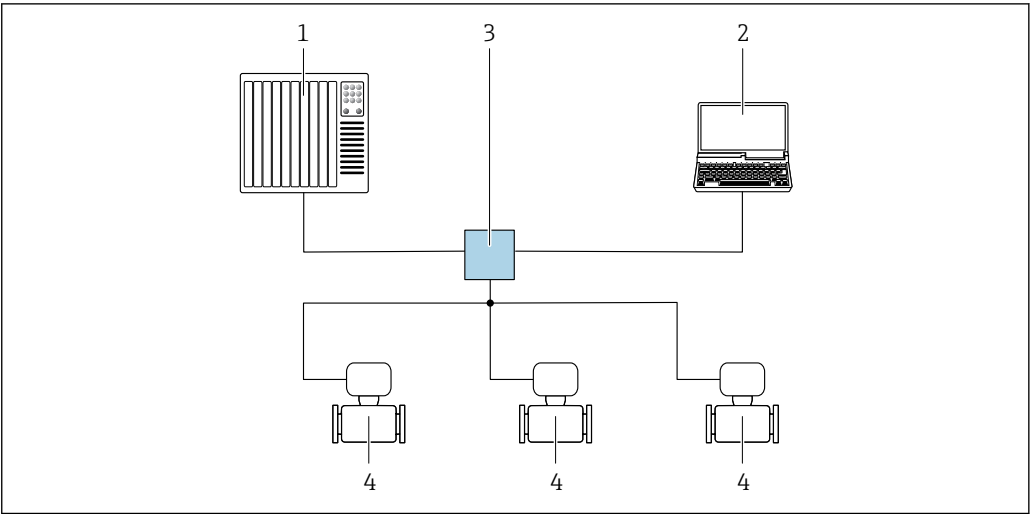
图 35 通过 PROFINET 网络进行远程操作：星形拓扑结构
