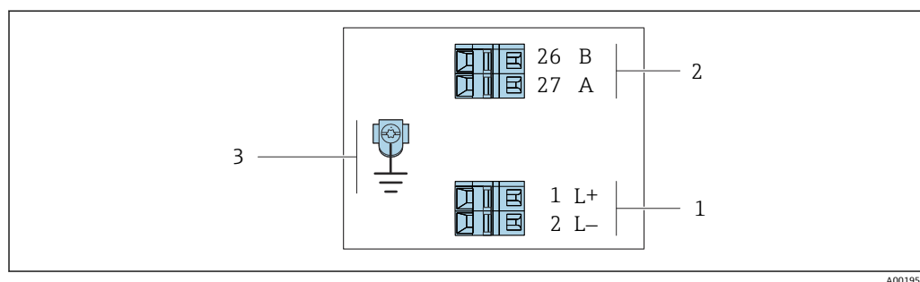
图 4 接线端子分配: Modbus RS485, 在非防爆危险区和 Zone 2/ Div. 2 防爆危险区中使用
