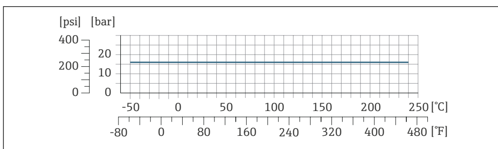
图 25 连接部件材质: 1.4404 (316/316L)
