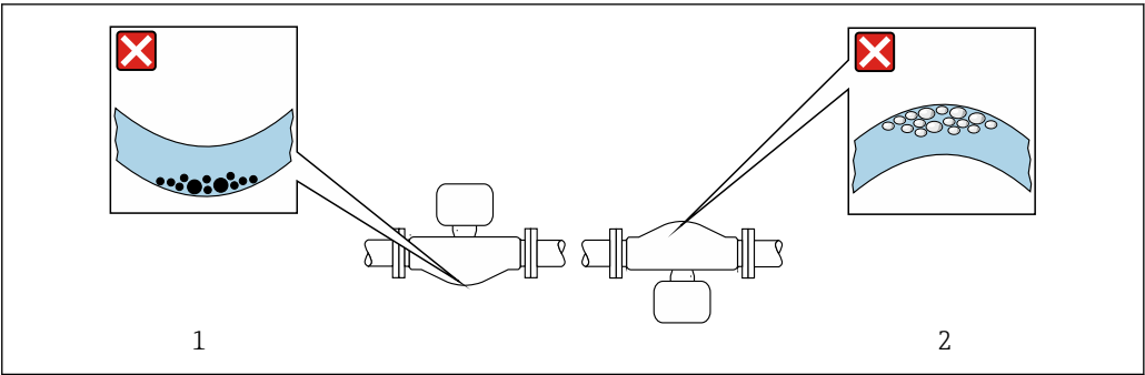
☒ 13 弯测量管传感器的安装方向
