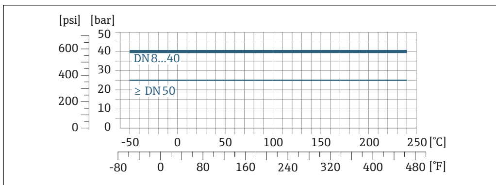
图 24 连接部件材质: 1.4404 (316/316L)
