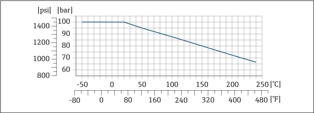
图 27 连接部件材质: 1.4404 (316/316L)
