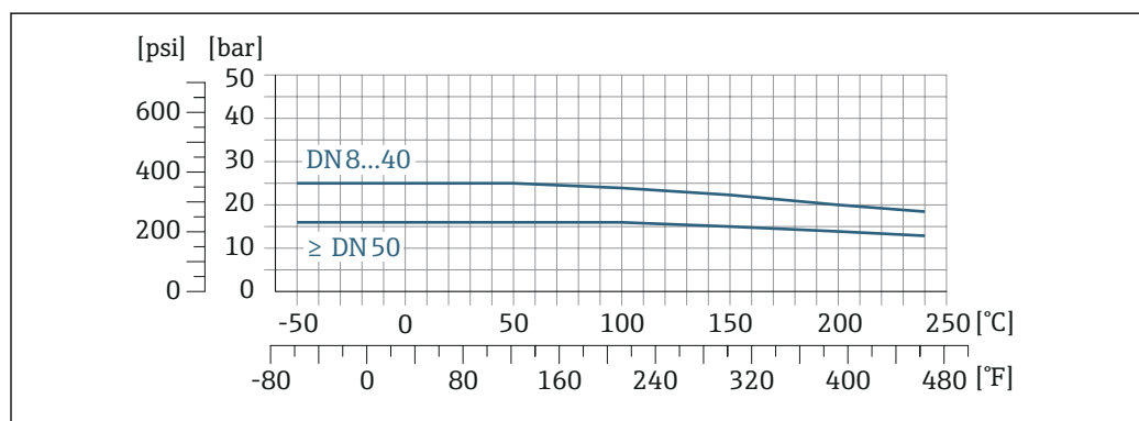
图 19 连接部件材质: 1.4404 (316/316L)
