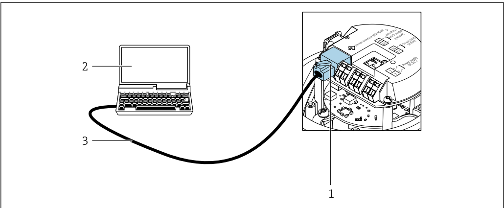
图 36 订购选项“输出”，选型代号 B：4...20 mA HART，脉冲/频率/开关量输出
