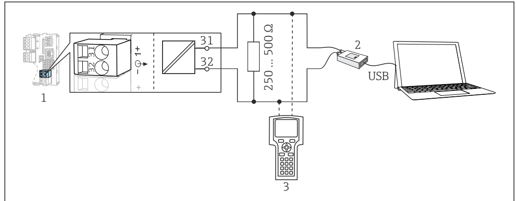
19 Передача данных по протоколу HART посредством модема
