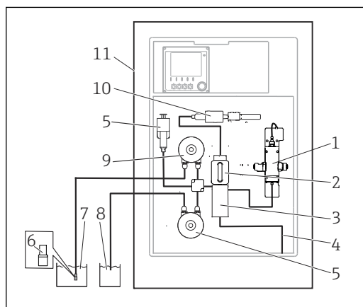
2 Измерительная система на основе Liquiline System CA80TP и впускного сетчатого фильтра
