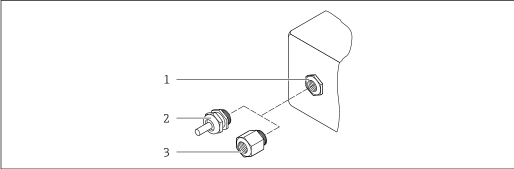
図 36 可能な電線口/ケーブルグランド 1 めねじ M20 × 1.5 2 ケーブルグランド M20 × 1.5 3 電線口用アダプタ (めねじ G ½" または NPT ½")
