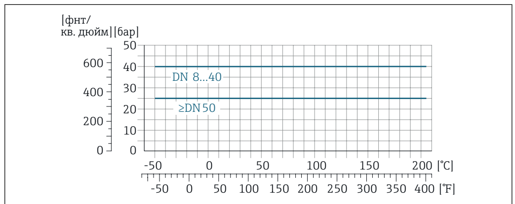
21 С материалом присоединения 1.4435 (316L)
