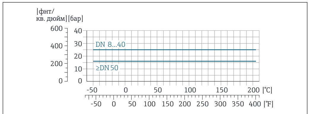
19 С материалом фланца 1.4435 (316L)
