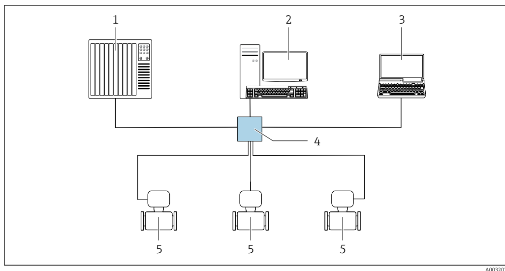
▣ 33 Варианты дистанционного управления через сеть EtherNet/IP: топология «звезда»
