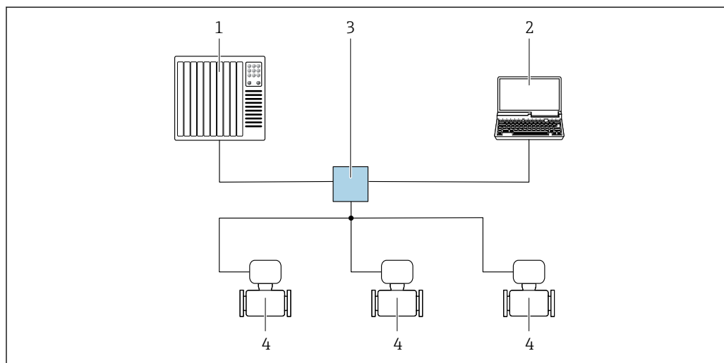
▣ 34 Варианты дистанционного управления через сеть PROFINET: топология «звезда»
