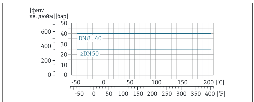
20 С материалом фланца 1.4435 (316L)
