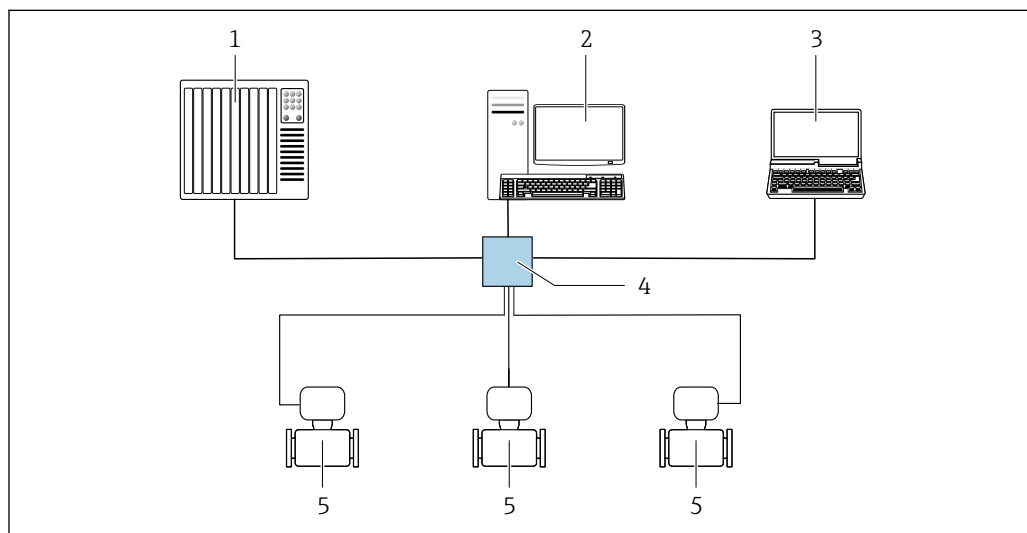
24 Варианты дистанционного управления через сеть EtherNet/IP: топология «звезда»
