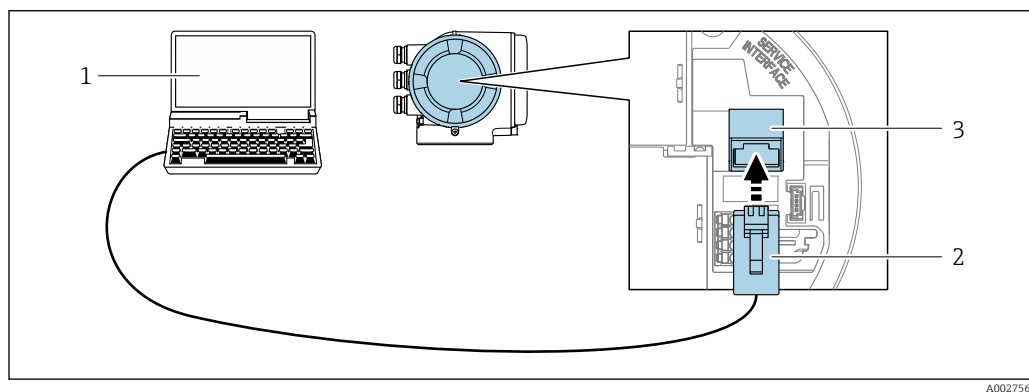
25 Connessione mediante interfaccia service (CDI-RJ45)
