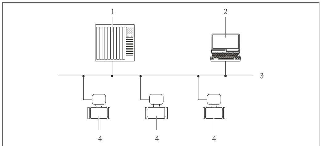
図 51 PROFIBUS DP ネットワークを介したリモート操作のオプション
