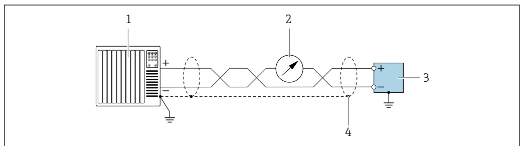
図 9 4～20 mA 電流出力（アクティブ）、HART 搭載の接続例
