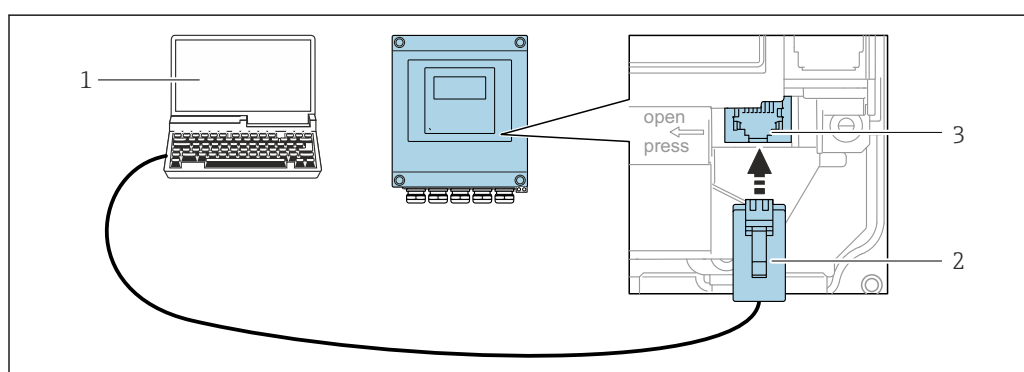
図 60 サービスインタフェース (CDI-RJ45) 経由の接続
