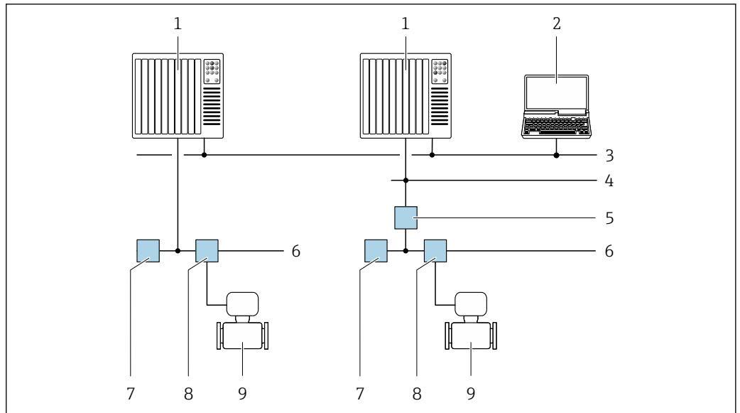
図 50 FOUNDATION Fieldbus ネットワークを介したリモート操作のオプション
