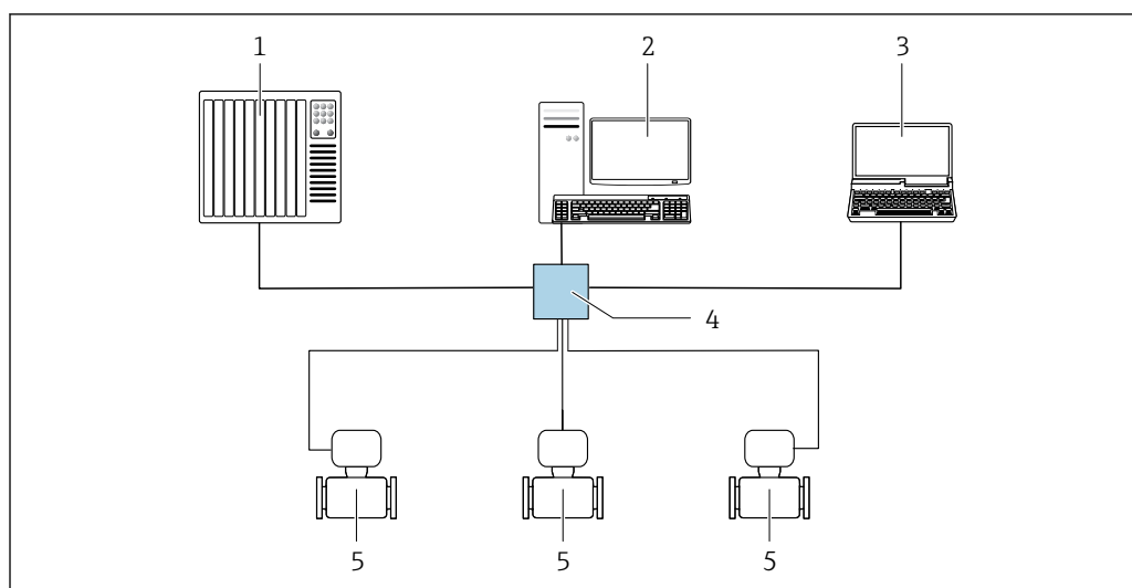
図 59 Modbus TCP over Ethernet - 100 Mbit/s 経由のリモート操作用オプション：スター型トポロジー
