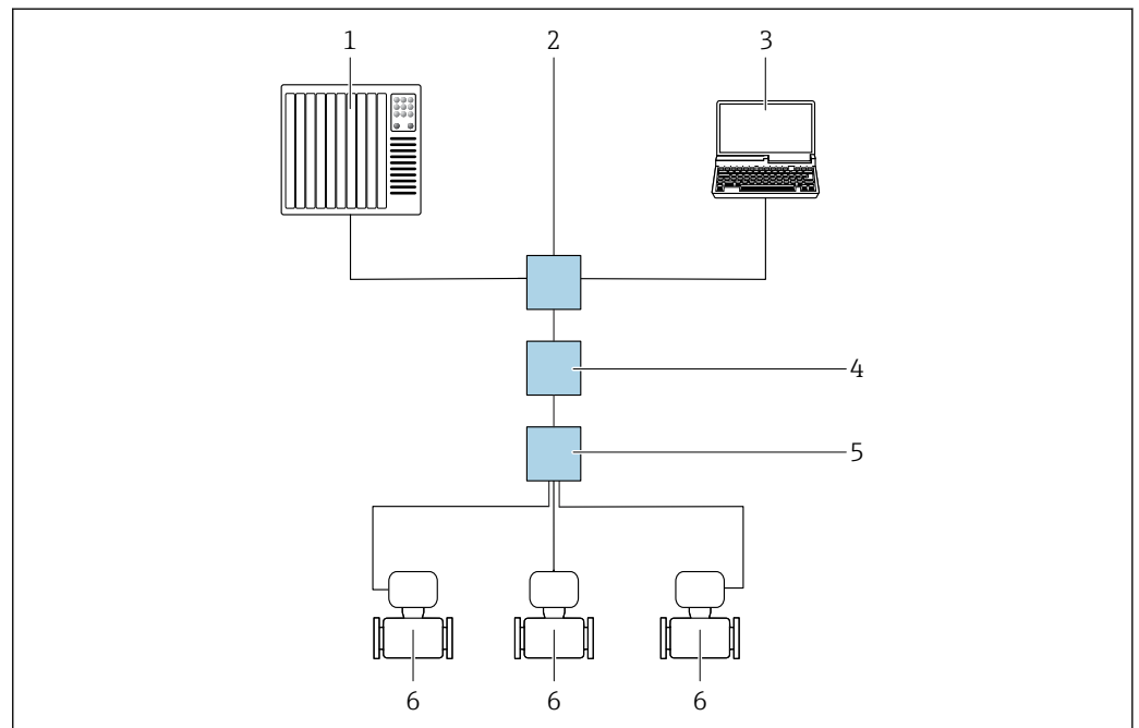
図 58 Modbus TCP over Ethernet-APL プロトコル経由のリモート操作用オプション（アクティブ）
