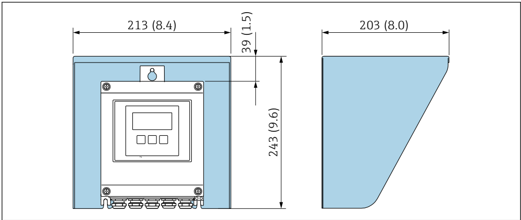
34 Proline 500 – デジタル用の日除けカバー、単位 mm (in)
