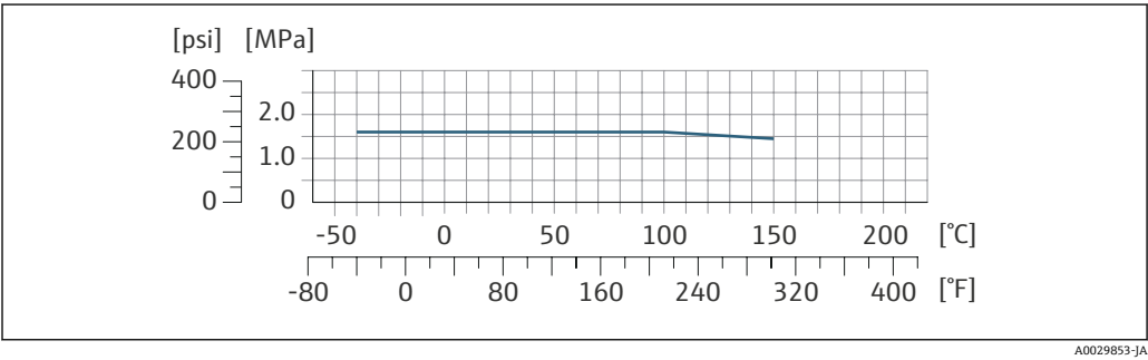
図 29 接続部の材質 1.4404 (SUS 316 相当または SUS 316L 相当)
