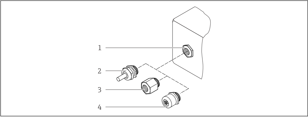
図 46 可能な電線口/ケーブルグランド
