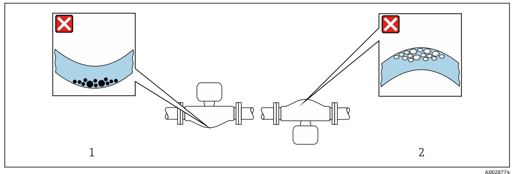
図 15 弓形計測チューブセンサの取付方向
