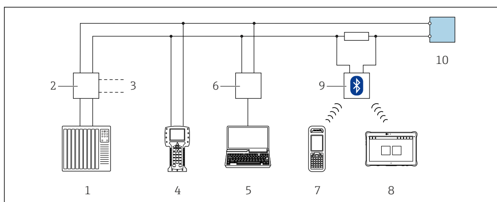
図 49 HART プロトコル経由のリモート操作用オプション（パッシブ）
