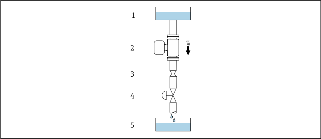
図 14 下向き垂直配管への設置（例：バッチアプリケーション用）
