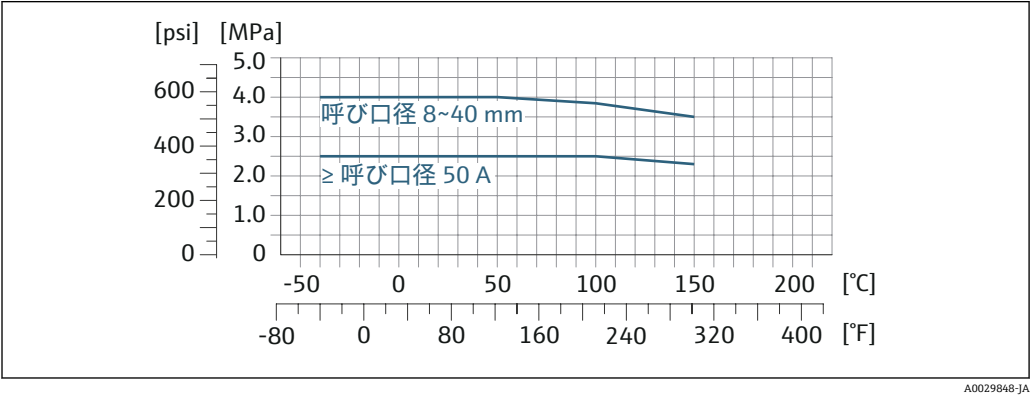
図 28 接続部の材質 1.4404 (SUS 316 相当または SUS 316L 相当)
