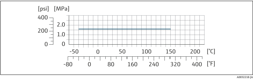
図 30 接続部の材質 1.4404 (SUS 316 相当または SUS 316L 相当)
