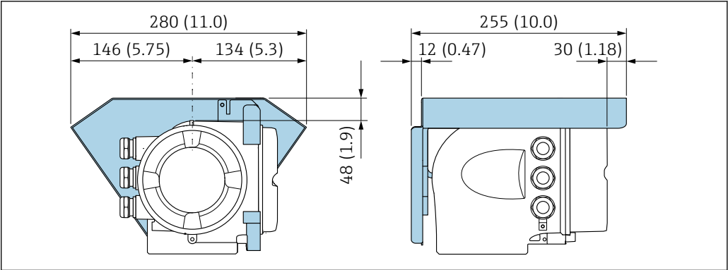
21 Proline 500 用の日除けカバー、単位 mm (in)
