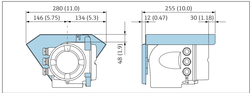
35 Proline 500 用の日除けカバー、単位 mm (in)
