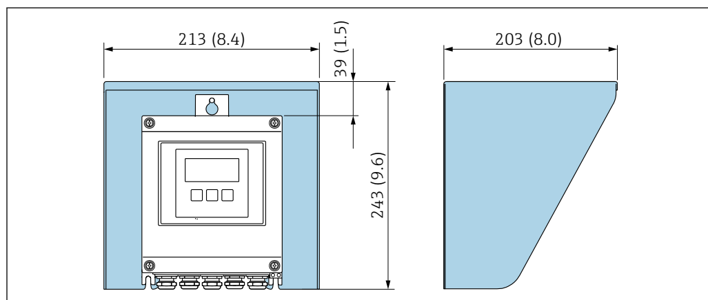
図 20 Proline 500 – デジタル用の日除けカバー、単位 mm (in)
