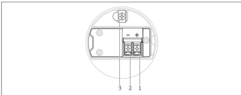
図 4 端子部の接続端子と接地端子
