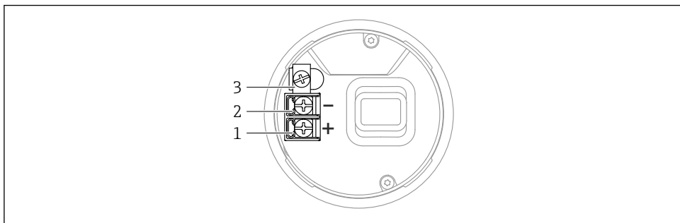
図 3 端子部の接続端子と接地端子（シングルコンパートメントハウジング）
