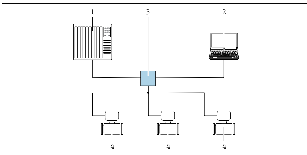
22 Варианты дистанционного управления через сеть PROFINET: топология «звезда»
