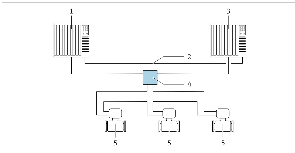
■ 25 Пример компоновки резервируемой системы (S2): кольцевая топология
