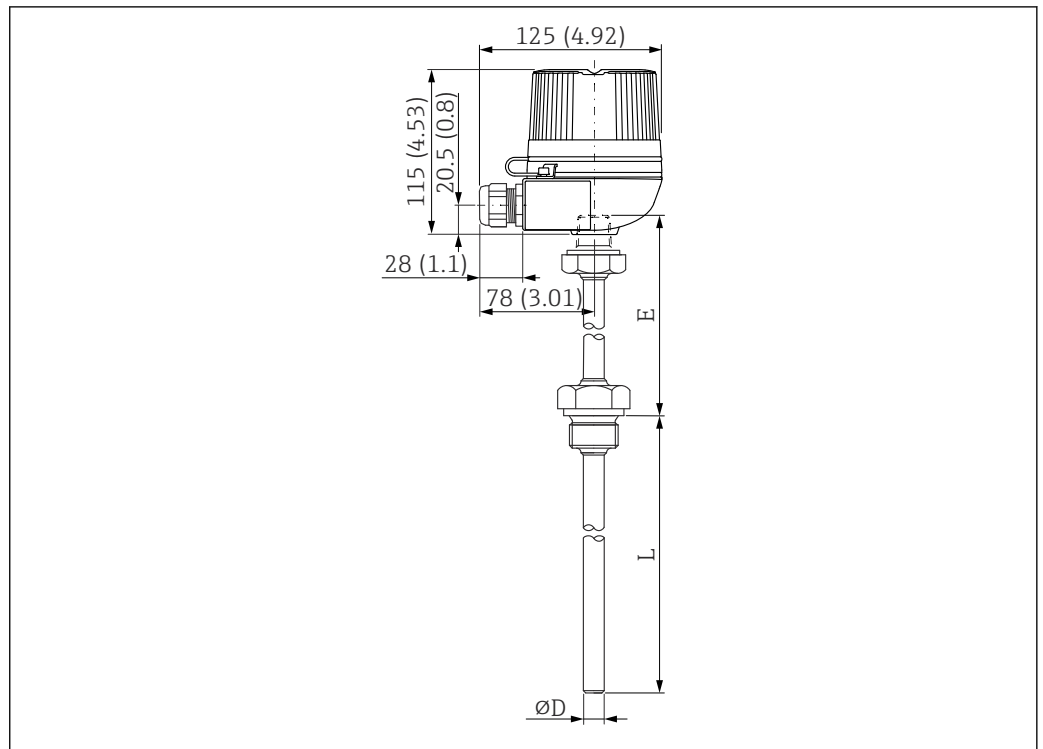
77 Structure de l'Omnigrad S TR61 ; dimensions : mm (in)
