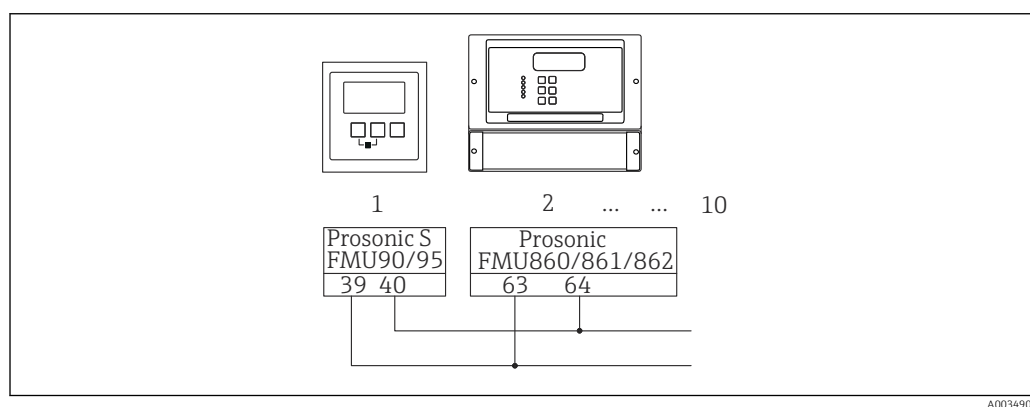
34 Synchronisation des FMU90/FMU95 avec le FMU86x
