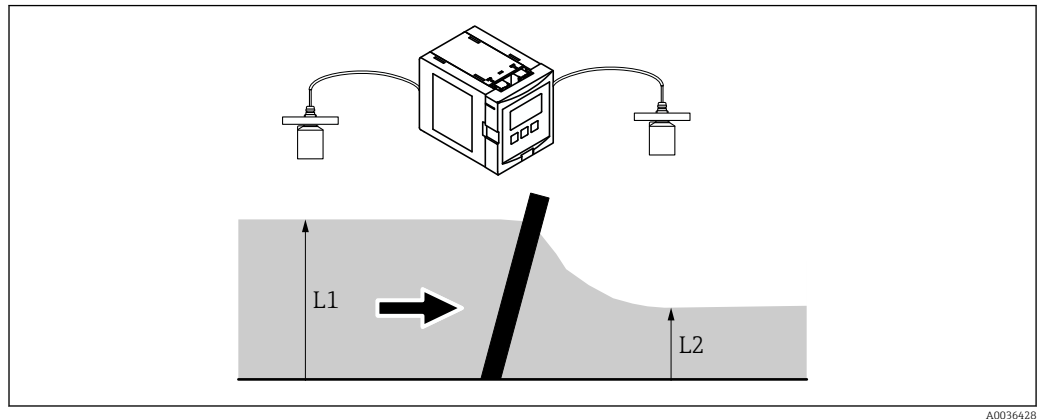
65 Principe de fonctionnement de la fonction de commande de dégrilleur
