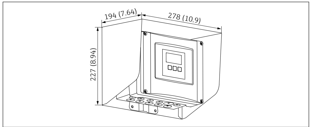
72 Capot de protection climatique pour boîtier de terrain en polycarbonate. Unité de mesure mm (in)
