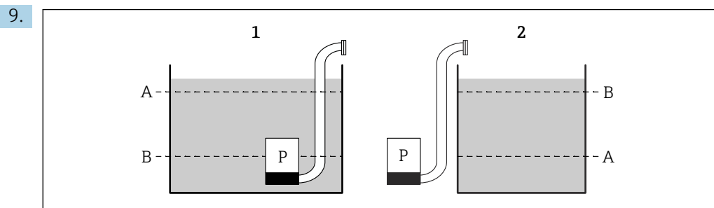
61 Point d'enclenchement et point de déclenchement pour la commande de limite
