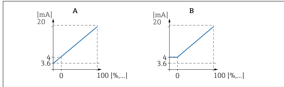
68 Seuil 4mA (uniquement pour plage de courant = 4 ... 20 mA)
