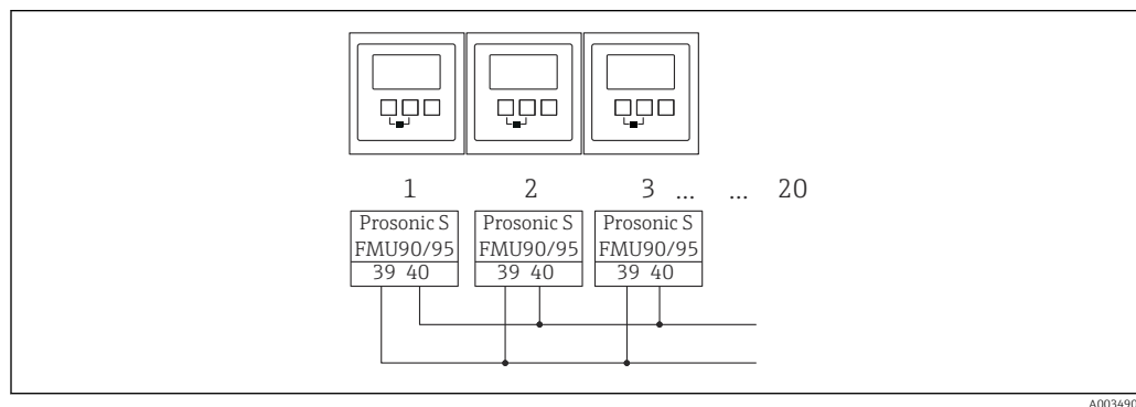
33 Synchronisation de plusieurs transmetteurs FMU90/FMU95
