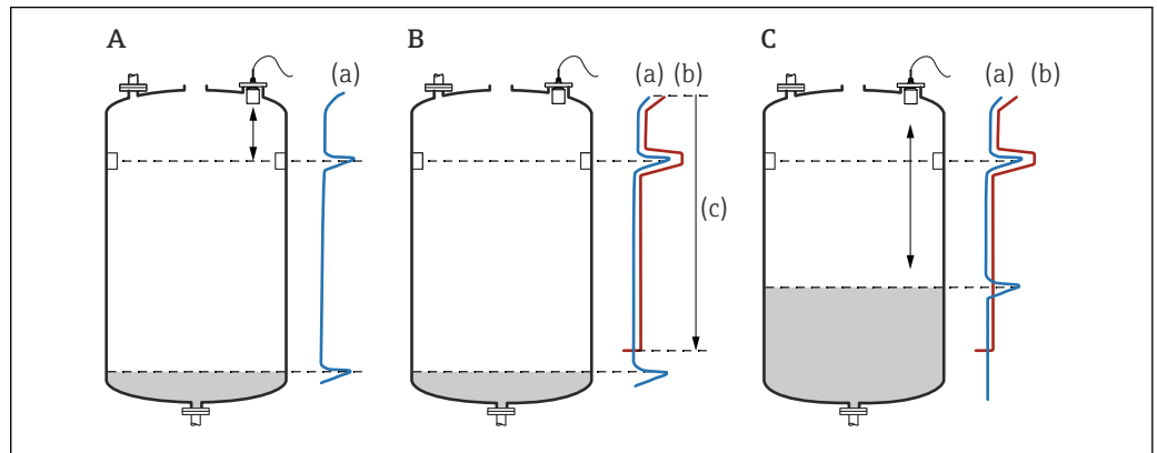
49 Principe de fonctionnement de la fonction de suppression des échos parasites ("mapping")
