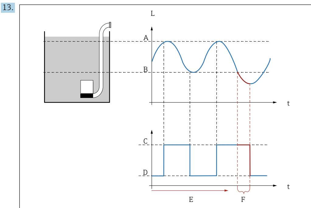
60 Effet des paramètres "Interva.réaction" et "Temps réaction"
