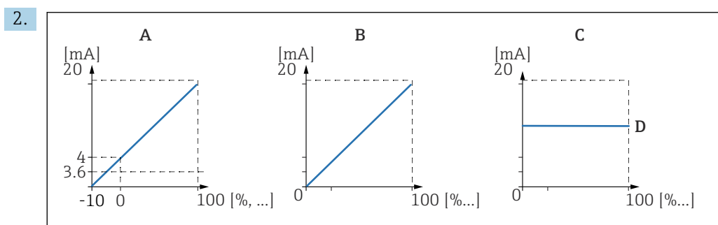
66 Étendue de mesure courant
