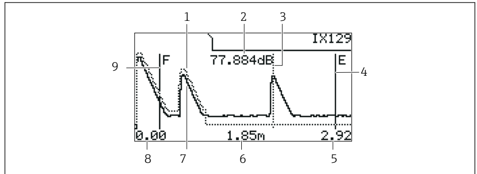
71 Courbe enveloppe sur l'afficheur local
