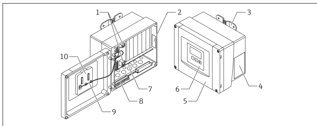
i 1 Composants du Prosonic S dans le boîtier de terrain en polycarbonate
