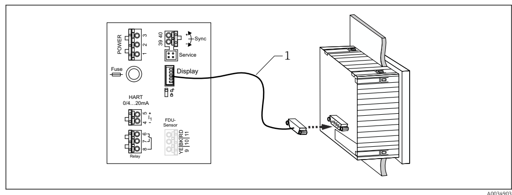
39 Raccordement du module d'affichage et de configuration séparé
