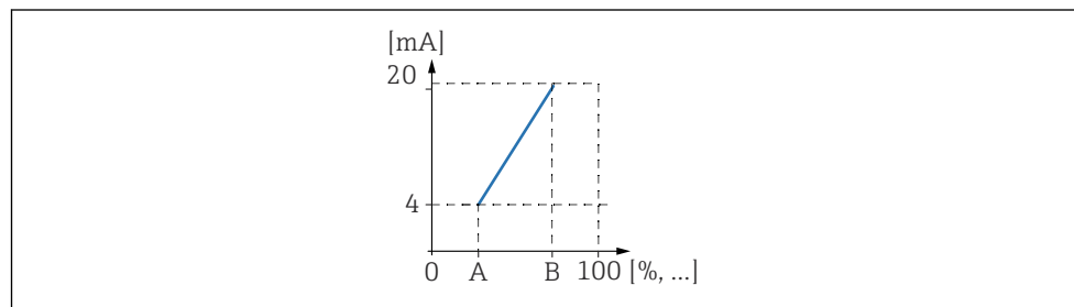
69 Principe de fonctionnement de la fonction zoom courant
