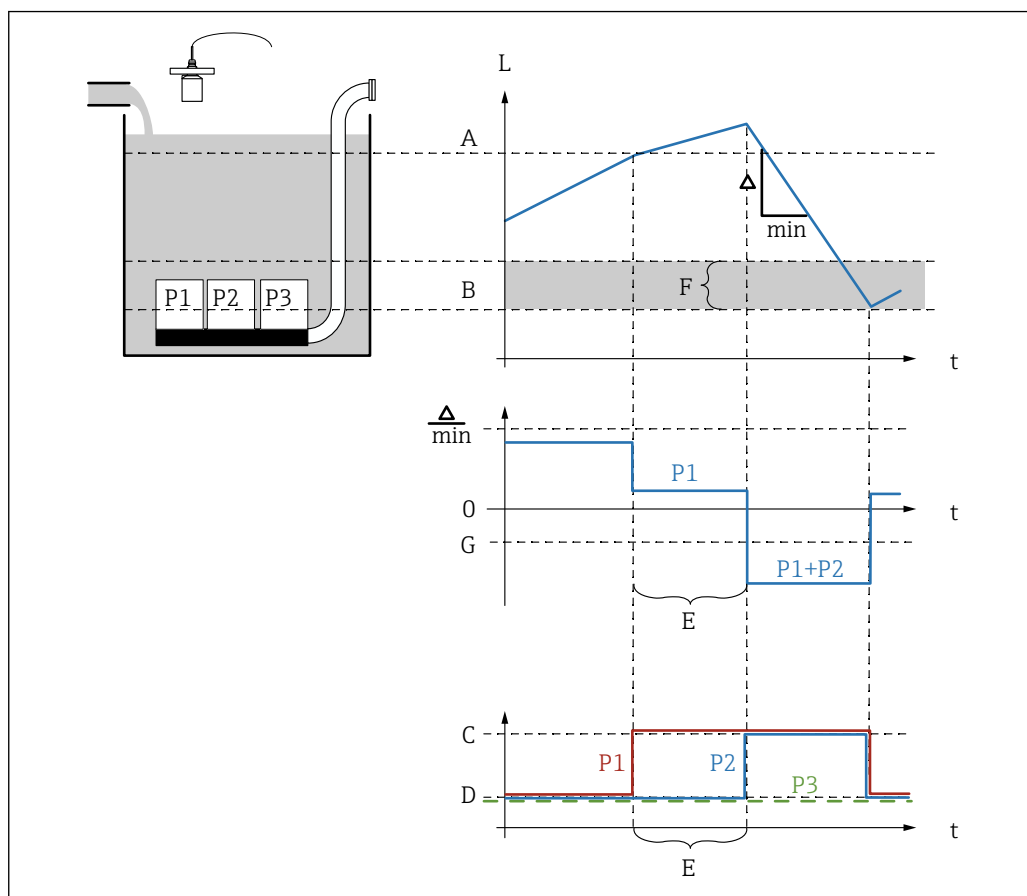
63 Principe de fonctionnement de la commande de vitesse de pompe
