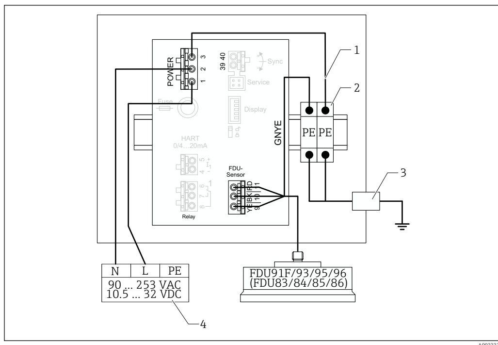
27 Compensation de potentiel de capteurs métalliques en boîtier de terrain en aluminium
