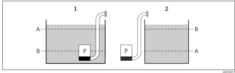
57 Point d'enclenchement et point de déclenchement pour la commande de limite
