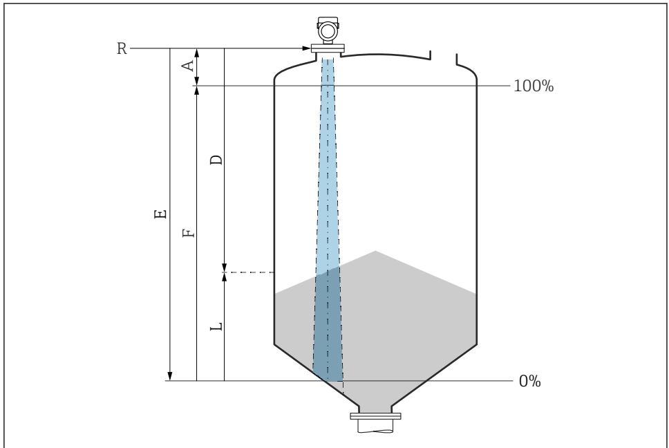
図 19 粉体のレベル測定用パラメータの設定
