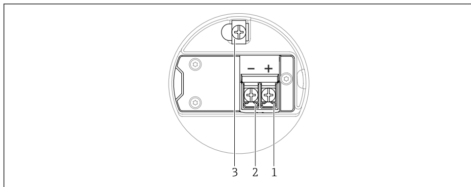
図 9 端子部の端子の割当て；4～20 mA HART；デュアルコンパートメントハウジング
