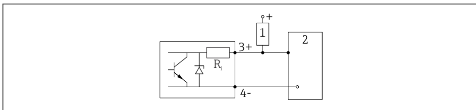
6 Tilslutningseksempel for den digitale indgang
