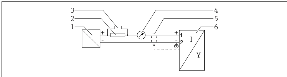
Funktionsdiagramm for 4 til 20 mA HART
