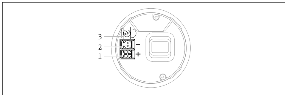
17 Aansluitklemmen en aardklem in het aansluitcompartiment, eenkamerbehuizing
