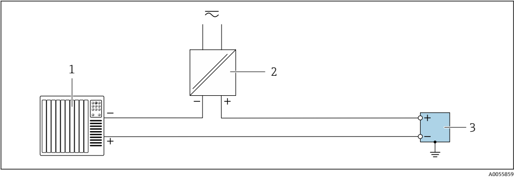
23 接线实例：继电器输出
