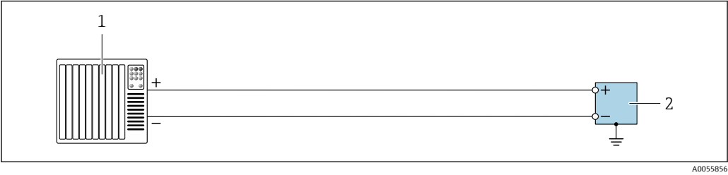
21 接线实例：脉冲输出/频率输出/开关量输出（有源）
