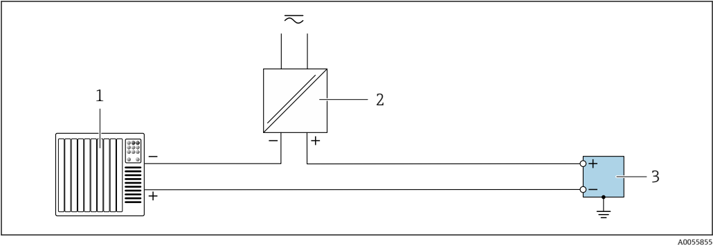
22 接线实例：脉冲输出/频率输出/开关量输出（无源）
