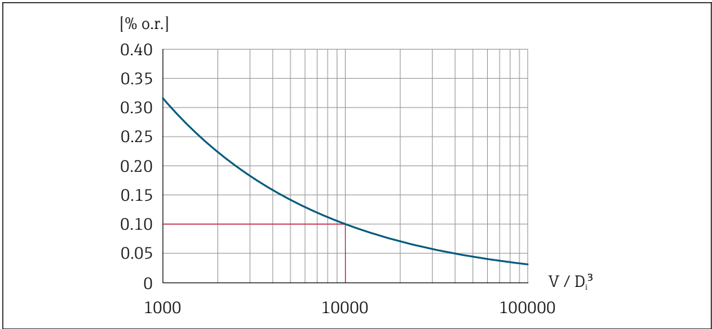
图 27 重复性 = 0.1 % o.r., 体积流量测量值[m³] of V = 10\,000 \cdot D_i^3
