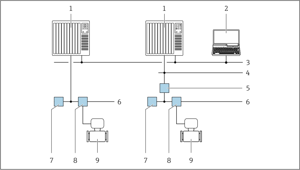
17 通过 FOUNDATION Fieldbus 网络进行远程操作
