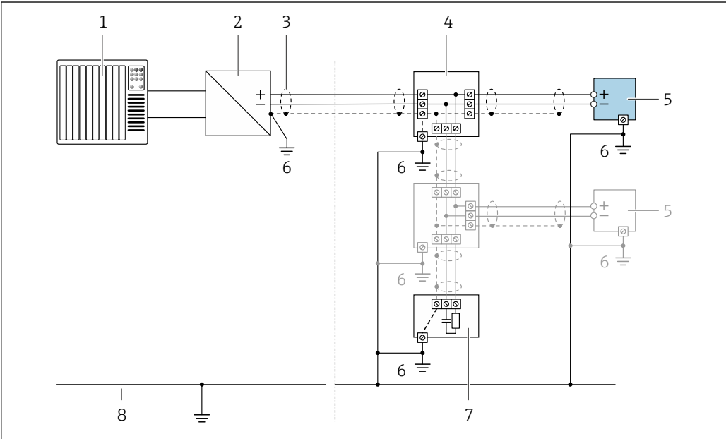
图 10 接线实例：FOUNDATION Fieldbus 1 自动化系统（例如 PLC） 2 电源调节器（FOUNDATION Fieldbus） 3 电缆屏蔽层：电缆屏蔽层必须两端接地，以符合 EMC 要求；请遵循电缆规格 4 接线箱 5 测量仪表 6 现场接地端 7 总线端接器 8 等电势连接线
