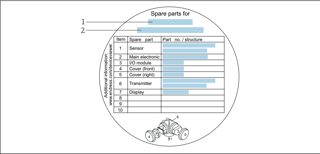
图 26 接线腔盖中的“备件标签”示例
