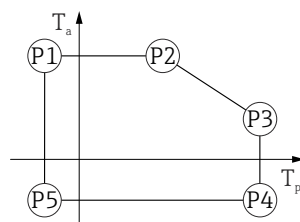
图 31 铝外壳, 带涂层; 过程温度范围: -20 \dots +200\text{ }^{\circ}\text{C} ( -4 \dots +392\text{ }^{\circ}\text{F} )
