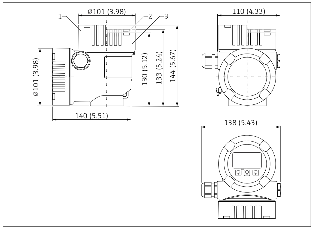
图 56 L 型双腔室铝外壳（带涂层）的外形尺寸示意图；包括 M20 接头和塑料插头。测量单位 mm (in)
