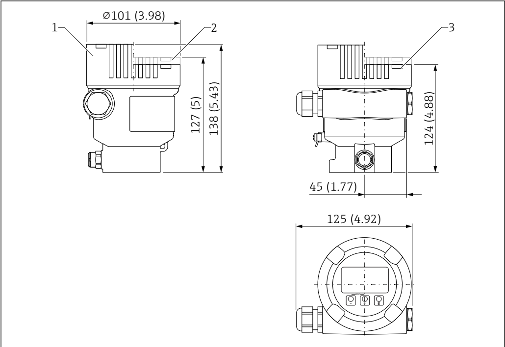
53 单腔室铝外壳（带涂层）的外形尺寸示意图；包括 M20 接头和塑料插头。测量单位 mm (in)
