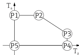
图 27 塑料外壳; 过程温度: 0 \dots +150 \text{ }^{\circ}\text{C} ( +32 \dots +302 \text{ }^{\circ}\text{F} ), 针对 CSA C/US 认证型仪表
