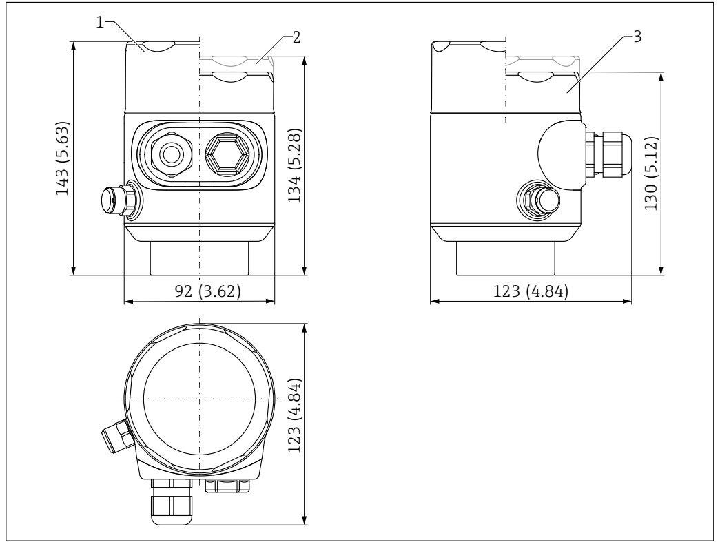
图 54 316L 单腔室外壳（卫生型）的外形尺寸示意图；包括 M20 接头和塑料插头。测量单位 mm (in)
