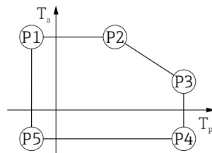
图 49 316L 外壳，卫生型；过程温度范围：-40 ... +200 °C (-40 ... +392 °F)
