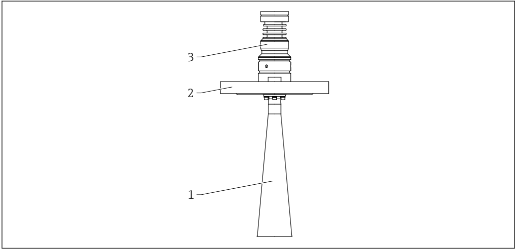
图 62 DN65 喇叭天线的材质。测量单位 mm (in)
