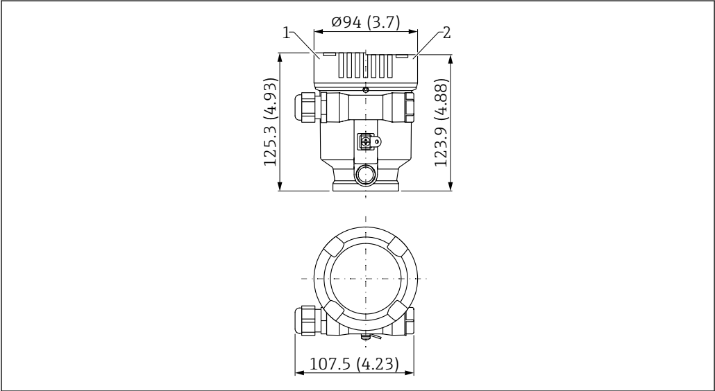
52 单腔室塑料外壳的外形尺寸示意图；包括 M20 接头和塑料插头。测量单位 mm (in)
