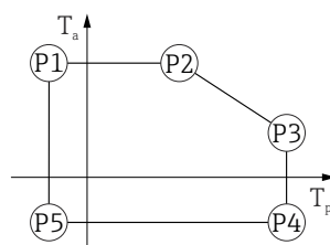
图 46 316L 外壳, 卫生型; 过程温度范围: -20 ... +150 °C (-4 ... +302 °F)
