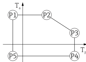
图 48 316L 外壳，卫生型；过程温度范围：-40 ... +150 °C (-40 ... +302 °F)
