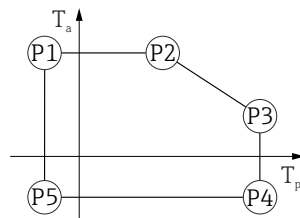
图 30 铝外壳, 带涂层; 过程温度范围: -20 \dots +150\text{ }^{\circ}\text{C} ( -4 \dots +302\text{ }^{\circ}\text{F} )
