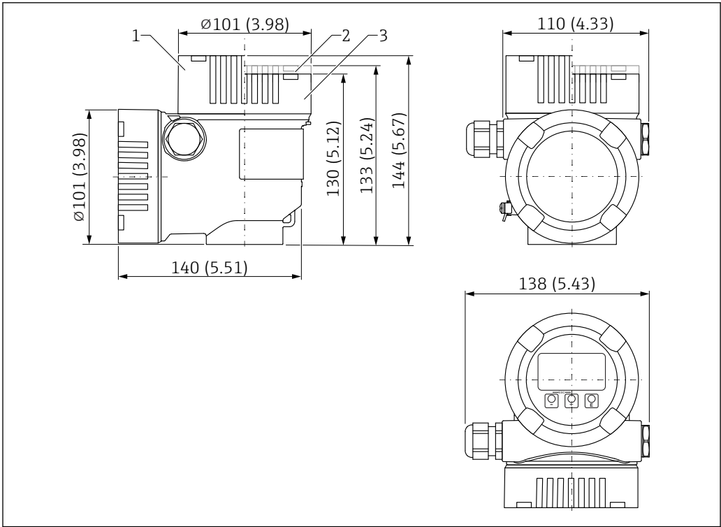
图 57 L 型双腔室 316L 外壳的外形尺寸示意图；包括 M20 接头和塑料插头。测量单位 mm (in)
