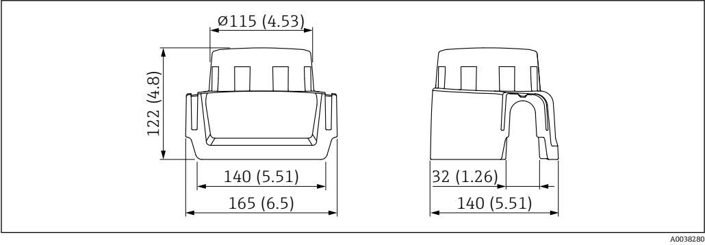
图 69 塑料防护罩 XW111 的外形尺寸示意图。测量单位 mm (in)
