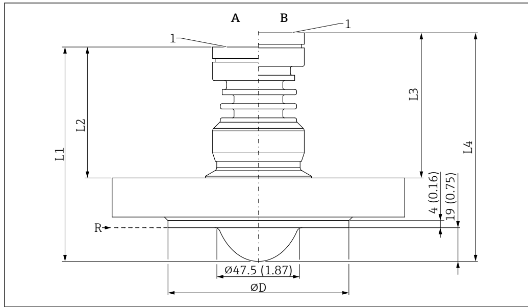
图 60 PTFE 涂层天线（齐平安装，50 mm (2 in)口径）的外形尺寸示意图；带法兰。测量单位 mm (in)
