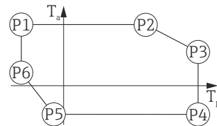
图 51 316L 外壳，卫生型；过程温度：-196 ... +200 °C (-320 ... +392 °F)
