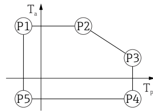
图 50 316L 外壳，卫生型；过程温度：-60 ... +150 °C (-76 ... +302 °F)
