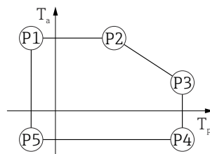
图 22 塑料外壳; 过程温度: -40 \dots +280 \text{ }^{\circ}\text{C} ( -40 \dots +536 \text{ }^{\circ}\text{F} )
