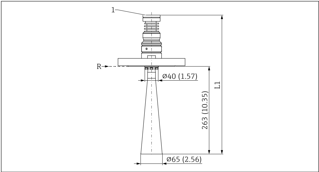
图 58 DN65 喇叭天线的外形尺寸示意图；法兰过程连接。测量单位 mm (in)
