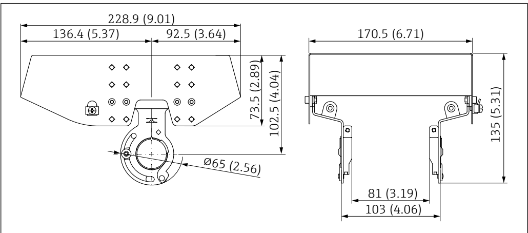
图 68 316L 防护罩 XW112 的外形尺寸示意图。测量单位 mm (in)
