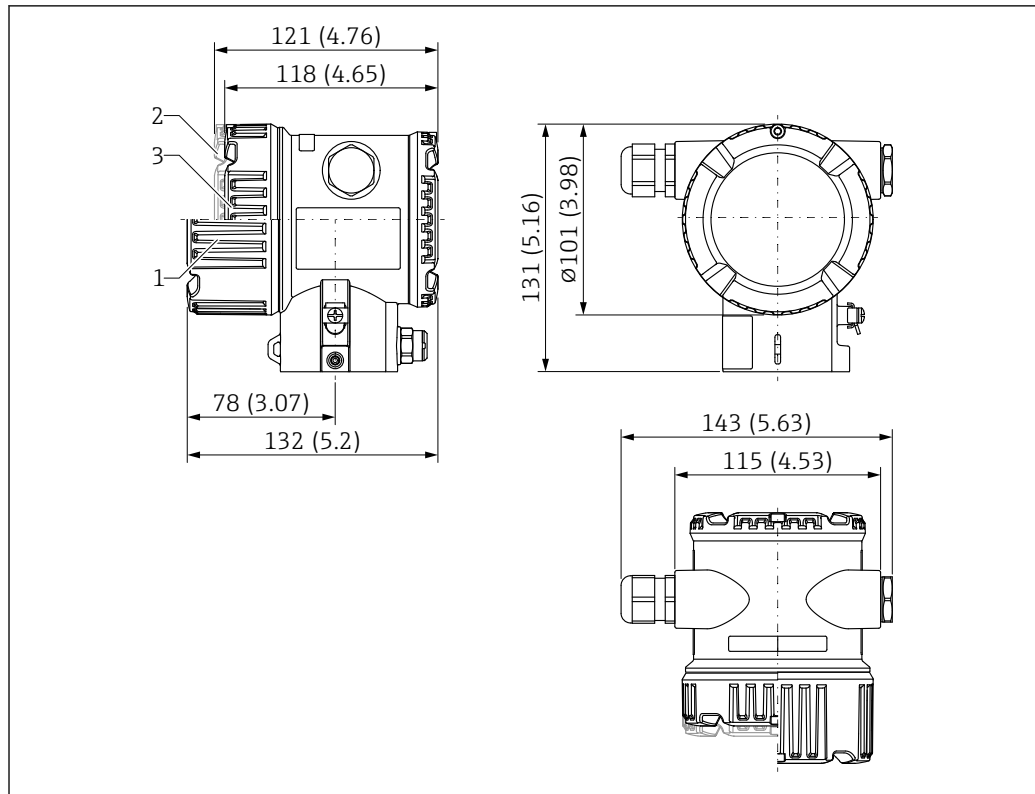
图 55 双腔室铝外壳（带涂层）的外形尺寸示意图；包括 M20 接头和塑料插头。测量单位 mm (in)
