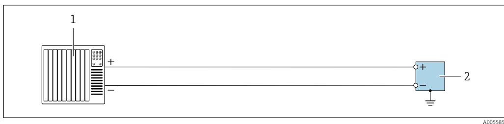
17 Пример подключения для импульсного/частотного/релейного выхода (активного)
