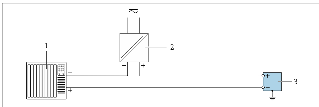
19 Пример подключения для релейного выхода
