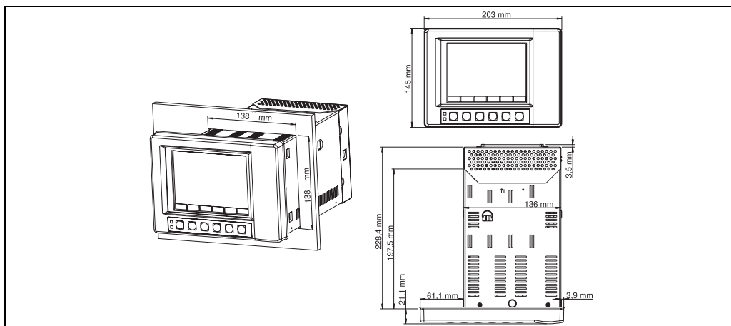
Abb. 2: Schalttafeleinbau bei Version mit Druckguss- bzw. Edelstahlfront
