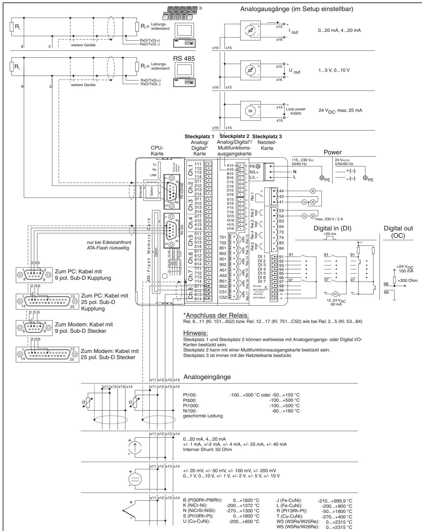
Abb. 3: Anschlüsse/Klemmenplan:
