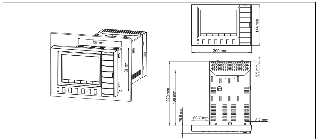
Abb. 10: Abmessungen Schalttafeleinbau bei Version mit Metall-Druckgussfront
