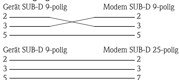
Abb. 7: Kabelbelegung Modem
