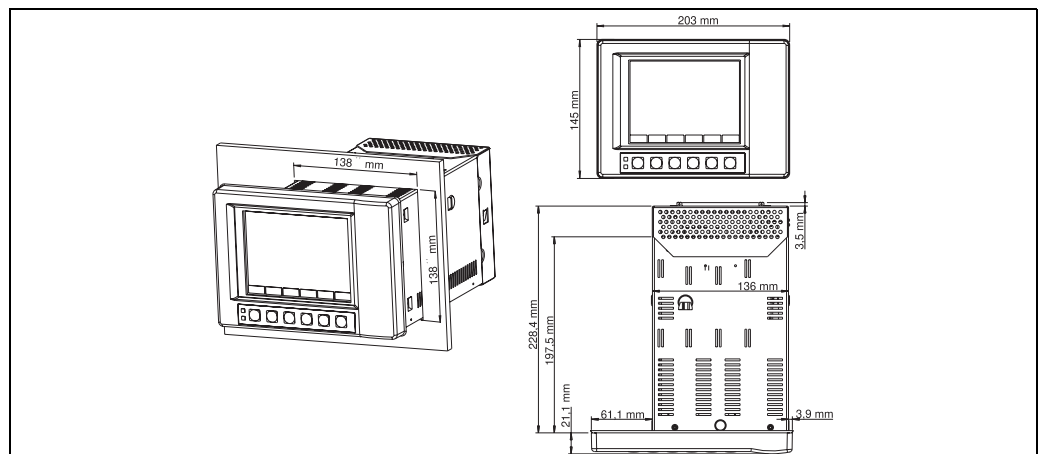
Abb. 11: Abmessungen Schalttafeleinbau bei Version mit Edelstahlfront
