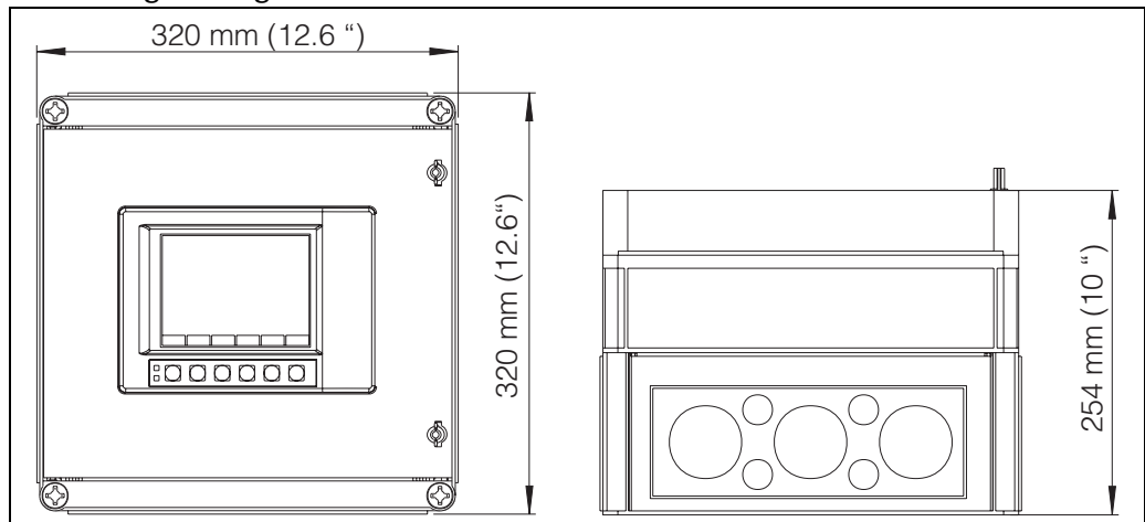
Abb. 14: Abmessungen Feldgehäuse (Angaben in mm)
