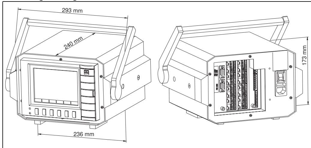
Abb. 13: Abmessungen Tischgehäuse (Angaben in mm)
