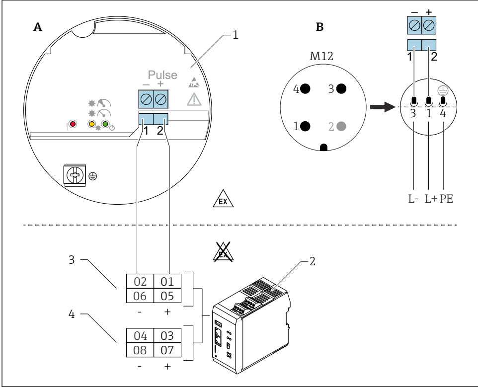
19 Bağlantı şeması: FEL60D elektronik parça ünitesinin QML51 Yoğunluk Hesaplayıcısına bağlantısı
