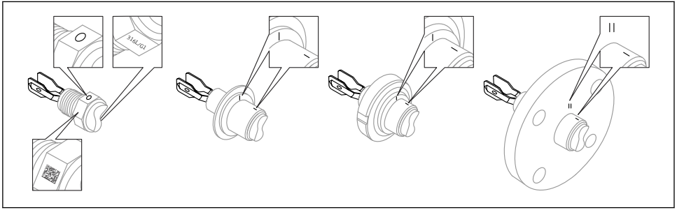
13 İşaretleme kullanılarak kanala yatay olarak monte edildiğinde titreşim çatalının konumu
