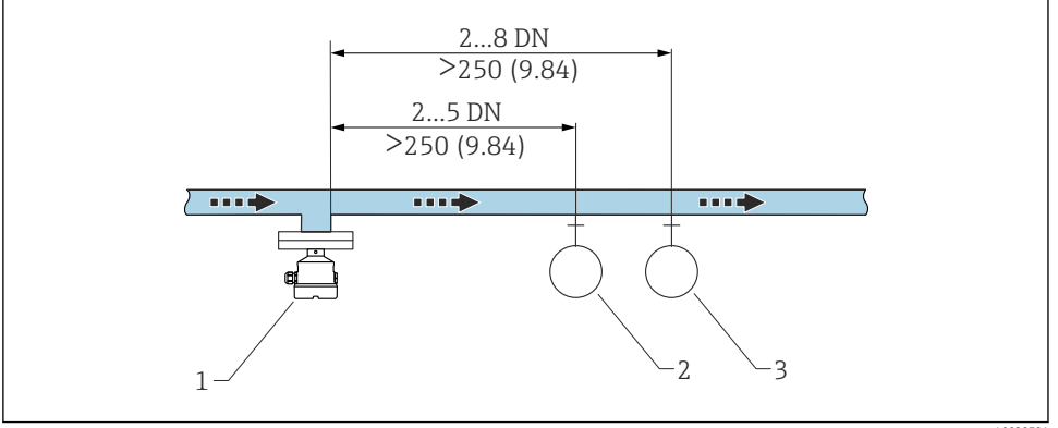
9 Çıkış yolunun montajı. Ölçü birimi mm (in)
