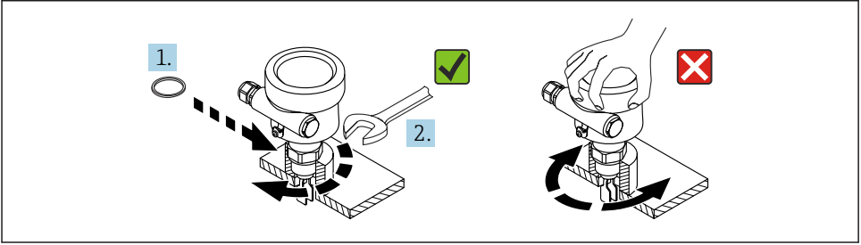
15 Cihazın vidalanması
