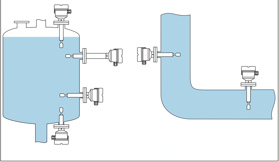
4 Bir kanal, tank veya boru için kurulum örnekleri
