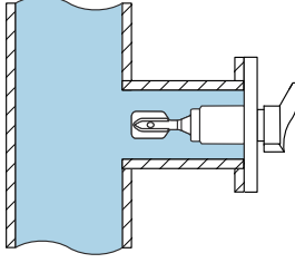
7 Doğrudan ürün akışından uzaktaki borulara montaj örneği
