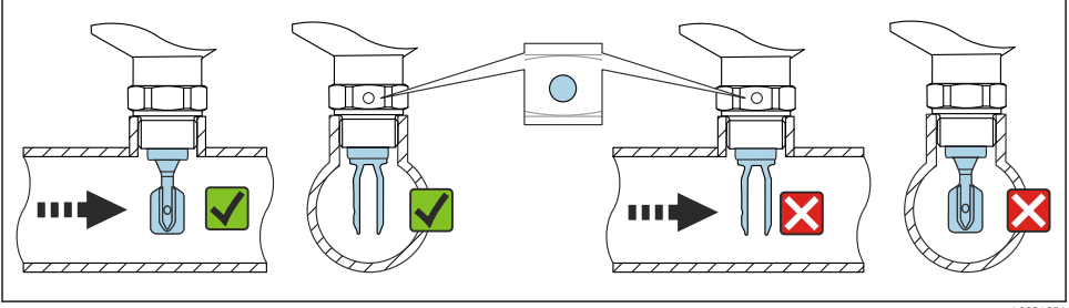
14 Boru tesisatına montaj (çatal pozisyonunu ve işareti dikkate alın)
