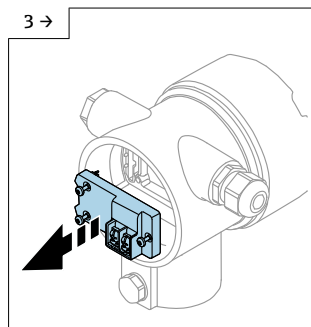
► 2-Draht Klemmenmodul
