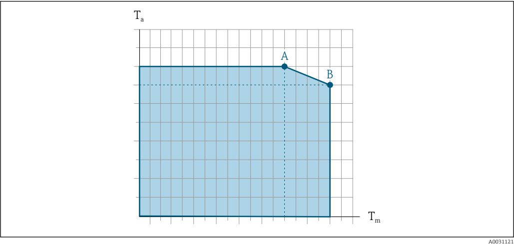
36 Пример зависимости, значения приведены в таблице. T a Температура окружающей среды T m Температура технологической среды A Максимально допустимая температура среды T m при T a max = 60 °C (140 °F); более высокие значения температуры технологической среды T m требуют снижения температуры окружающей среды T a B Максимально допустимая температура окружающей среды T a при максимальной установленной температуре среды T m для сенсора
