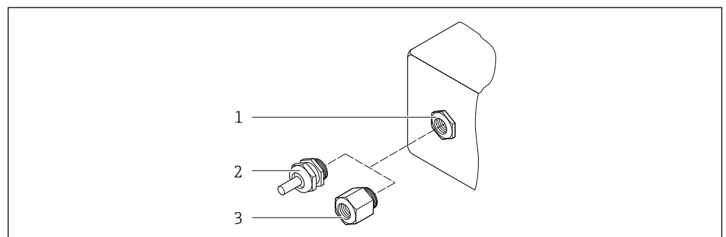
37 Возможные варианты кабельных вводов / кабельных уплотнений
