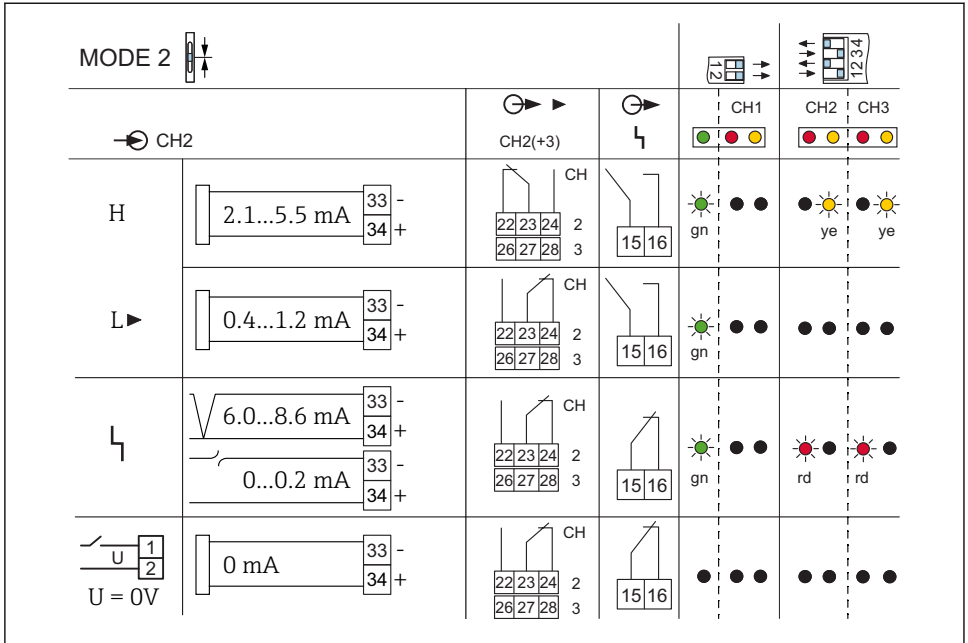
17 Comportamiento de la conmutación y señalización con corriente de error L < 1,2 \text{ mA} (FEL48, FEL58, FEL68, FEM58, FEI58)
