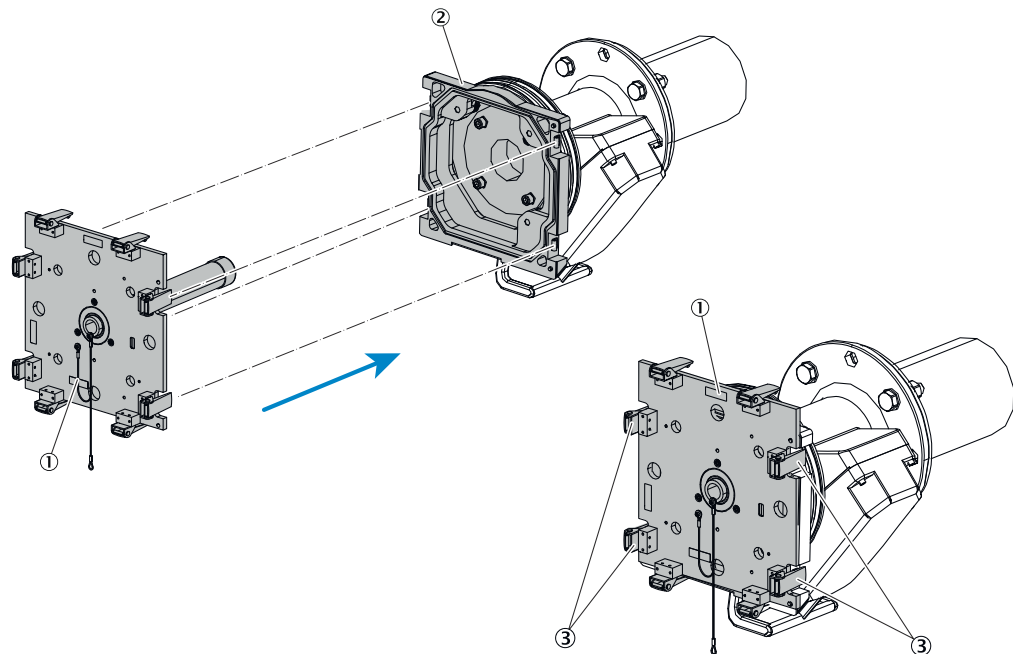
Abbildung 21: Anbau Justiervorrichtung Empfangseinheit
