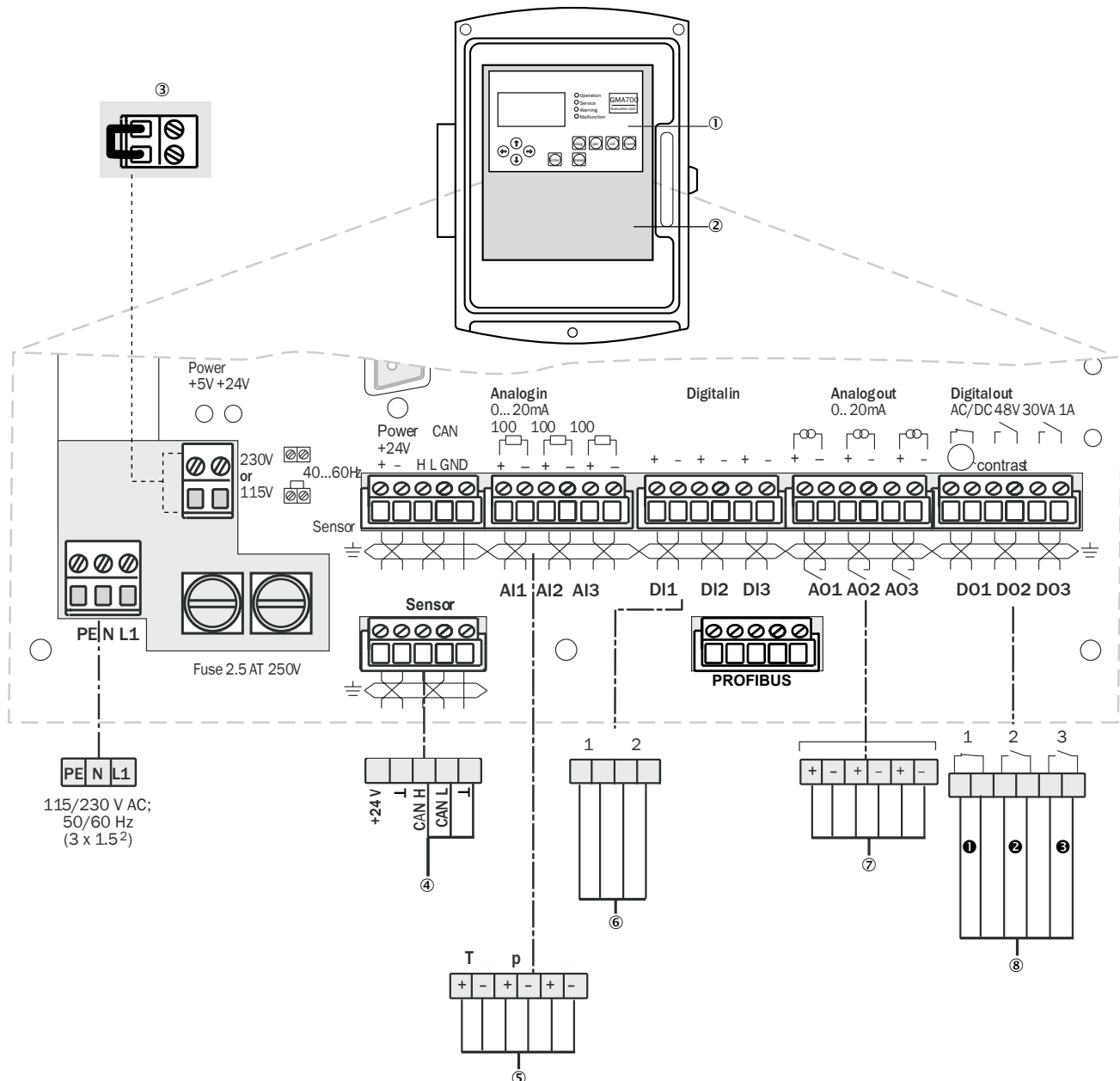
Abbildung 14: Elektrische Verdrahtung der Steuereinheit AWE
