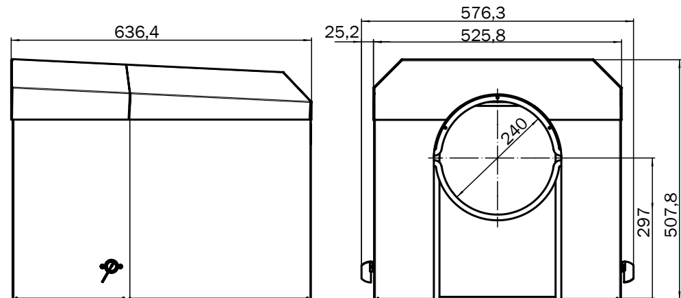
Abbildung 42: Wetterschutzhaube für Sende-Empfangseinheit (Maße in mm)
