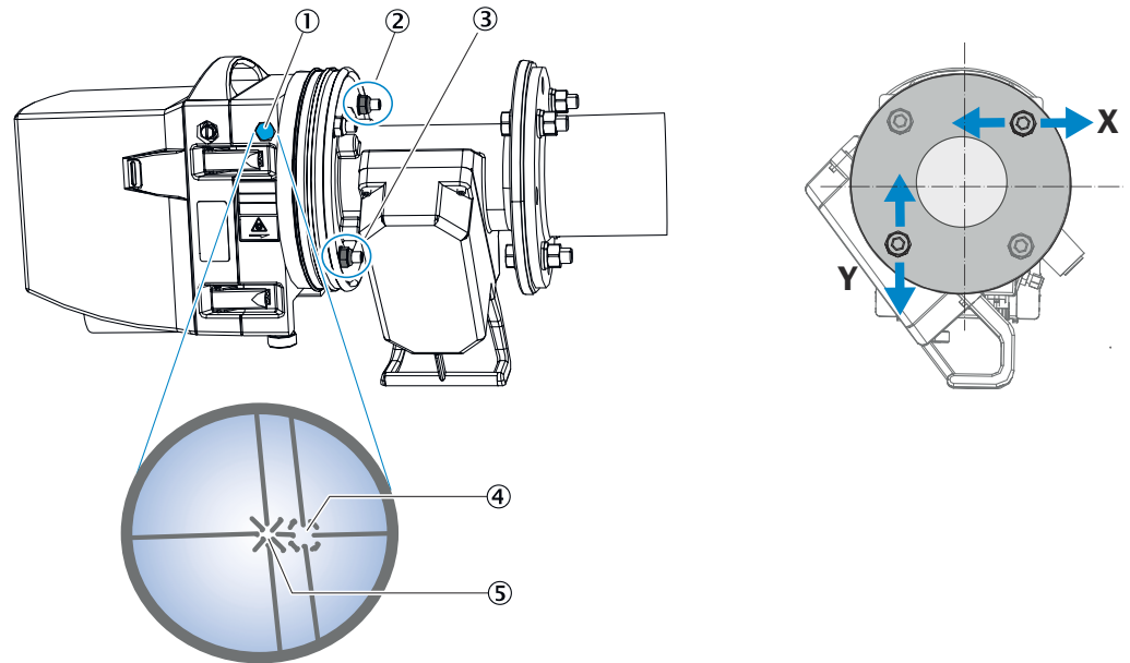
Abbildung 27: Optische Feinausrichtung an Sende-Empfangseinheit (NH 3 , HF)
