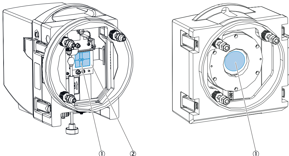
Abbildung 34: Optische Oberflächen an der Sende-Empfangseinheit und Reflektoreinheit
