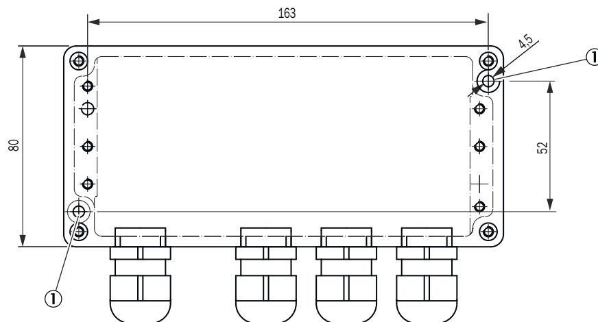
Abbildung 11: Montage Anschlusseinheit (Maße in mm)
