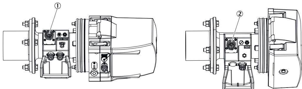
Abbildung 16: Spülluftanschlüsse an Sende-Empfangseinheit und Reflektoreinheit
