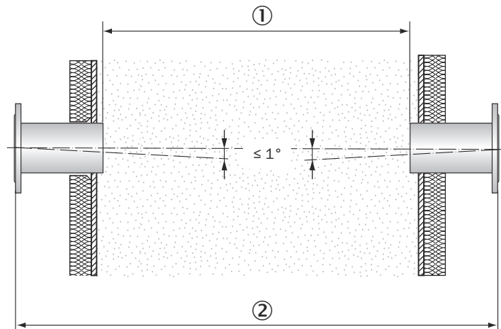
Abbildung 3: Flansche mit Rohr – Festlegung Messstrecke
