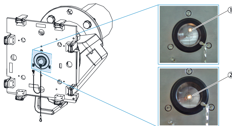
Abbildung 23: Überprüfung optische Ausrichtung Reflektoreinheit
