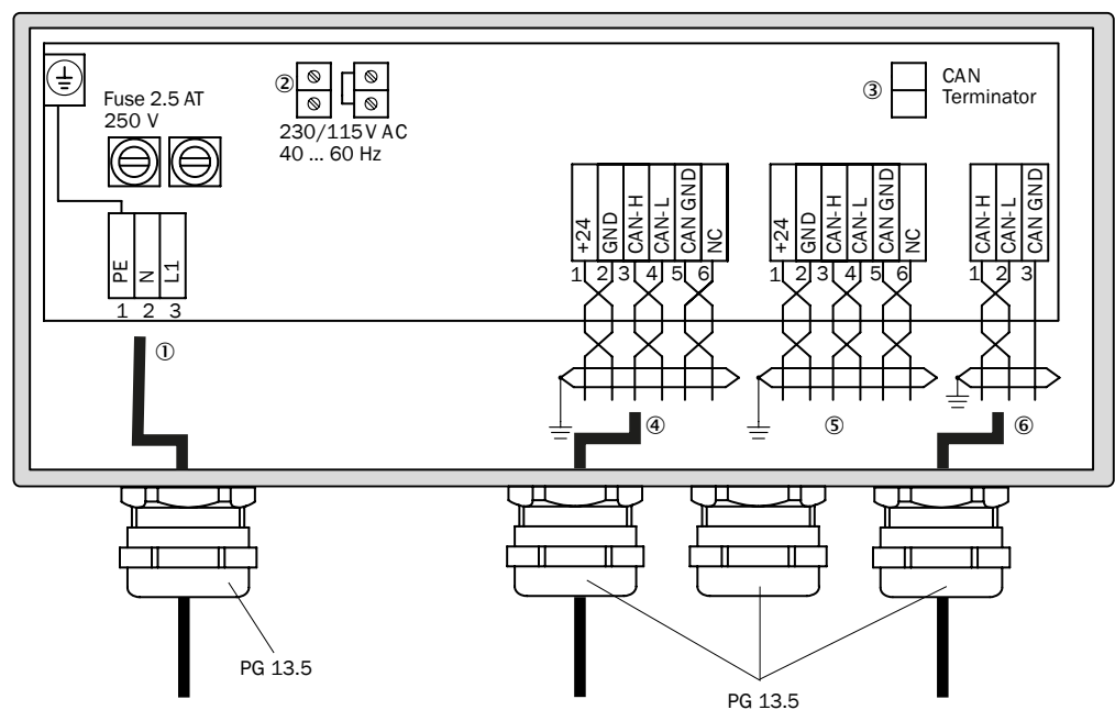
Abbildung 17: Elektrischer Anschluss Anschlusseinheit
