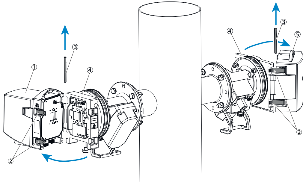
Abbildung 33: Demontage Sende-Empfangseinheit und Reflektoreinheit
