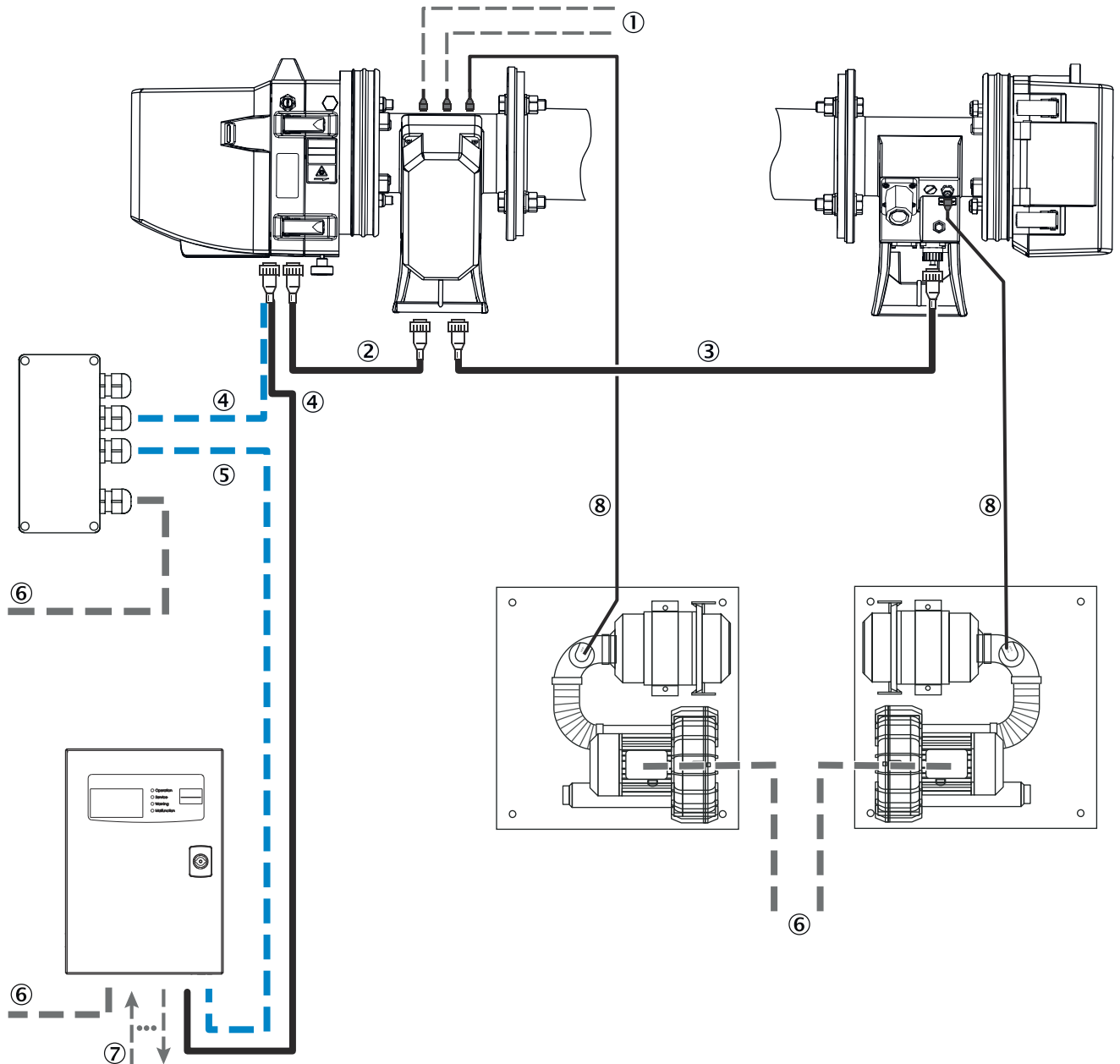
Abbildung 12: Elektrische Verdrahtung der Gerätekomponenten
