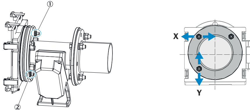
Abbildung 22: Optische Ausrichtung Reflektoreinheit
