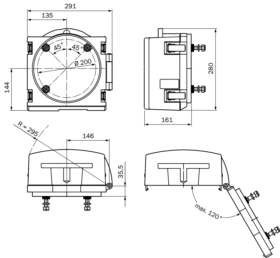
Abbildung 37: Reflektoreinheit (Maße in mm)
