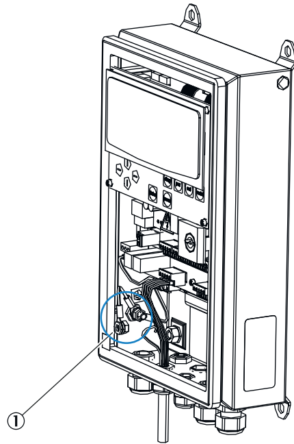
Abbildung 15: Anschluss der Erdungsleitungen
