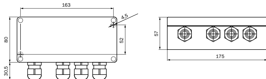
Abbildung 41: Abmessungen Anschlusseinheit (Maße in mm)
