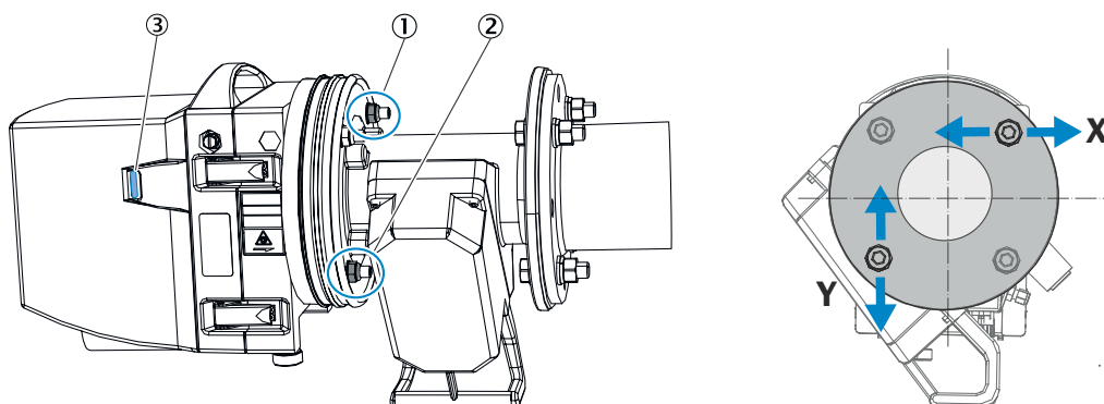
Abbildung 28: Optische Feinausrichtung an Sende-Empfangseinheit (HCl, CO)
