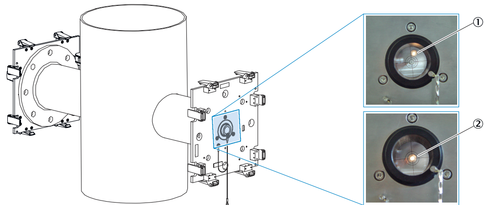
Abbildung 6: Überprüfung der Ausrichtung
