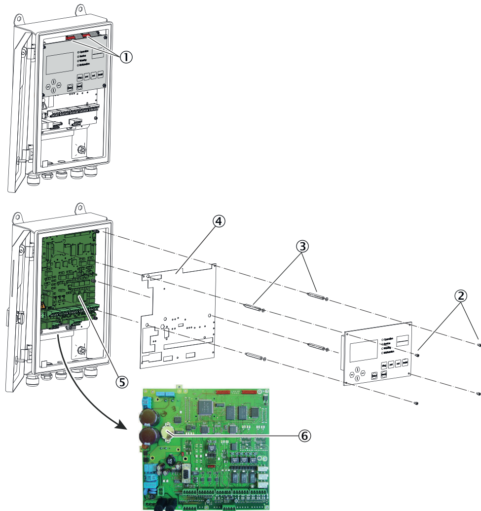
Abbildung 35: Steuereinheit demontieren
