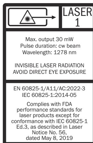
Laserschild: HF-Messung
