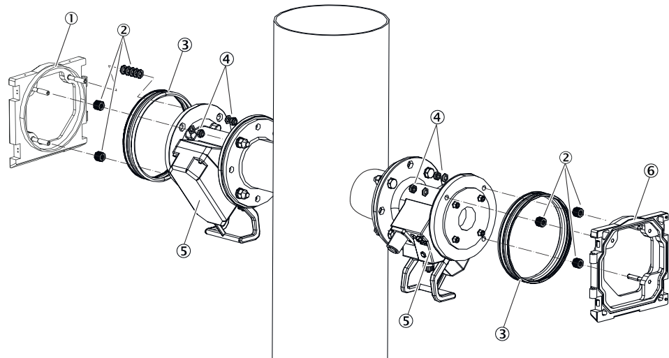
Abbildung 8: Montage der Flanschvorsätze
