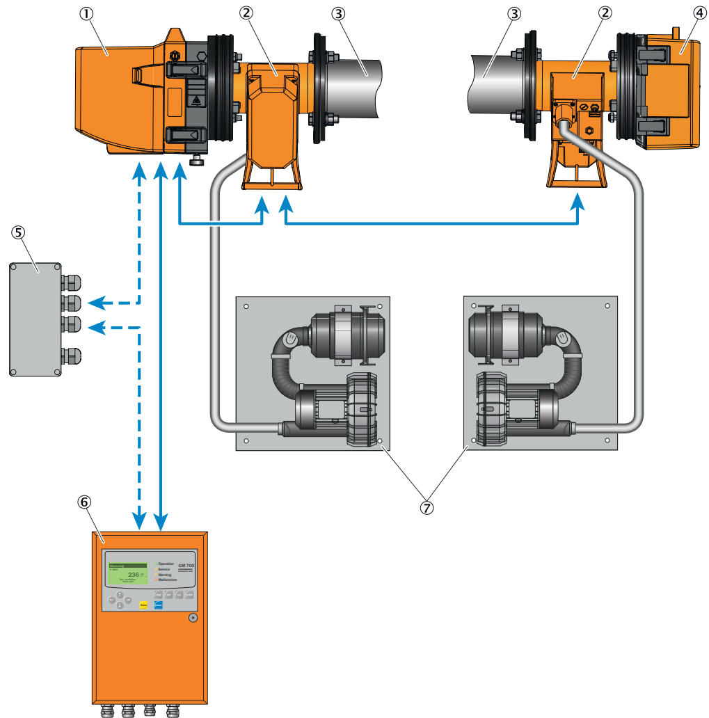
Abbildung 2: Aufbau der Messgerätekomponenten
