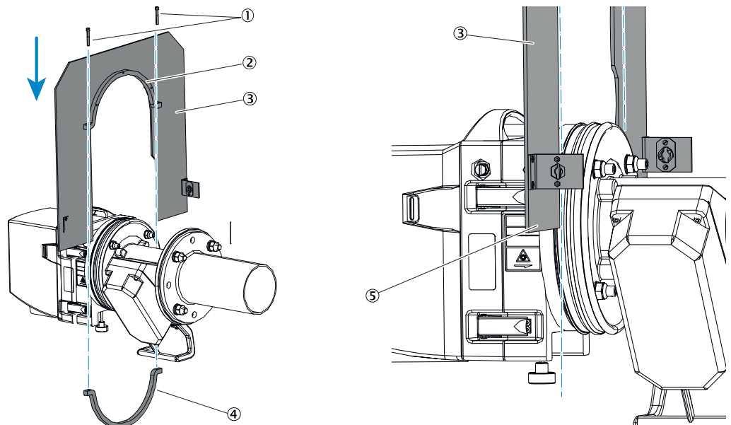
Abbildung 30: Montageplatte anbauen.
