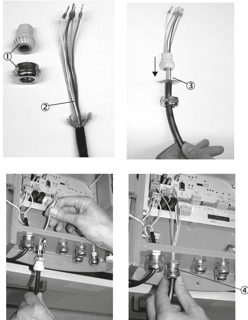
Abbildung 13: CAN-Bus-Leitung korrekt montieren (dargestellt an der Steuereinheit AWE)
