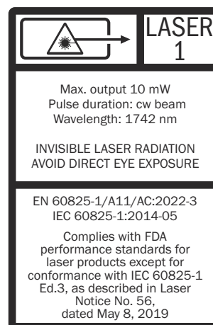
Laserschild: HCl-Messung
