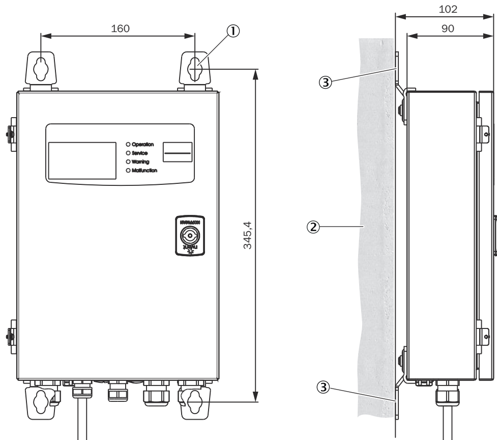
Abbildung 10: Montage Steuereinheit AWE Stahlblechgehäuse (Maße in mm)
