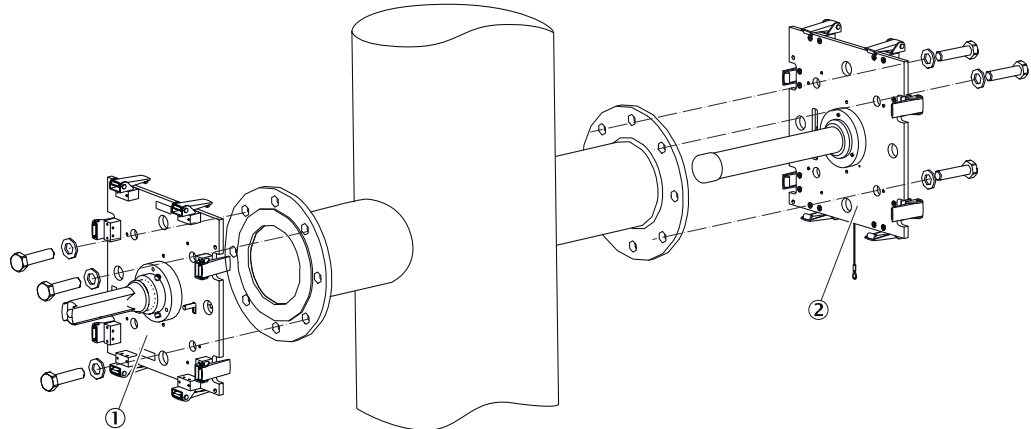
Abbildung 5: Justiervorrichtung anbringen
