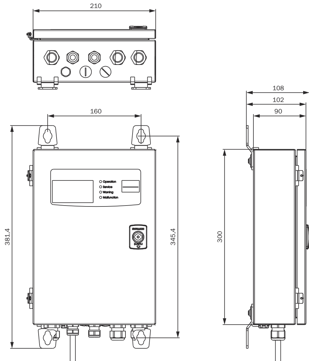
Steuereinheit AWE
