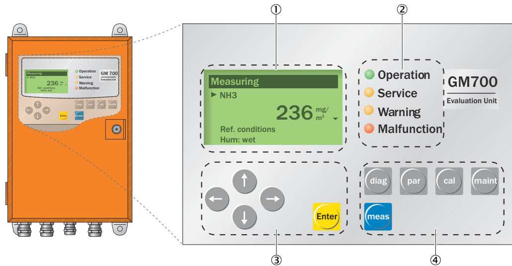
Abbildung 32: Bedien- und Anzeigeelemente
