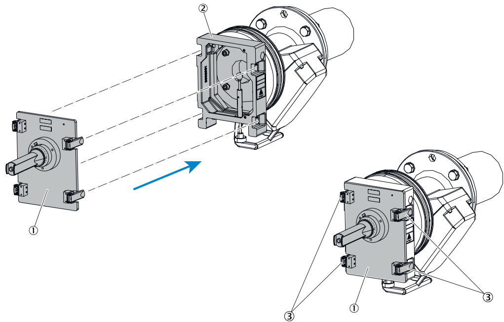
Abbildung 20: Anbau Justiervorrichtung Sendeeinheit
