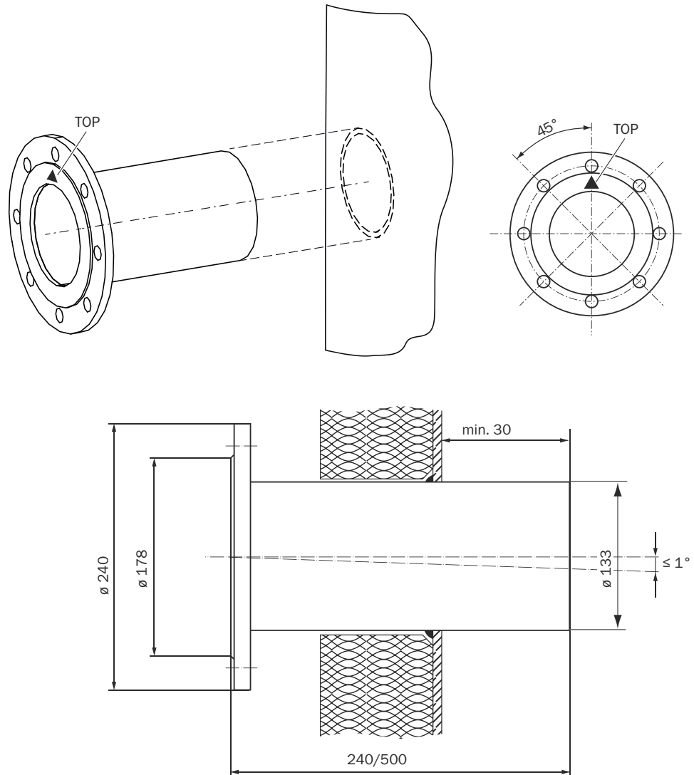
Abbildung 4: Flansch mit Rohr inkl. Orientierung "TOP"
