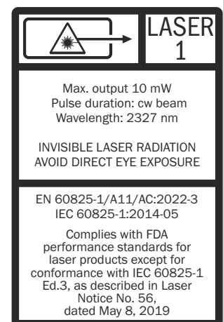
Laserschild: CO-Messung
