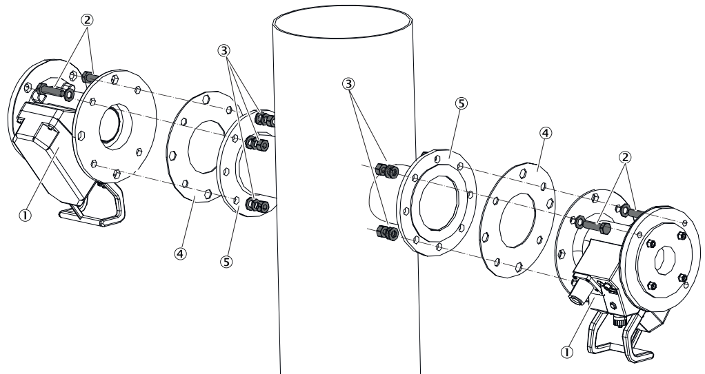
Abbildung 7: Montage der Spülluftvorsätze an Flansche mit Rohr
