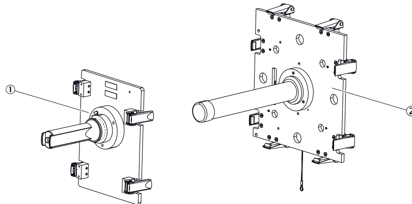
Abbildung 19: Justiervorrichtung
