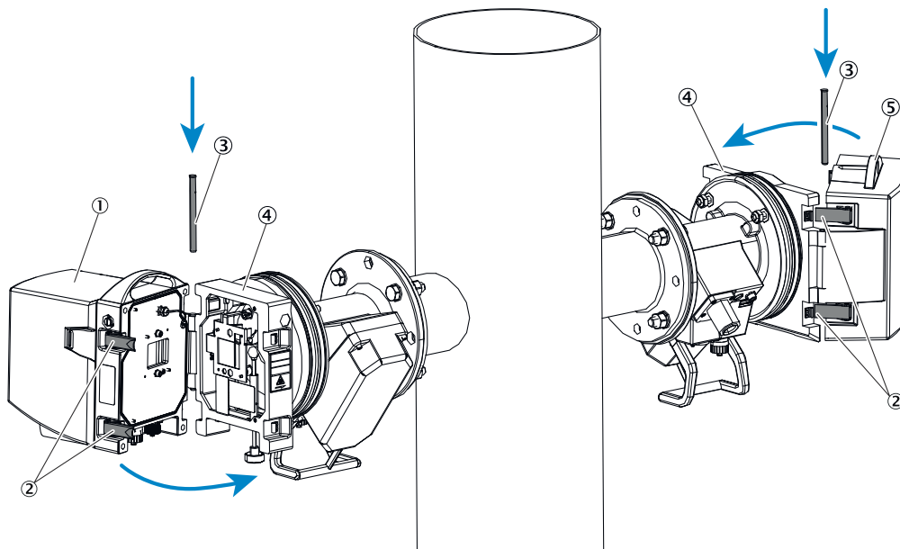
Abbildung 24: Sende-Empfangseinheit und Reflektoreinheit an Flanschvorsätze montieren
