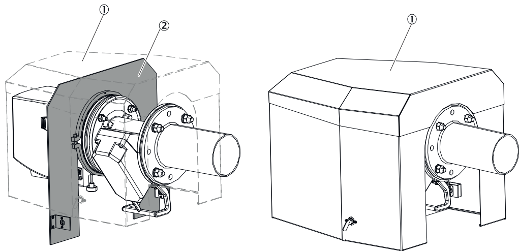
Abbildung 31: Wetterschutzhaube aufsetzen.
