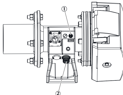
Abbildung 26: Elektrische Anschlüsse Reflektoreinheit
