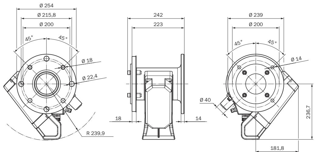
Abbildung 40: Spülluftvorsatz (Maße in mm)
