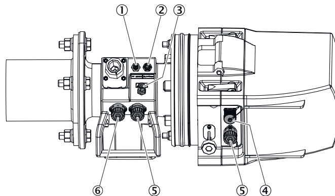
Abbildung 25: Elektrische Anschlüsse Sende-Empfangseinheit
