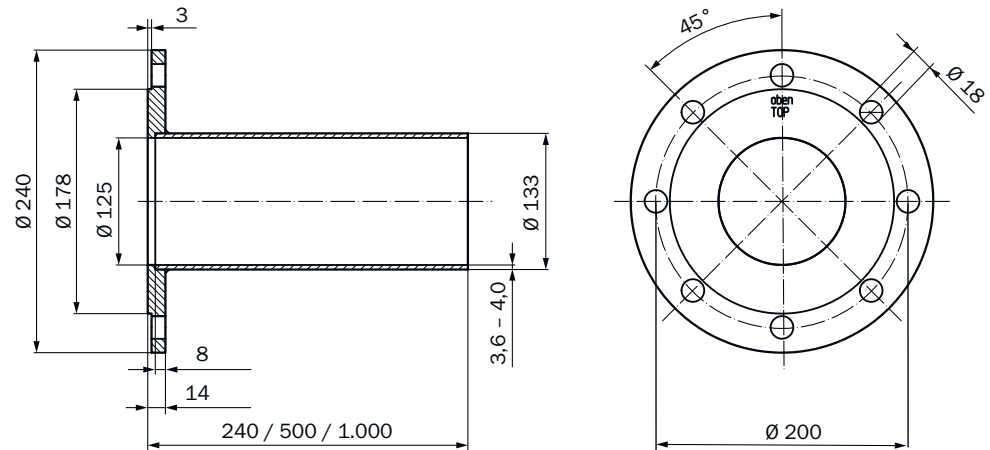
Abbildung 39: Flansch mit Rohr DN125 (Maße in mm)
