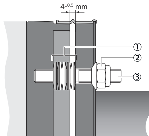
Abbildung 9: Detailansicht Anordnung der Tellerfedern
