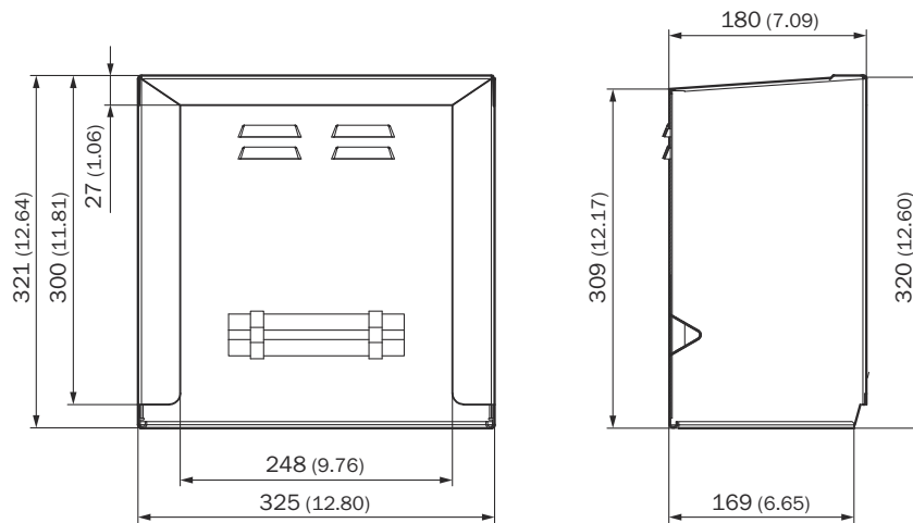
Abbildung 43: Wetterschutzhaube für Reflektoreinheit (Maße in mm)
