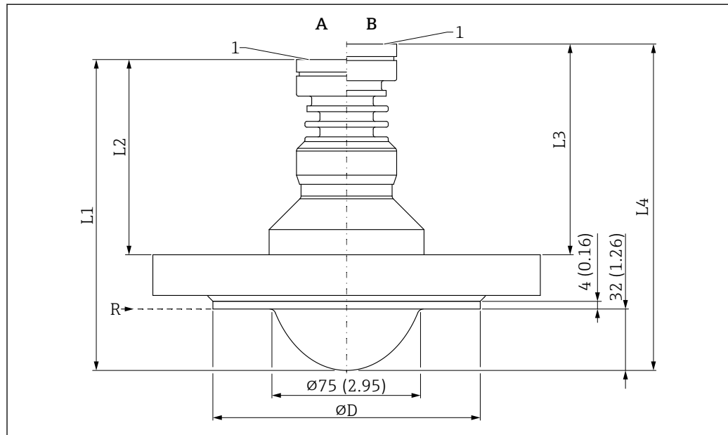
61 Размеры пластированной материалом PTFE антенны, монтируемой заподлицо, 80 мм (3 дюйм), с фланцем. Единица измерения мм (дюйм)
