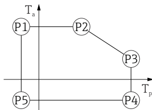
30 Алюминиевый корпус с покрытием; рабочая температура -20 до +150 °C ( -4 до +302 °F)
