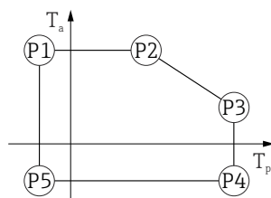
■ 16 Пластмассовый корпус; рабочая температура -20 до +200 °C ( -4 до +392 °F)
