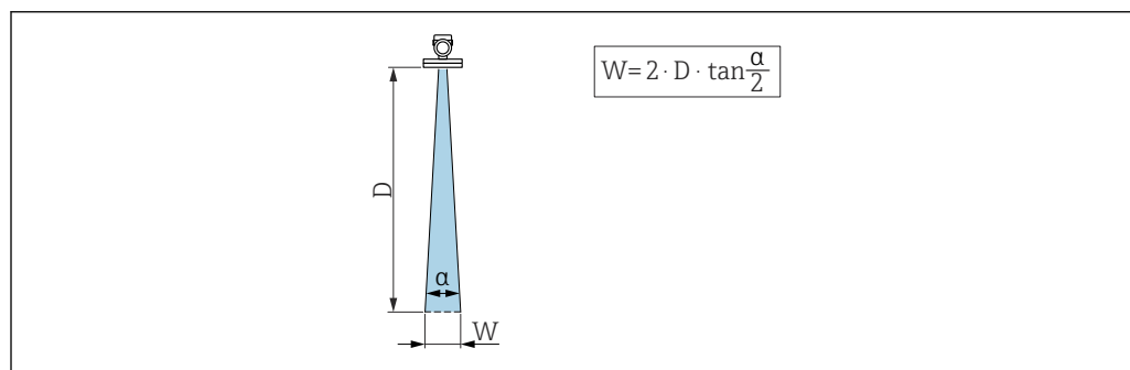
9 Взаимосвязь между углом расхождения луча \alpha , расстоянием D и диаметром луча W
