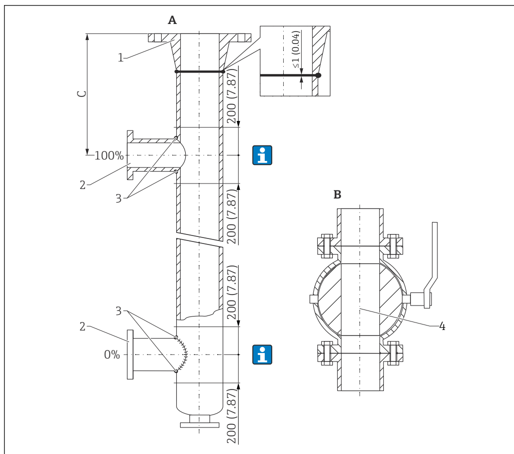
13 Пример конструкции байпаса. Единица измерения мм (дюйм)
