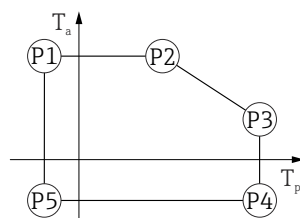
20 Пластмассовый корпус; рабочая температура -40 до +200 °C (-40 до +392 °F)
