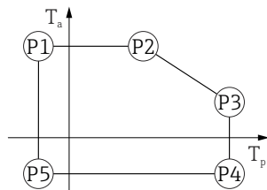
14 Пластмассовый корпус; рабочая температура -20 до +150 °C ( -4 до +302 °F)
