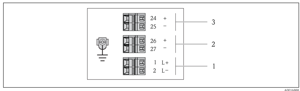
6 Przyporządkowanie zacisków dla wersji 4-20 mA HART z wyjściem impulsowym/częstotliwościowym/statusu
