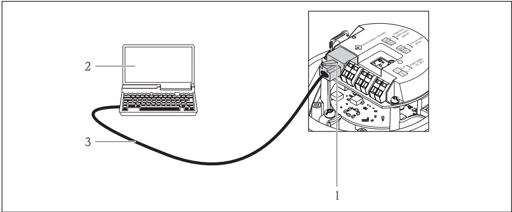
15 Sposób podłączenia dla pozycji kodu zam. "Wyjście; wejście", opcja B: "4-20mA HART, imp./częst./wyj. statusu"
